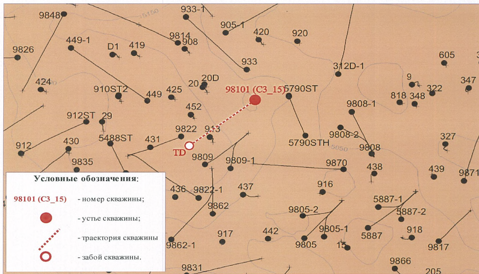
Рис. 4.2 Структурная карта по кровле II объекта
