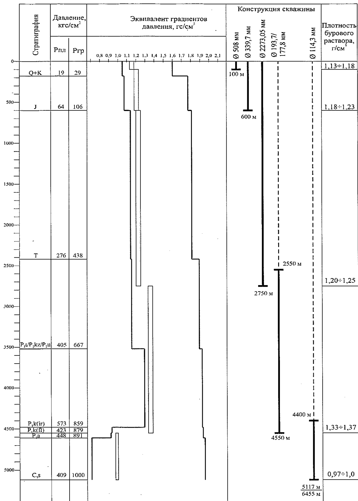
Рисунок 5.1_2- Совмещенный график давлений (облечённая конструкция)
