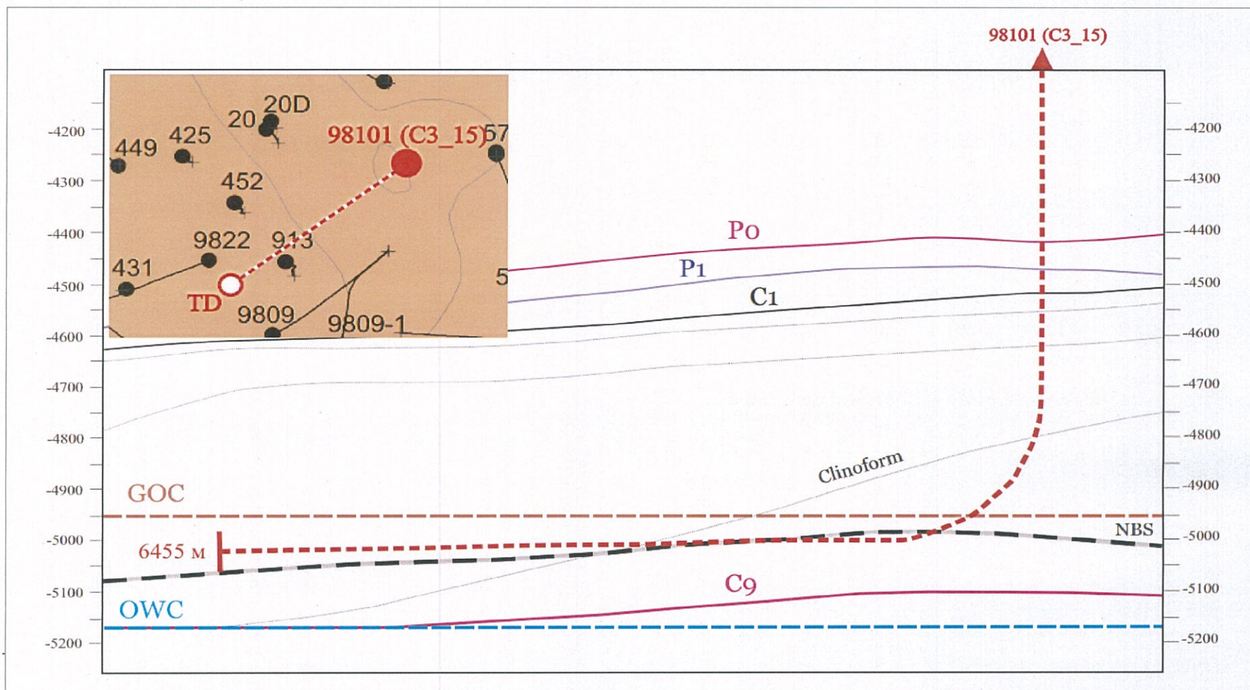
Рис. 4.1 - Профиль скважины
