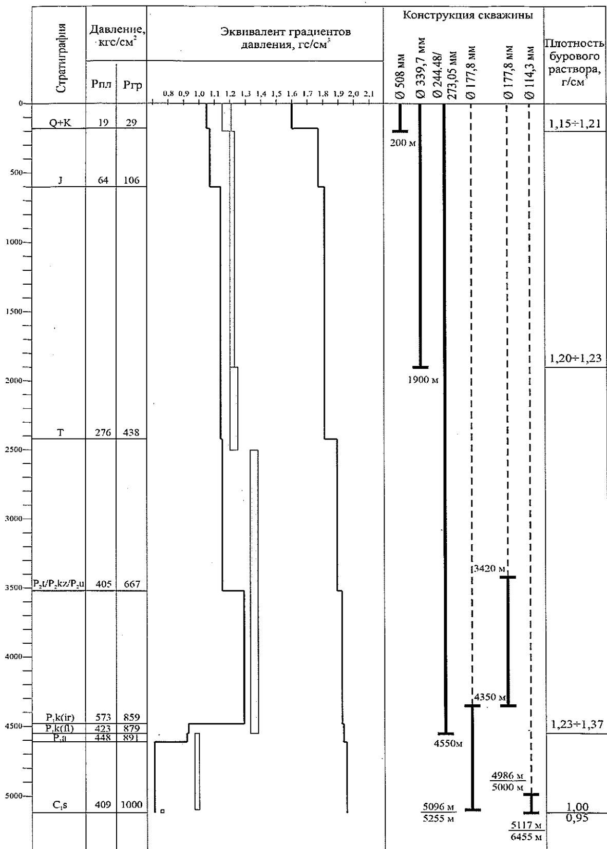
Рисунок 5.1_1- Совмещенный график давлений (стандартная конструкция)
