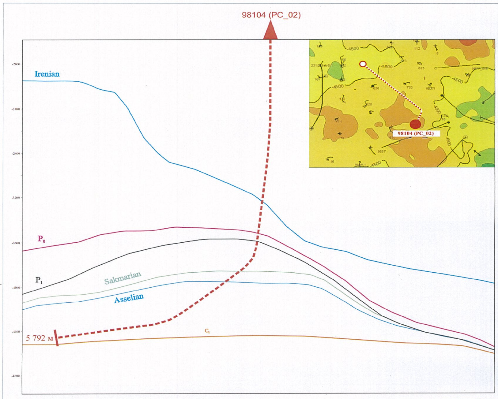
Рис. 4.1 - Профиль скважины
