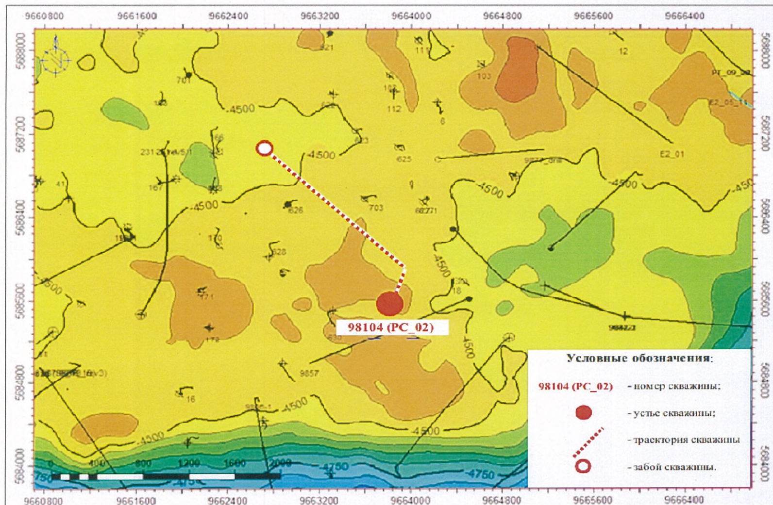
Рис. 4.2 Структурная карта по кровле I объекта
