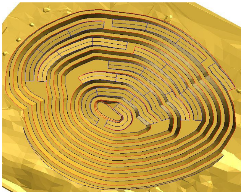
Рис. 5. План карьера месторождения Коктас
