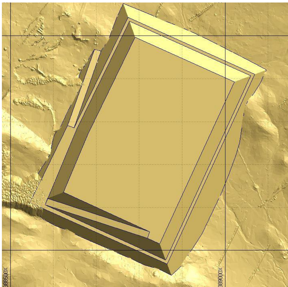
Рис. 9. Аксонометрия отвала
