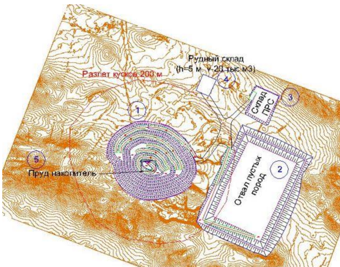
Рис. 10. Генплан месторождения Коктас
