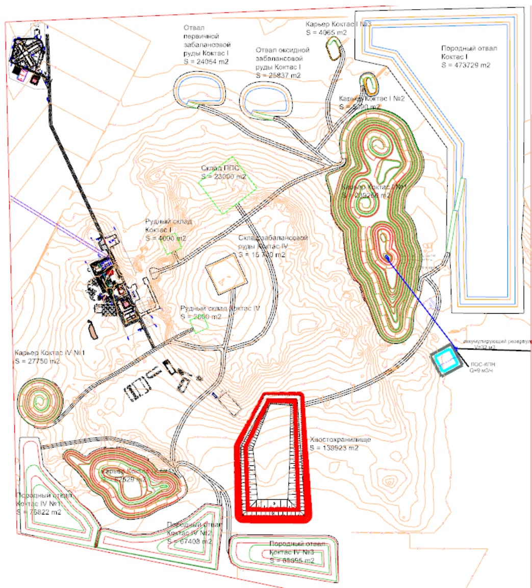
Генеральный план месторождения Коктас
