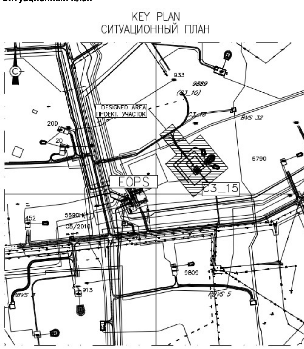
Рисунок 2.1. Ситуационный план
