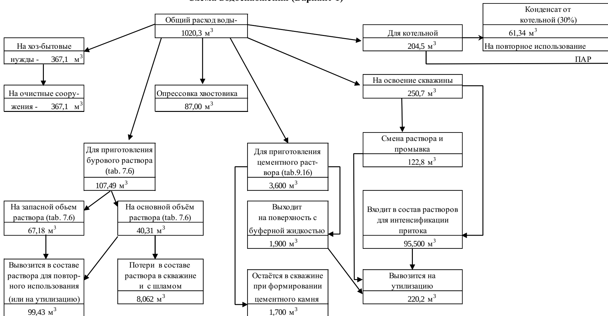
Рисунок 3.5 – Схема водопотребления и водоотведения при бурении горизонтального бокового ствола 239-1 в скважине 239 вариант 1
