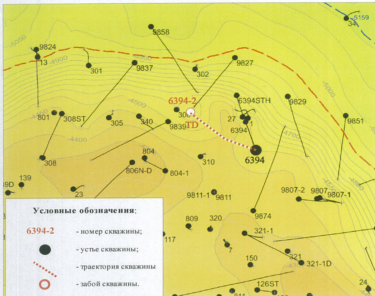
Рисунок 4.2 - Структурная карта по кровле С 1
