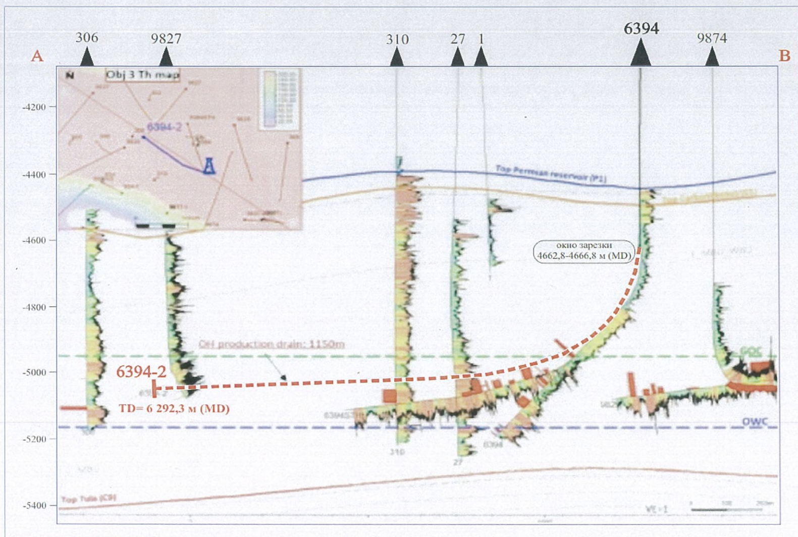
Рисунок 4.1 - Профиль скважины
