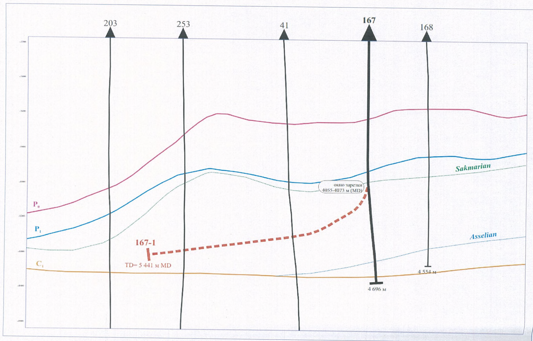
Рис.4.1 - Профиль скважины
