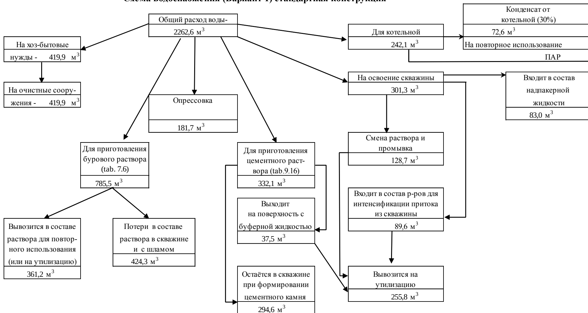
Рисунок 3.5 – Схема водопотребления и водоотведения при строительстве скважины 98103 (C2_13) вариант 1
