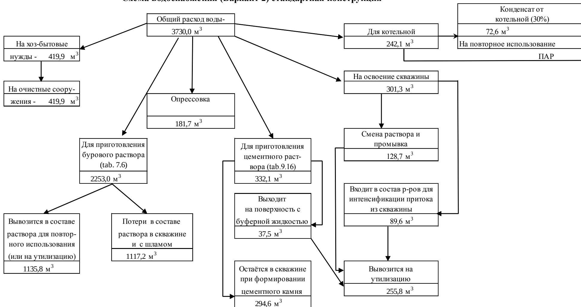
Рисунок 3.6 – Схема водопотребления и водоотведения при строительстве скважины 98103 (C2_13) вариант 2
