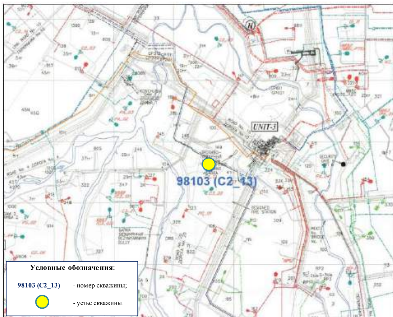
Рисунок 3.2 – Карта-схема расположения проектируемой скважины 98103 (C2_13)
