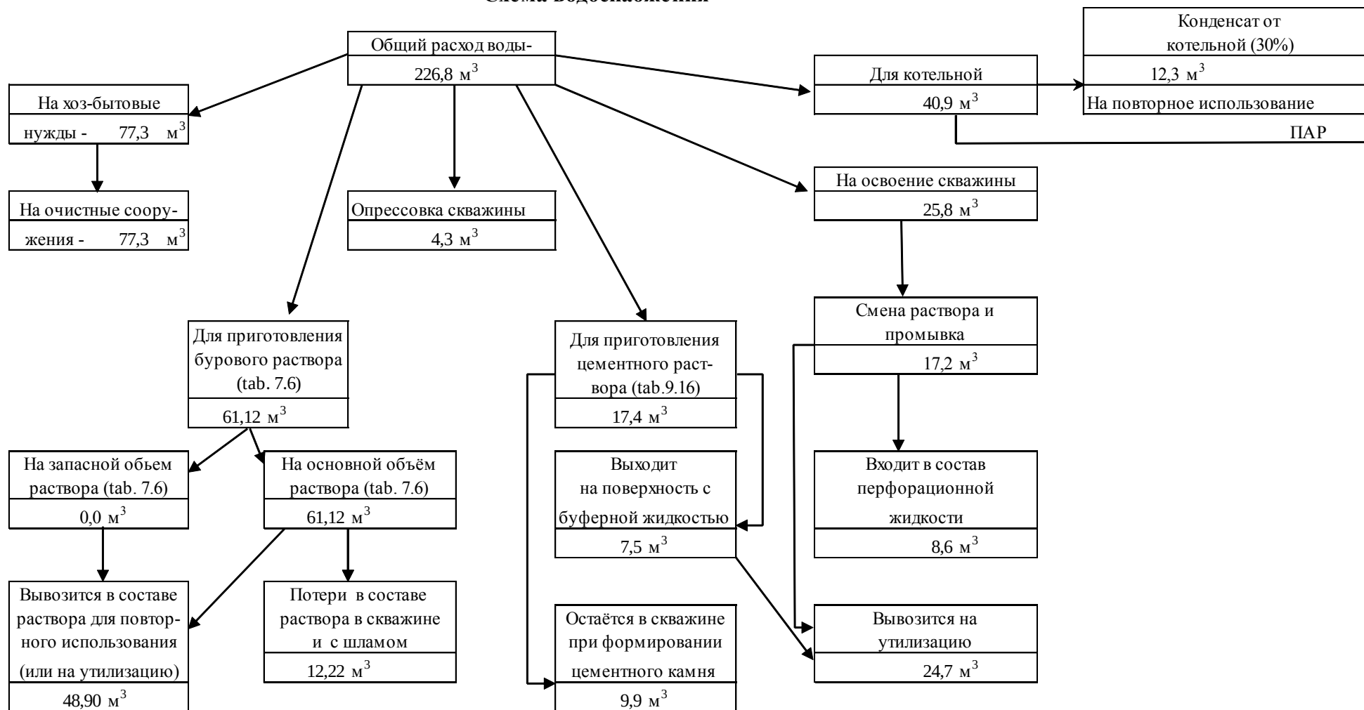
Рисунок 3.5 – Схема водопотребления и водоотведения при строительстве одной водозаборной скважины
