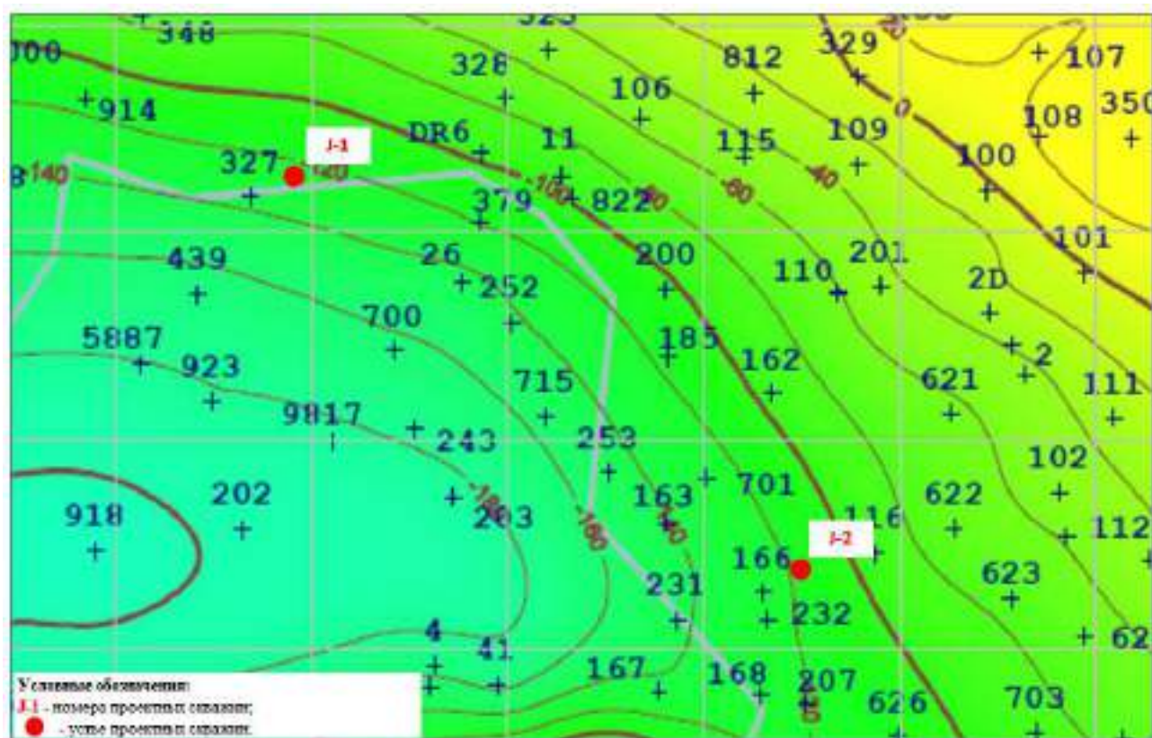
Рисунок 3.3 – Карта-схема расположения проектируемых скважин J-1 и J-2
