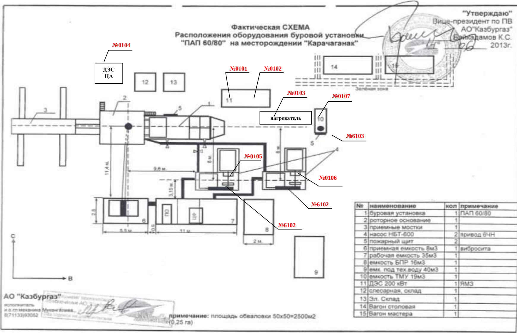
Рисунок 3.4 – Карта-схема буровой площадки ПАП60/80 с источниками выбросов загрязняющих веществ
