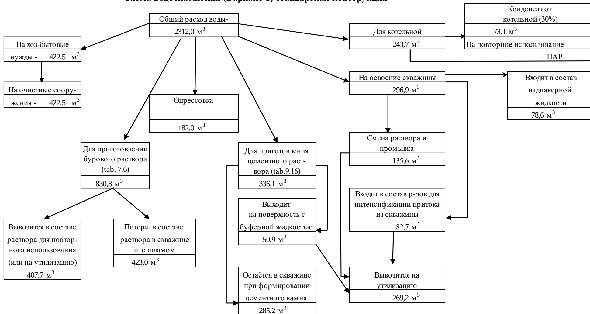
Рисунок 3.5 – Схема водопотребления и водоотведения при бурении добывающей скважины 98110 (Е2_03)
