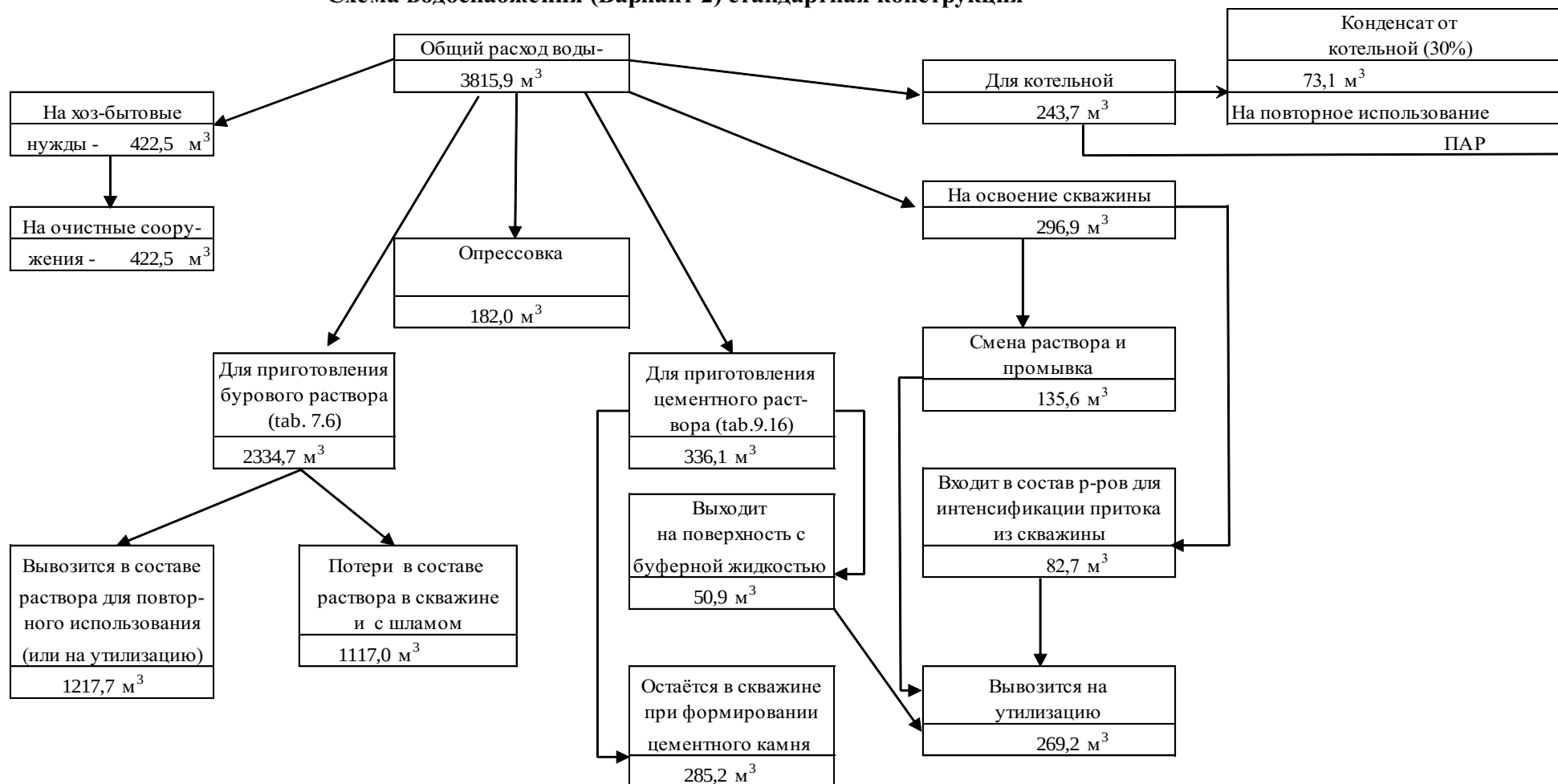
Схема водоснабжения (Вариант 2) стандартная конструкция
