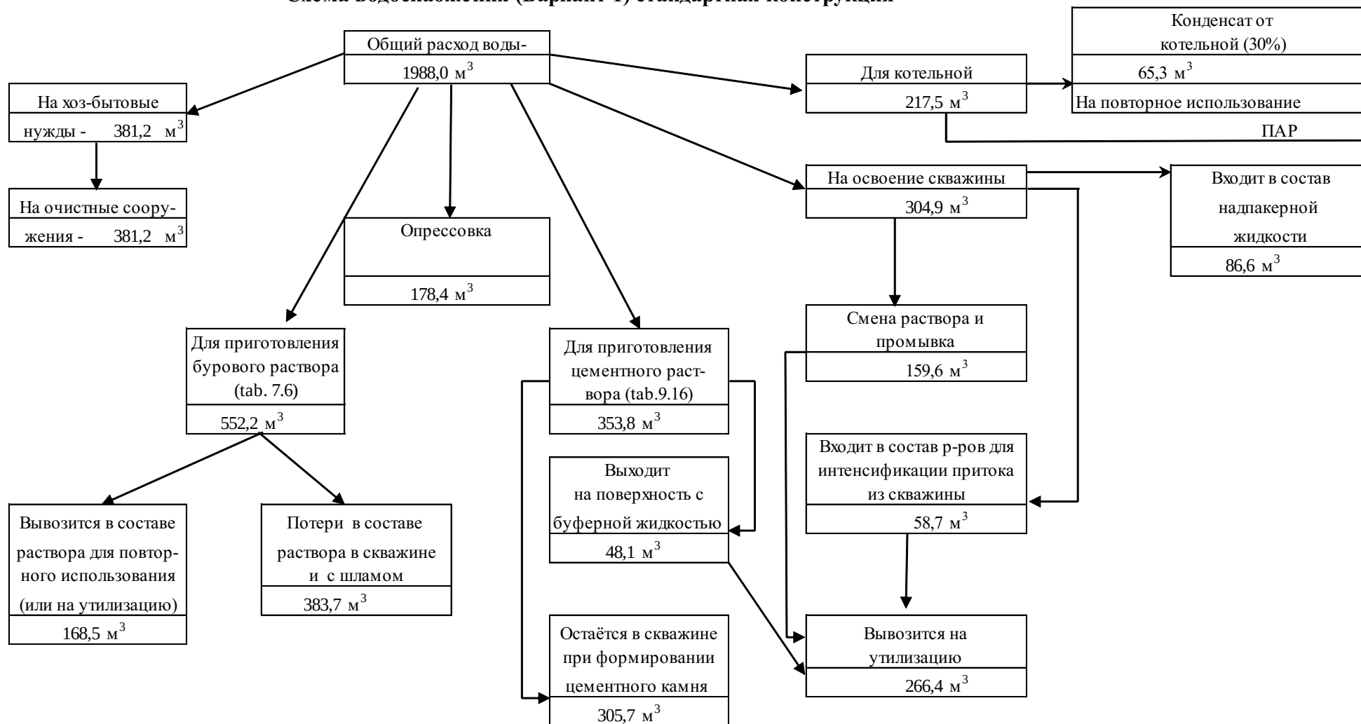
Рисунок 3.5 – Схема водопотребления и водоотведения при строительстве скважины 98105 (PG_02) вариант 1
