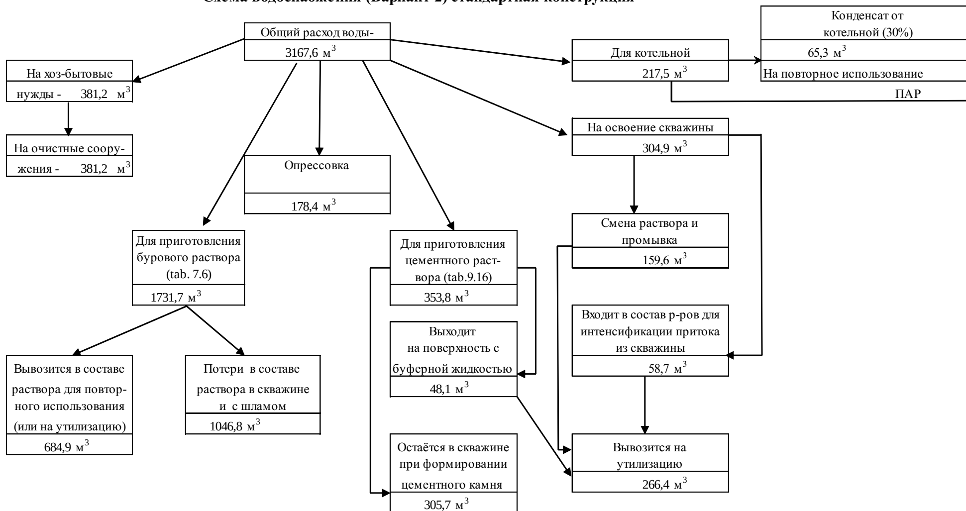
Рисунок 3.6 – Схема водопотребления и водоотведения при строительстве скважины 98105 (PG_02) вариант 2
