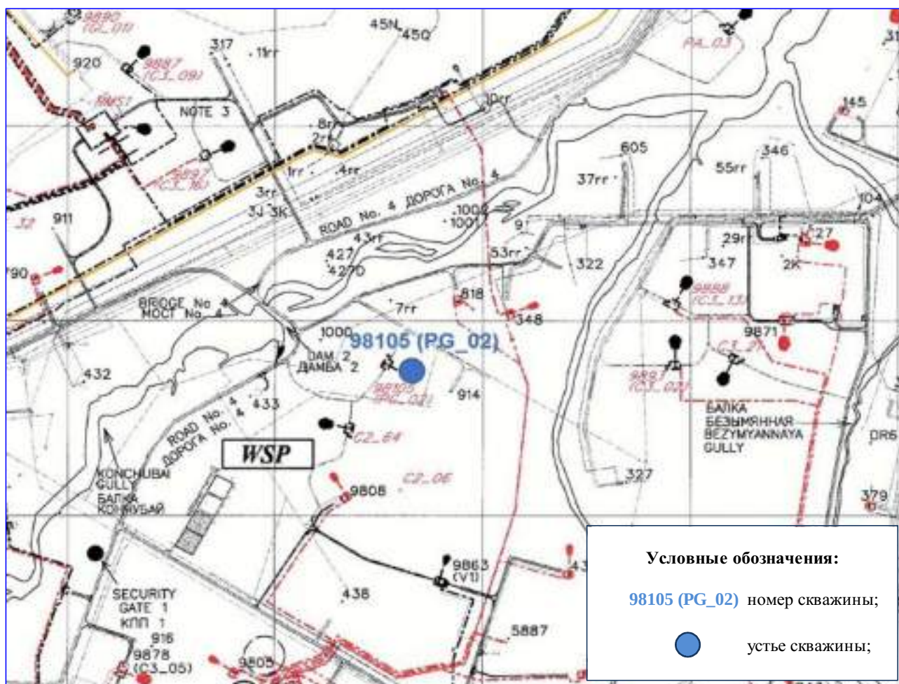
Рисунок 3.2 – Карта-схема расположения проектируемой скважины 98105 (PG_02)
