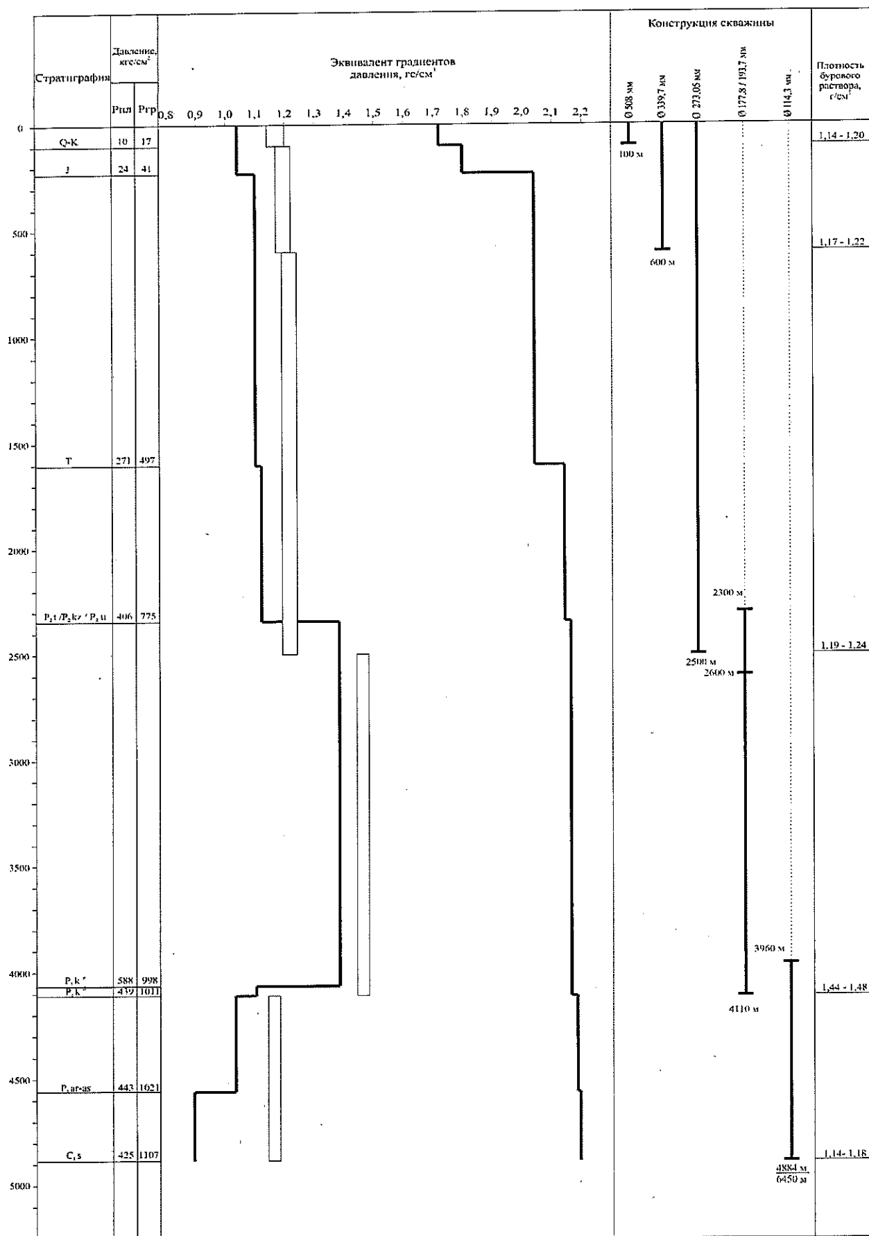
Рисунок 5.1_2- Совмещенный график давлений (облечённая конструкция)
