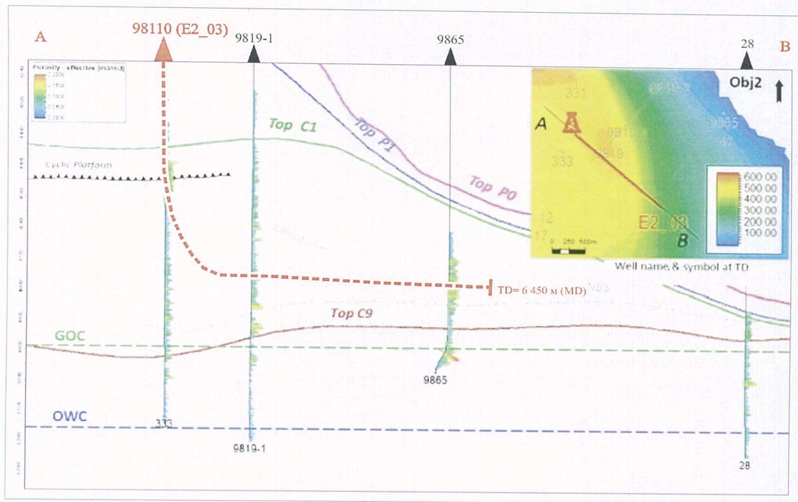
Рисунок 4.1 - Профиль скважины
