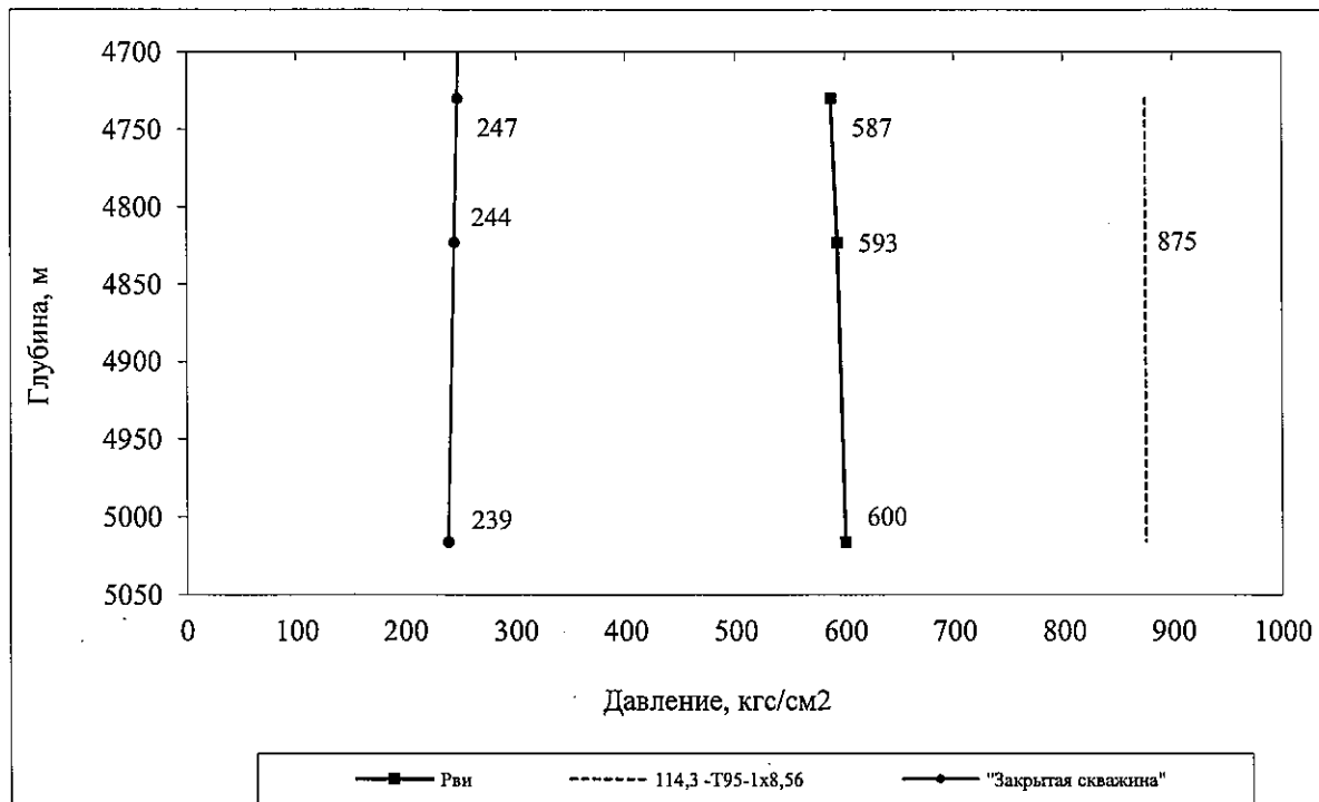
Рисунок 9.14- График избыточных внутренних давлений
