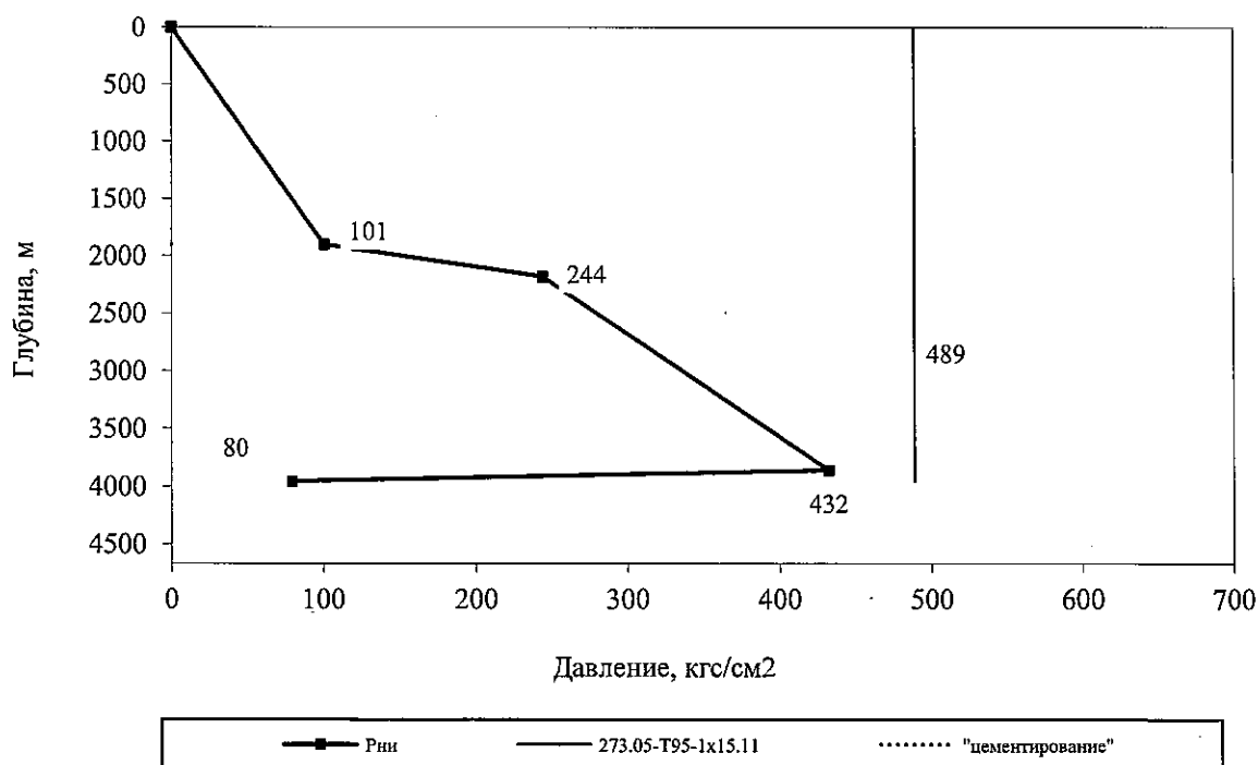
Рисунок 9.5- График избыточных наружных давлений
