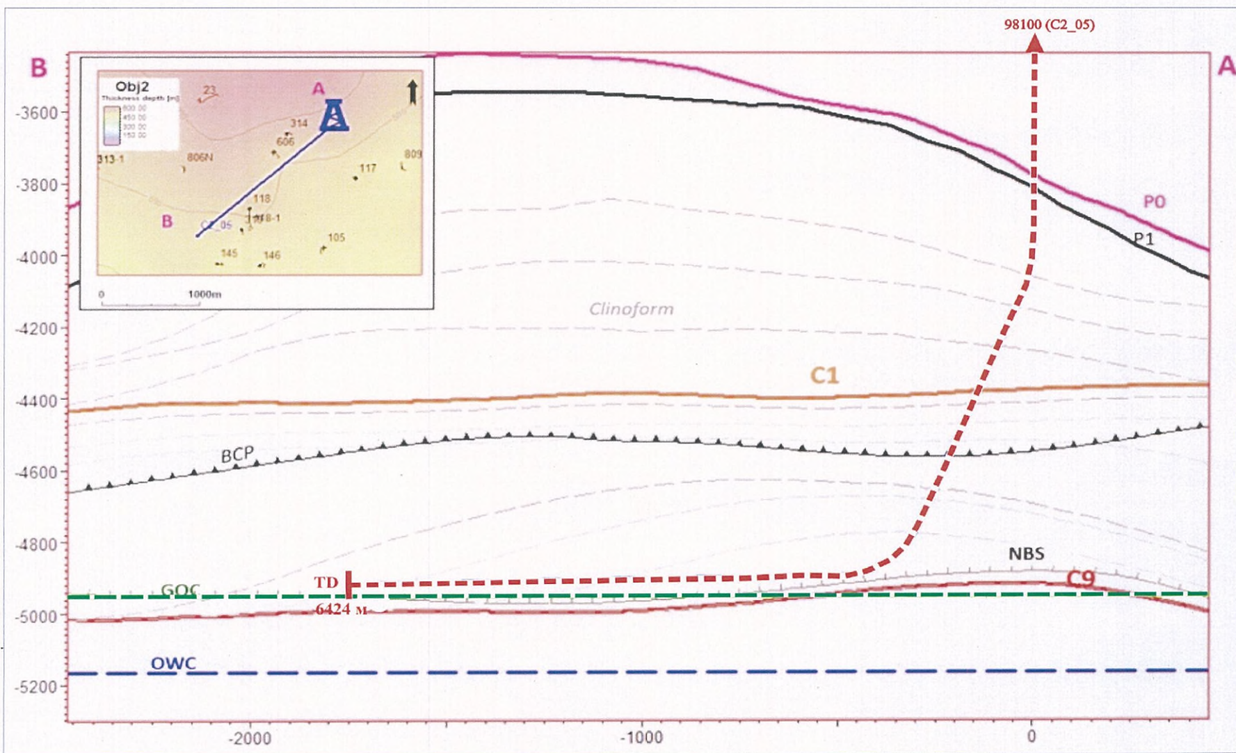
Рис. 4.1 - Профиль скважины
