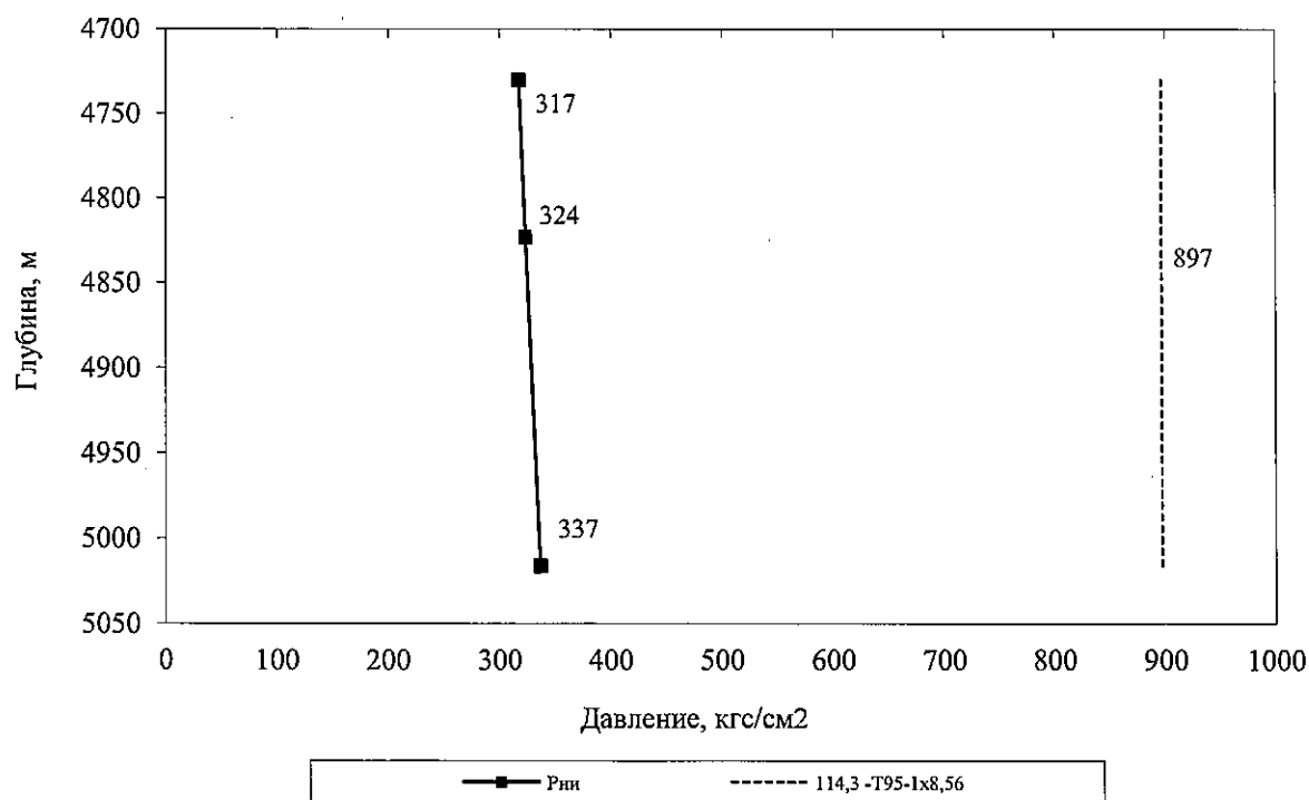
Рисунок 9.13- График избыточных наружных давлений
