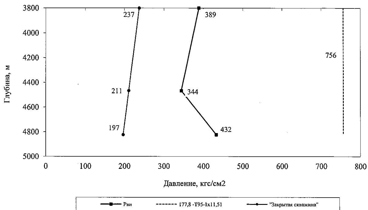
Рисунок 9.10- График избыточных внутренних давлений
