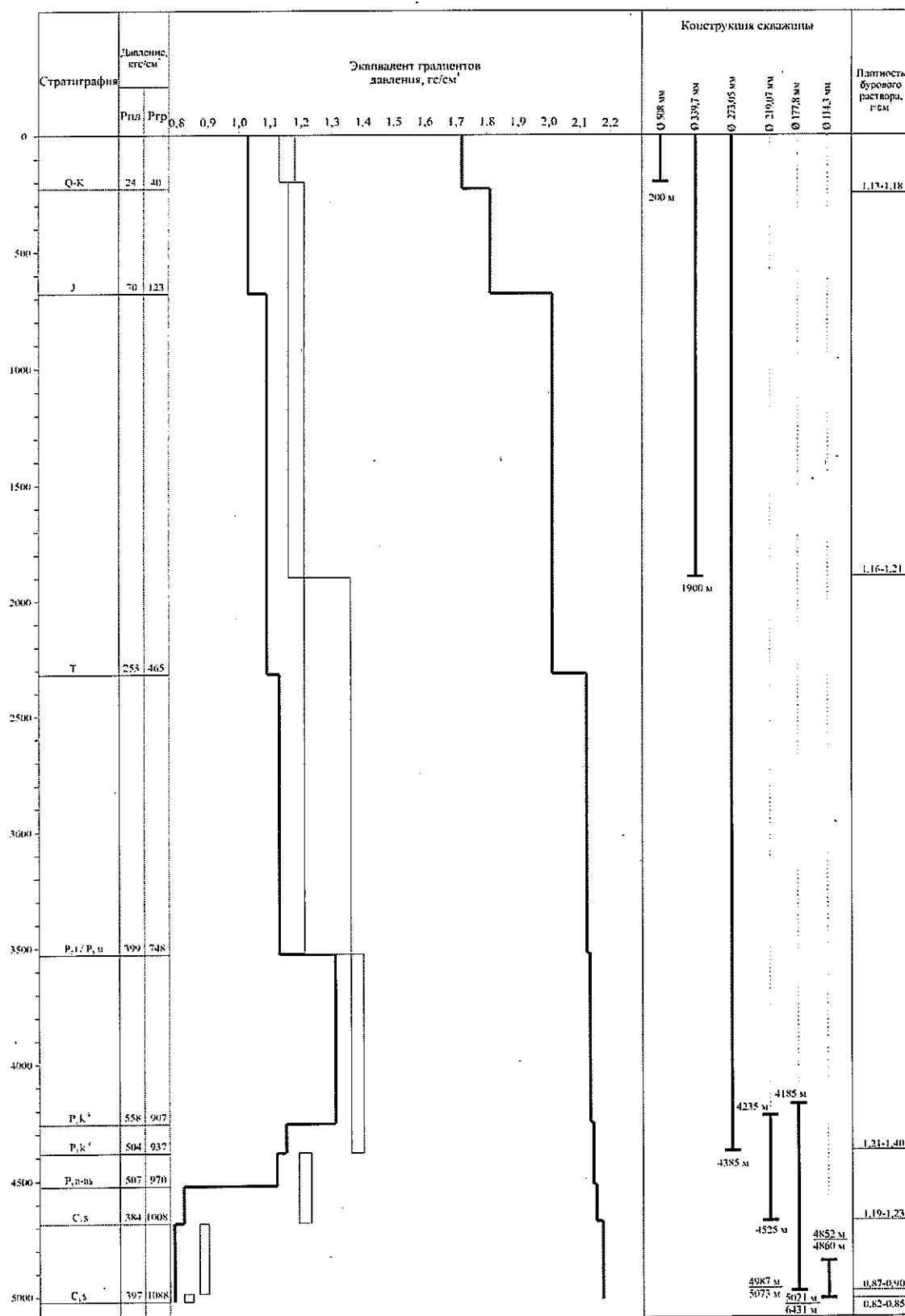
Рисунок 5.1- Совмещенный график давлений
