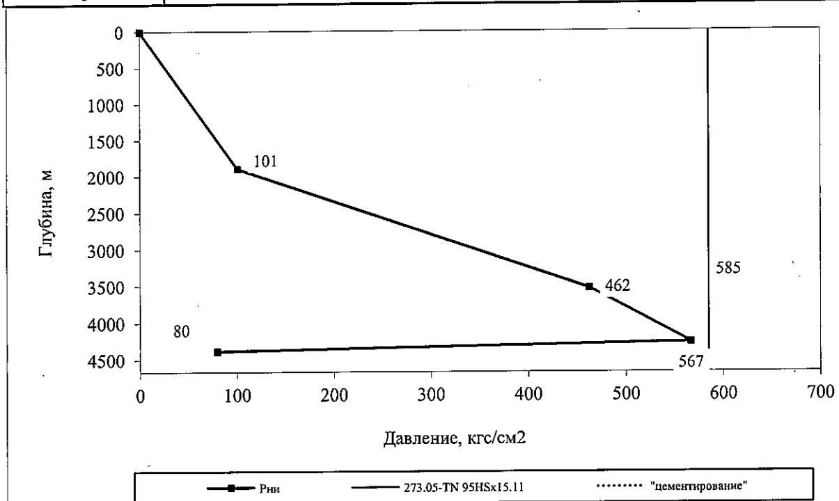
Рисунок 9.5- График избыточных наружных давлений
