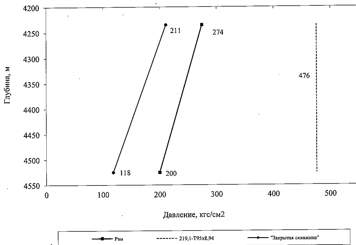
Рисунок 9.8- График избыточных внутренних давлений
