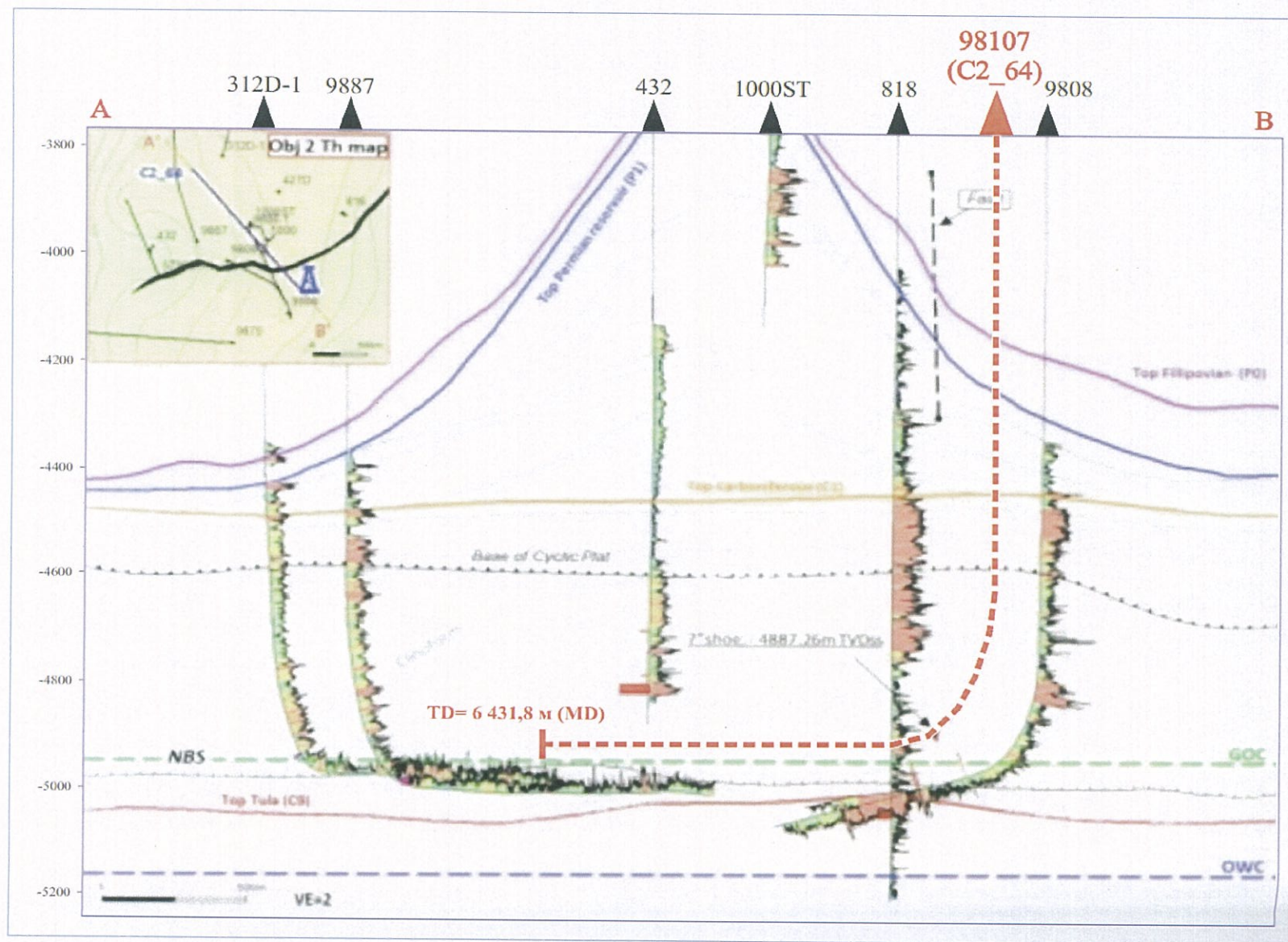
Рисунок 4.1 - Профиль скважины
