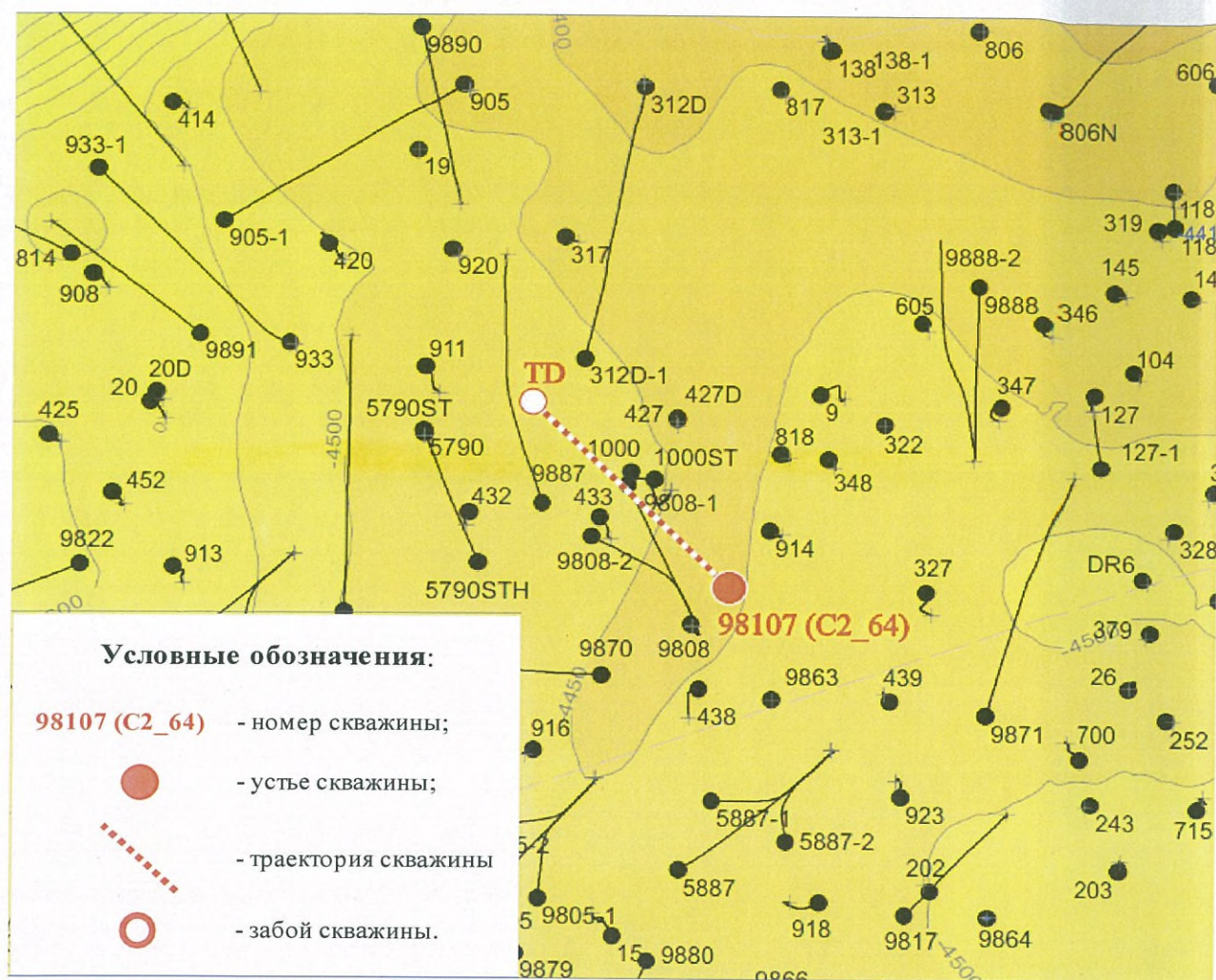
Рисунок 4.2 - Структурная карта по кровле C_1
