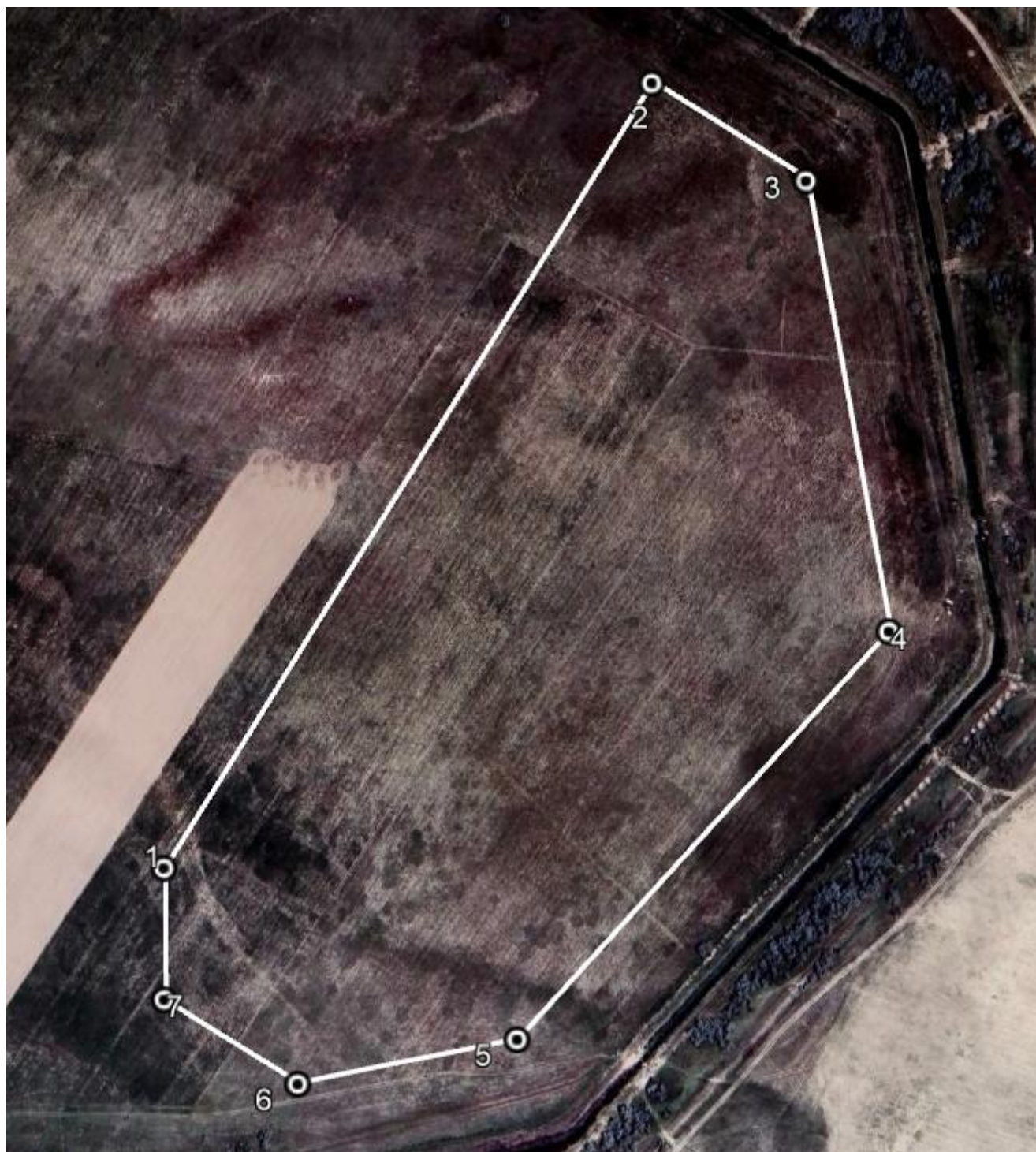
Рис.1.2 Схема участка «Грунтовый резерв-1» с расположением угловых точек (на основе космоснимка)
