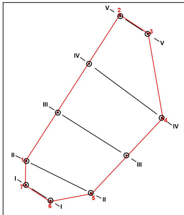
Схема расположения проектных скважин Проявление «Грунтовый резерв №1» Масштаб 1:5 000
