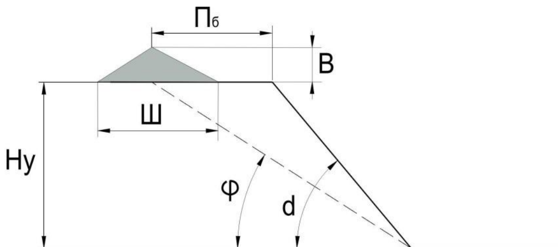
Рис.3.4.1 Схема уступа
