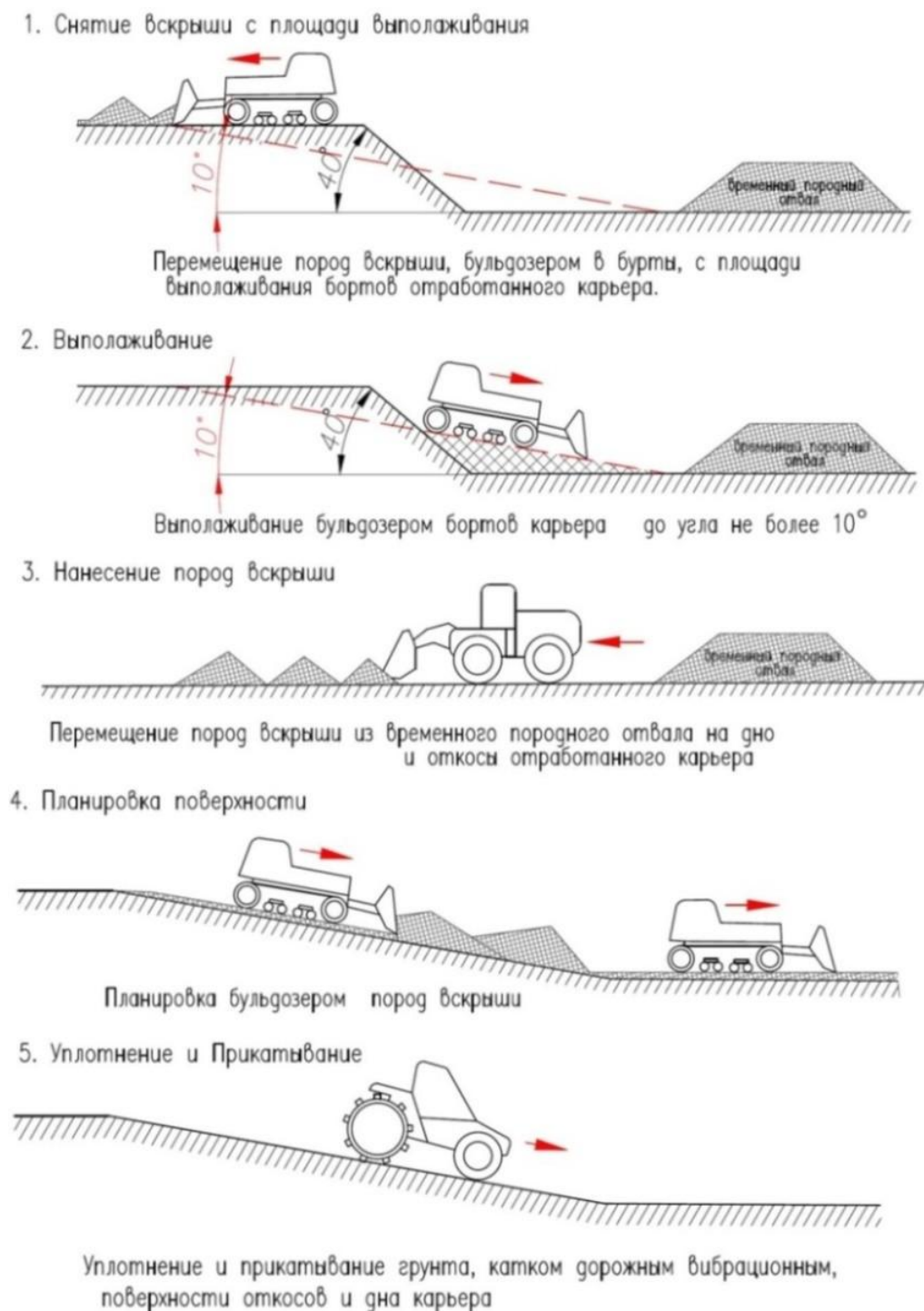
Рис. 7.3.2 Принципиальная схема рекультивации
