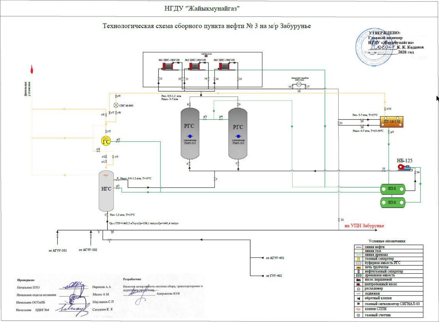
Рисунок 1.9- Технологическая схема подготовки нефти №3 на м/р Забурунье
