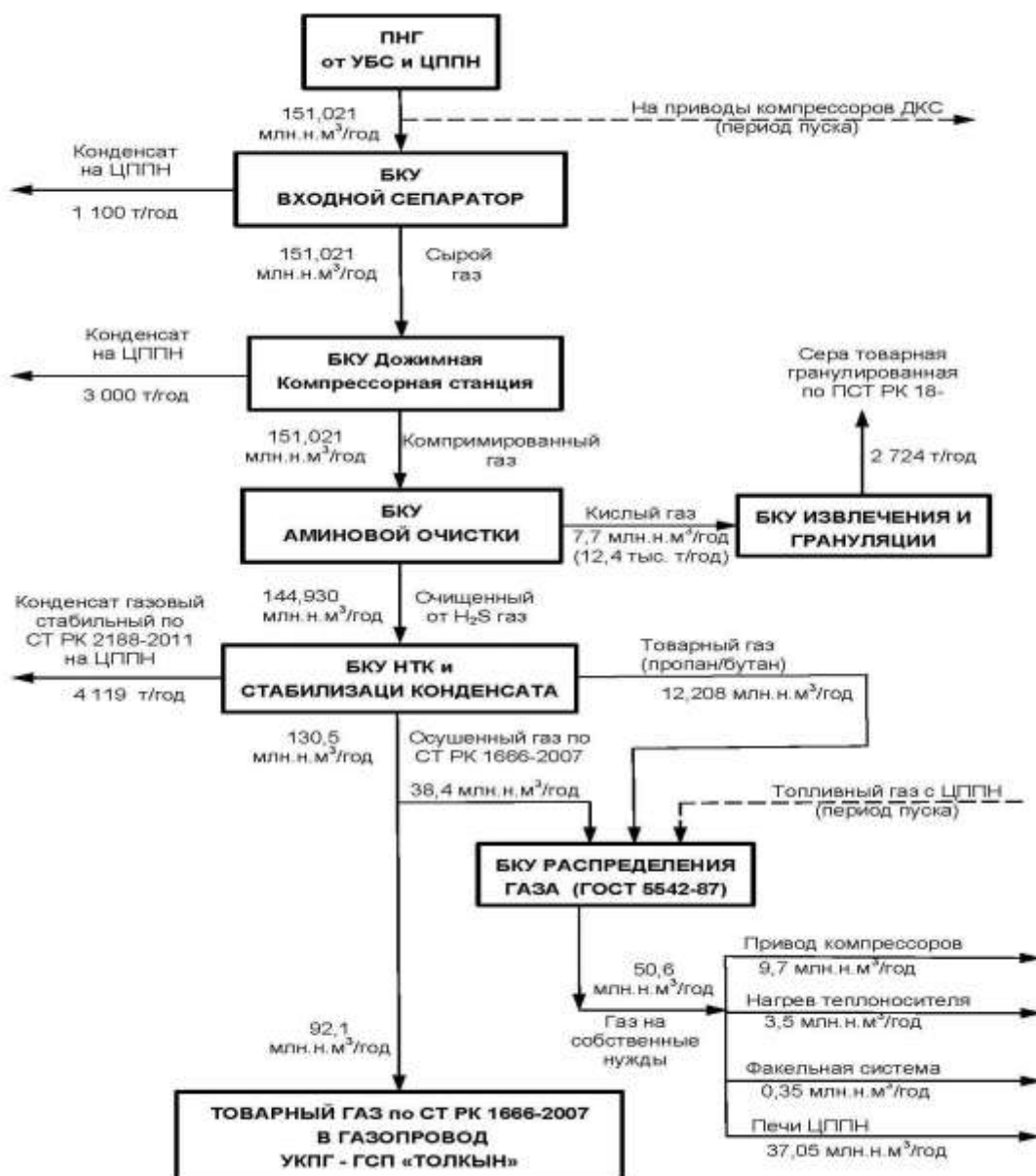
Рисунок 8.1 - Блок – схема переработки попутного газа на УКПГ
