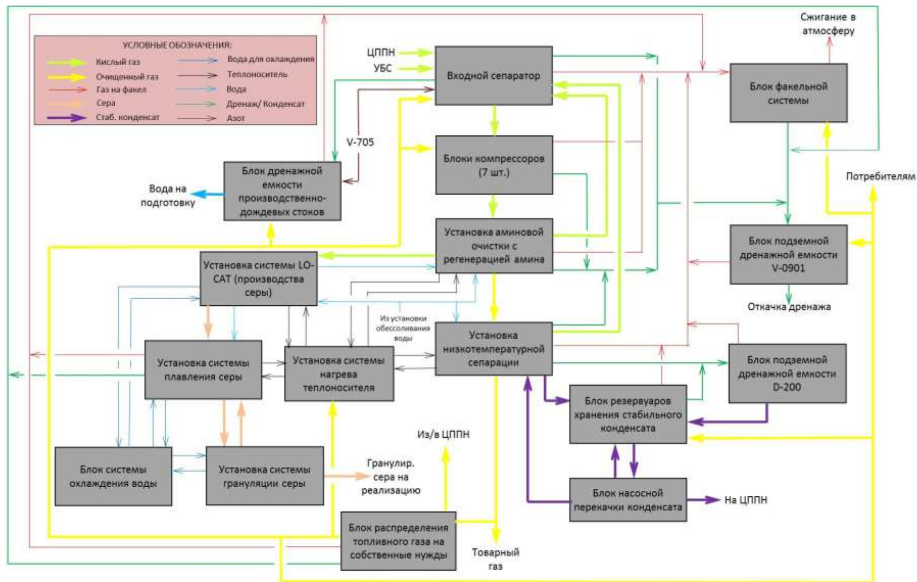
Рисунок 8.2 - Технологическая схема УКПГ
