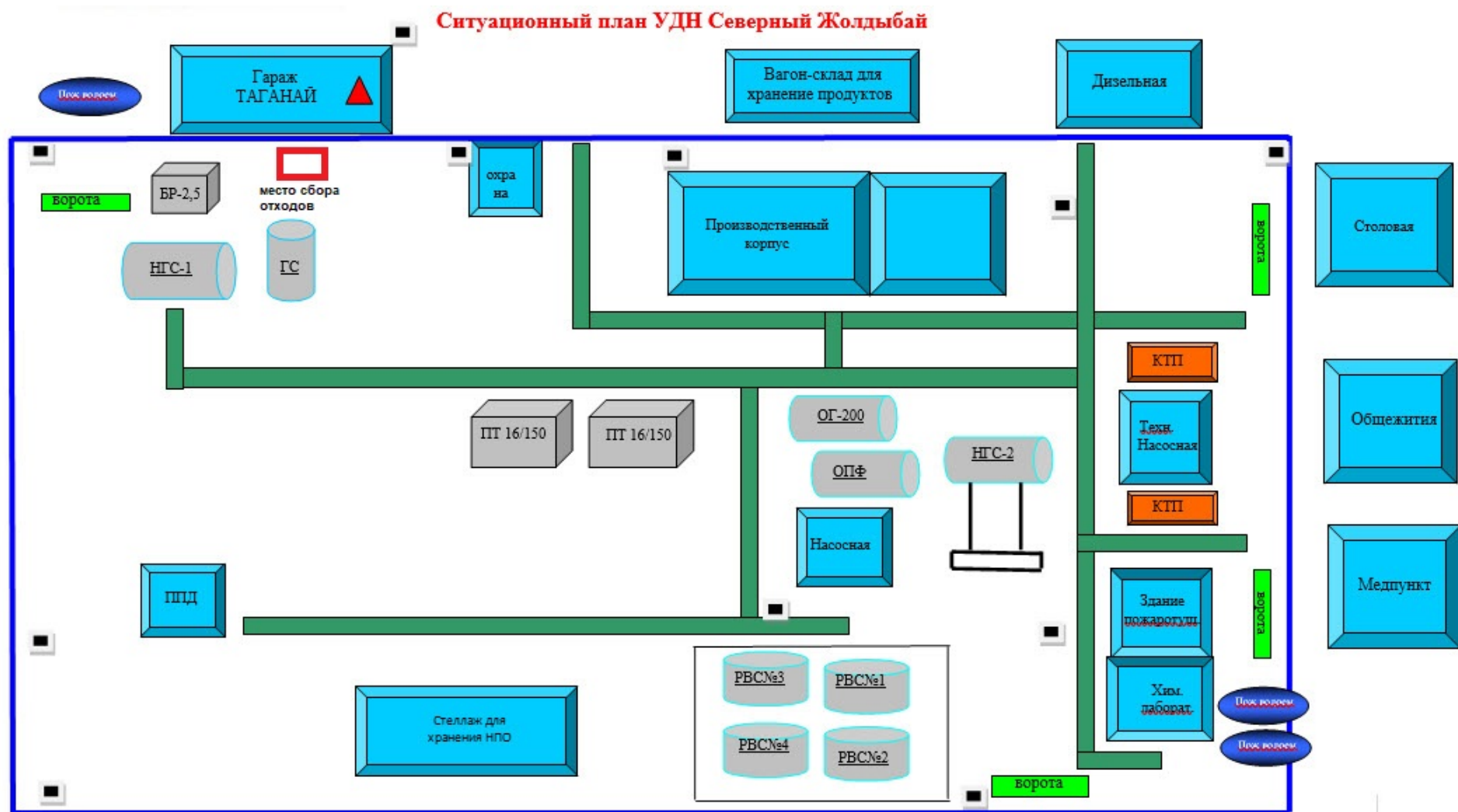
Рис.2.5 – Технологическая схема сбора нефти Северный Жолдыбай
