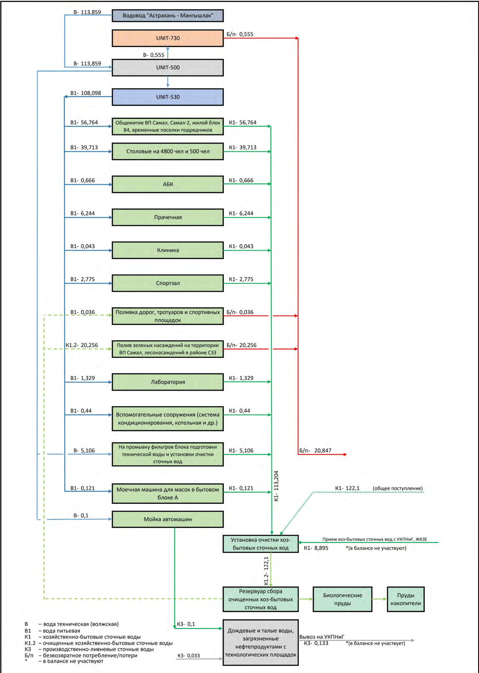
Рисунок 4.4.1 Балансовая схема водопотребления и водоотведения в период с 12 сентября по 31 декабря 2026 года
