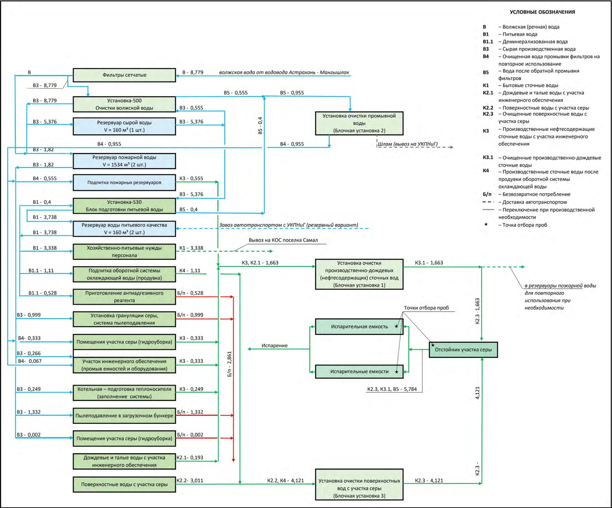
Рисунок 4.4 Балансовая схема водопотребления и водоотведения в период с 12 сентября по 31 декабря 2026 года, тыс. м³/период
