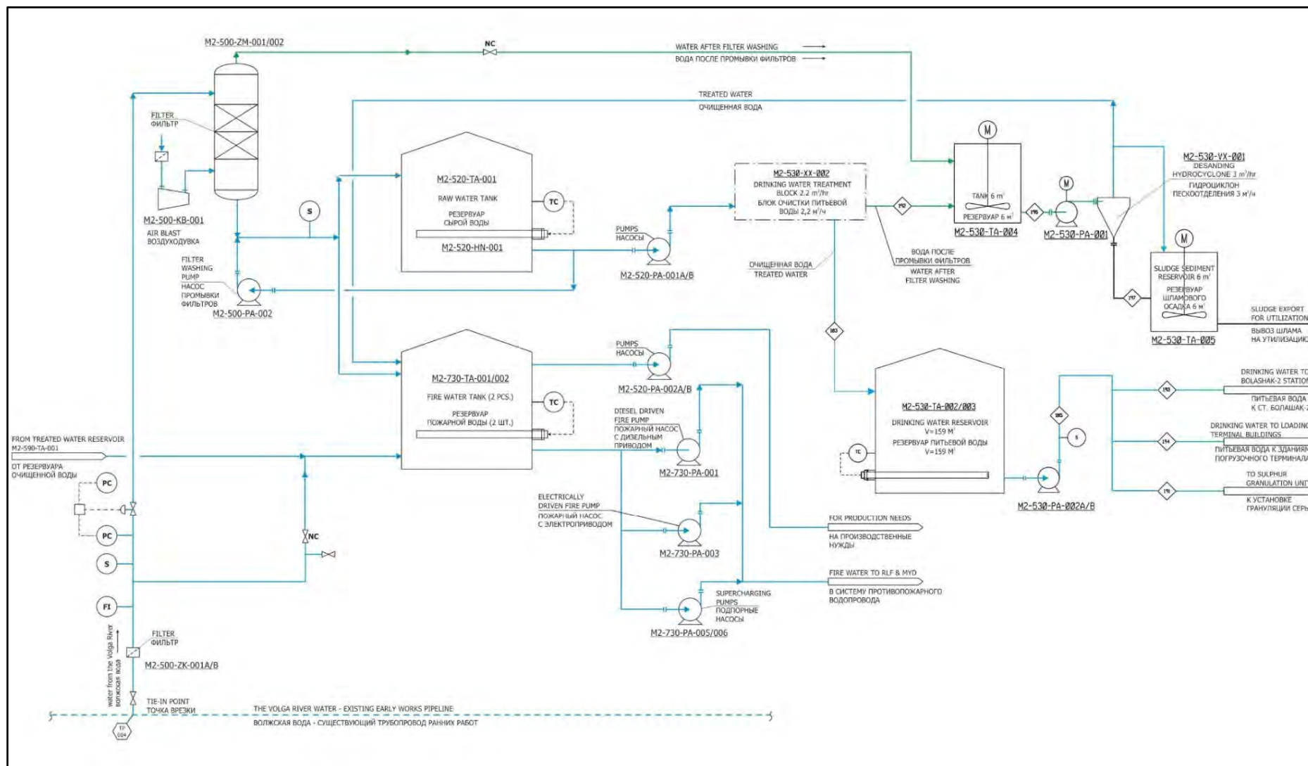
Рисунок 4.1 Принципиальная технологическая схема водоснабжения
