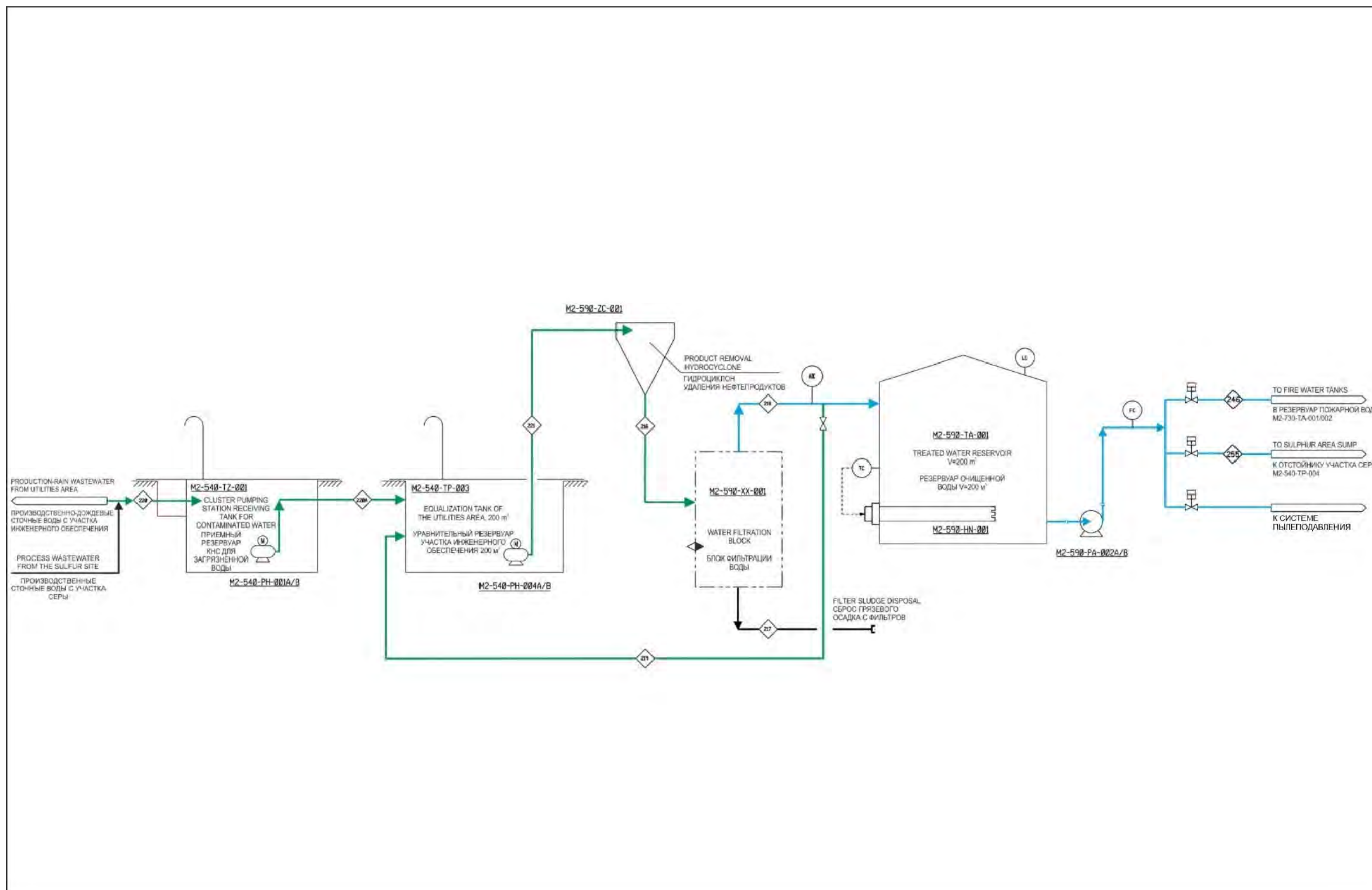
Рисунок 4.3 Принципиальная технологическая схема сбора, очистки и сброса производственно-дождевых вод с участка инженерного обеспечения
