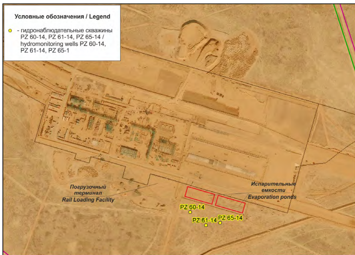
Рисунок 3.1 Карта - схема оператора с расположением очистных сооружений ЖКЗЕ, мониторинговых и наблюдательных скважин в районе испарительных емкостей
