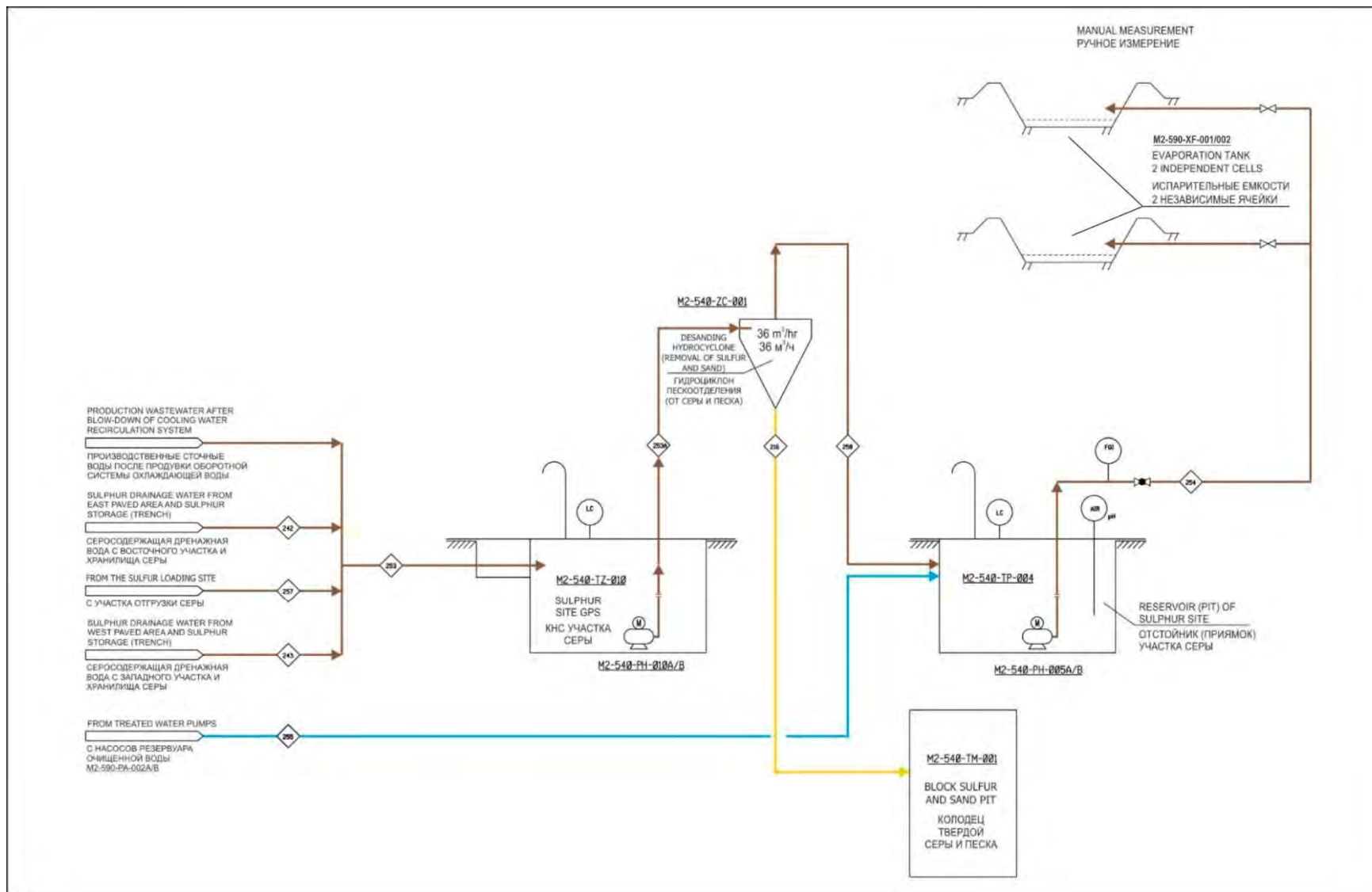
Рисунок 4.2 Принципиальная технологическая схема сбора, очистки и сброса поверхностных вод с участка серы
