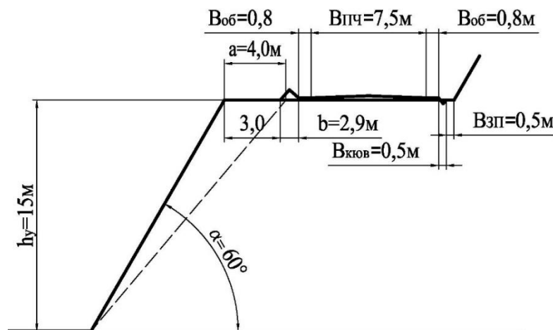
Рисунок 3.2 – Схема поперечного профиля транспортной бермы
