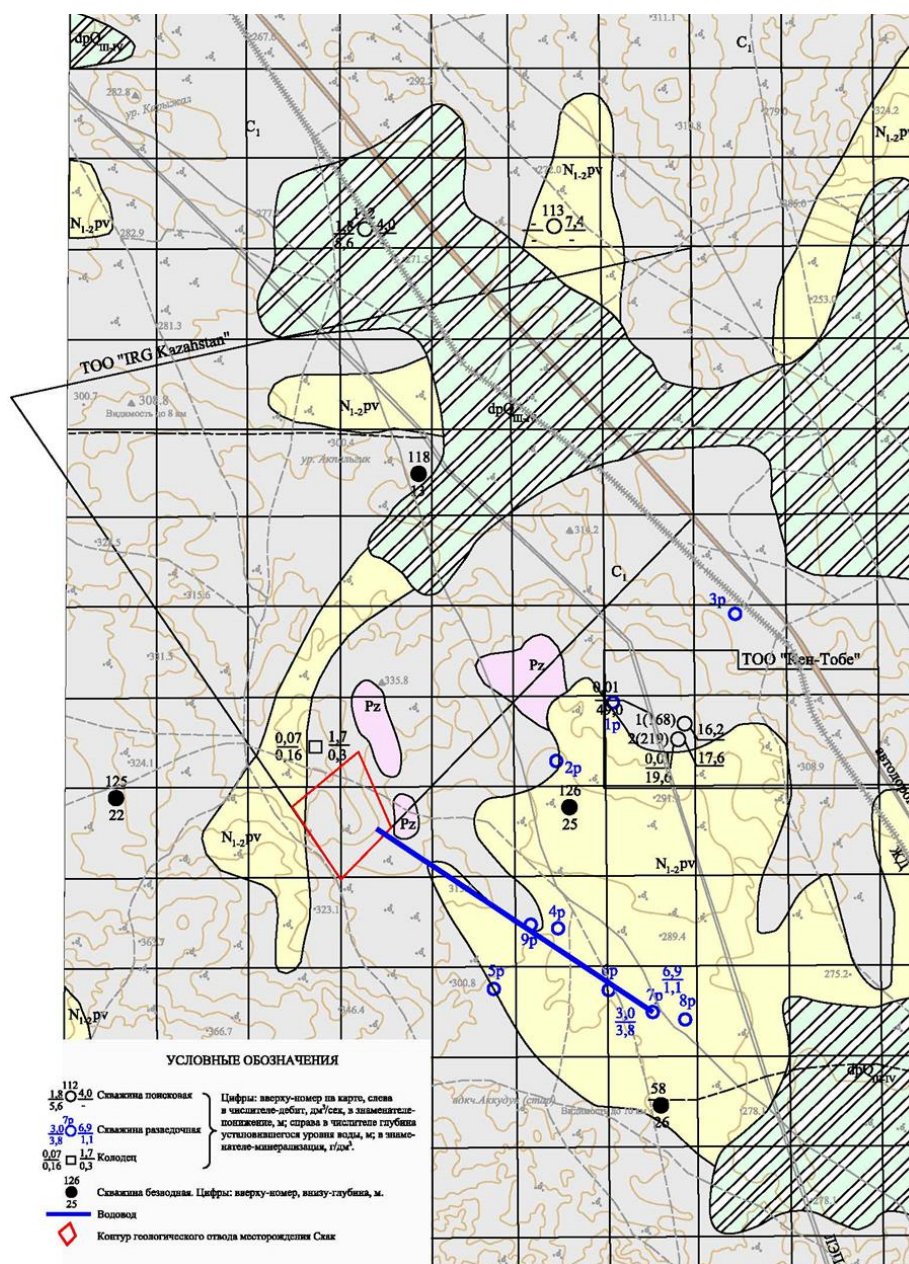
Рисунок 2.1 – Схема прокладки водовода для технического водоснабжения на месторождениях Кедейского рудного узла
