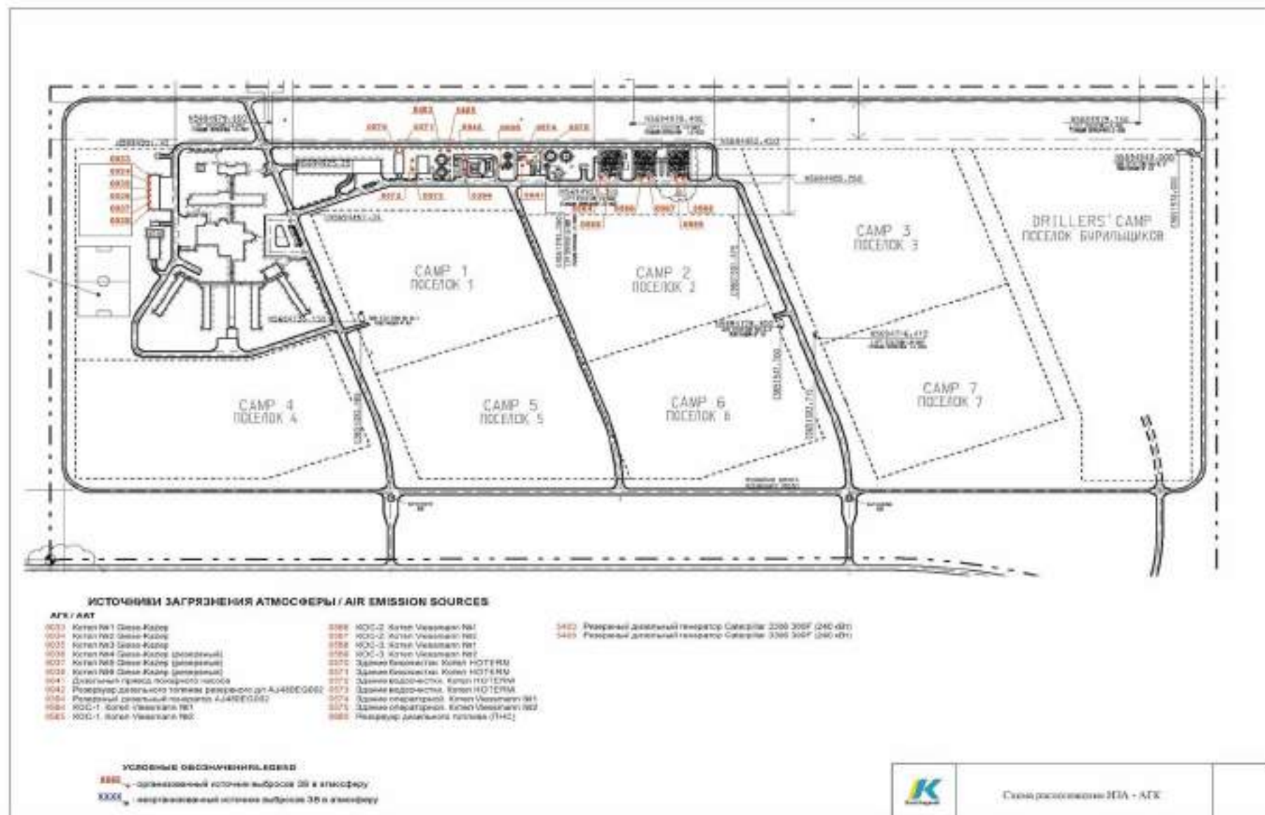
Рисунок 2.1.4 Схема расположения ИЗА-АГК
