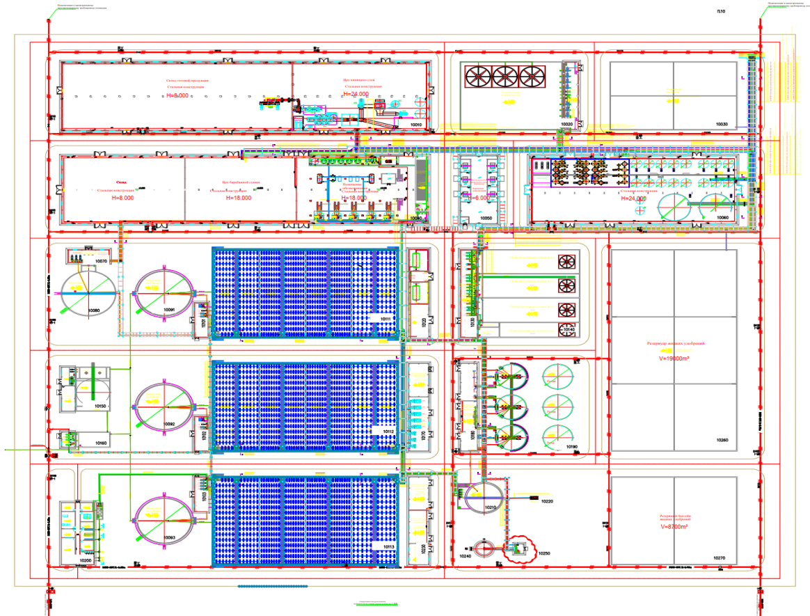
Планировка третьего этажа здания обезвоживания
