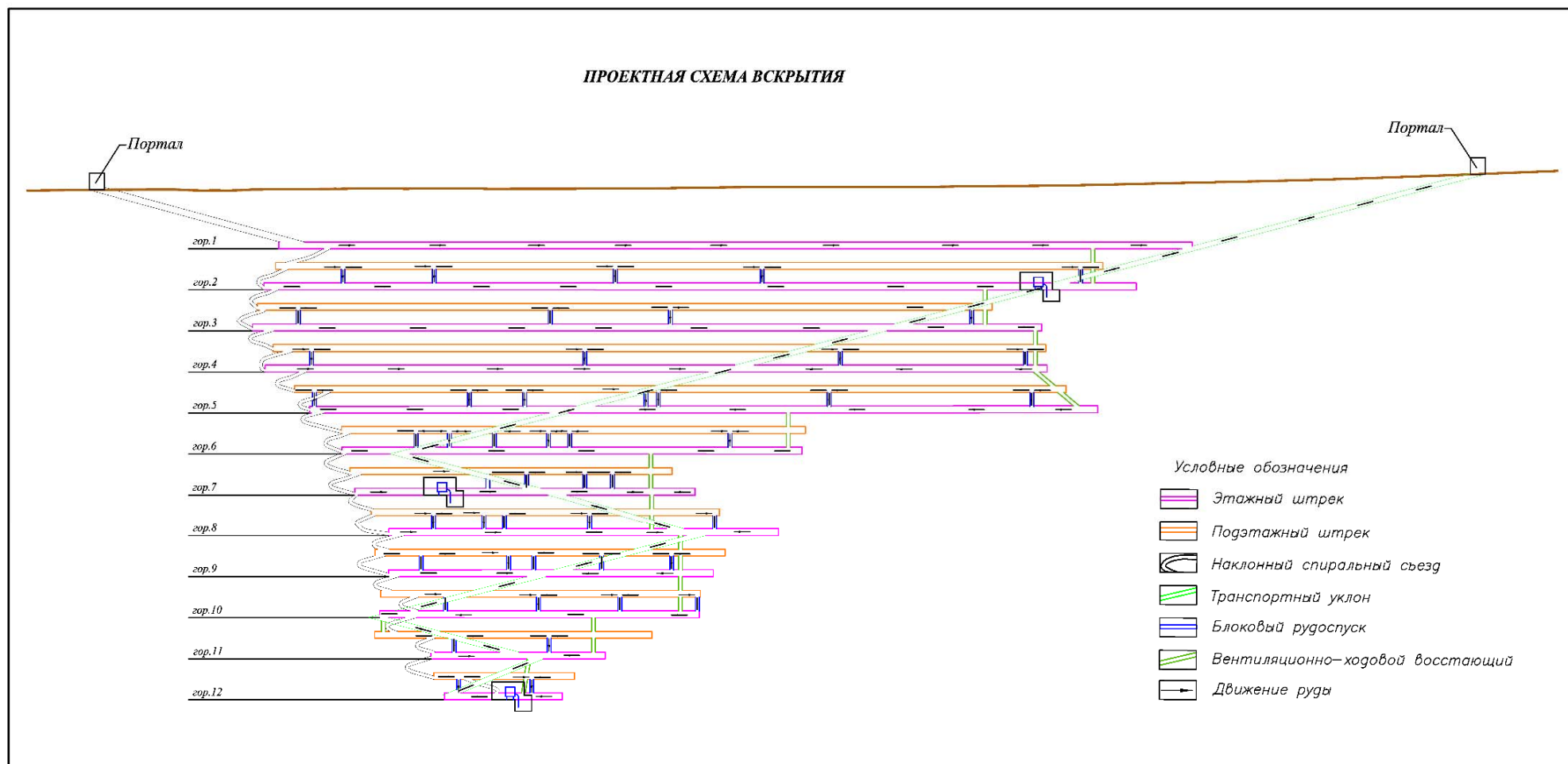
Рисунок 4.3.1 Схема вскрытия месторождения Аксоран
