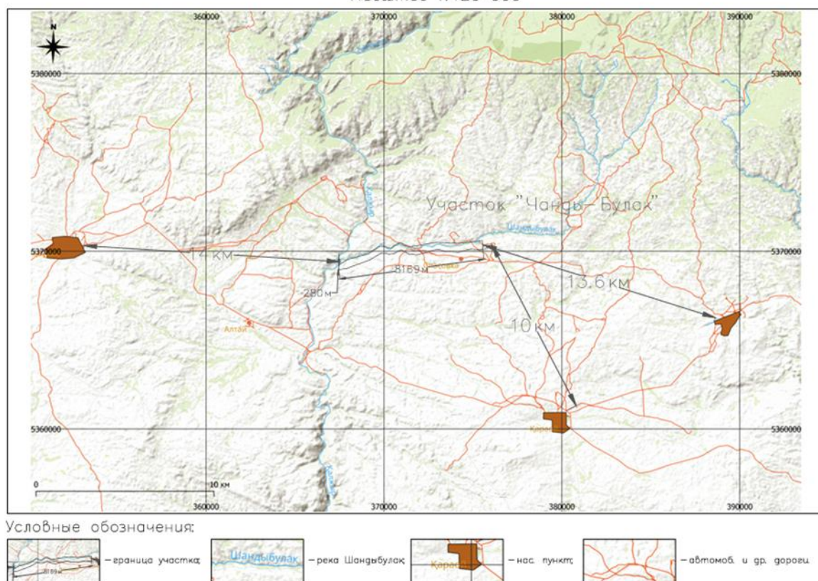
Ситуационная карта-схема расположения участка "Чанды-булак" Масштаб 1:120 000
