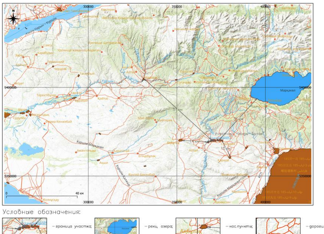
Рис. 1 – Обзорная карта района расположения месторождения «Чанды-Булак» с указанием расстояния до ближайших жилых зон.
