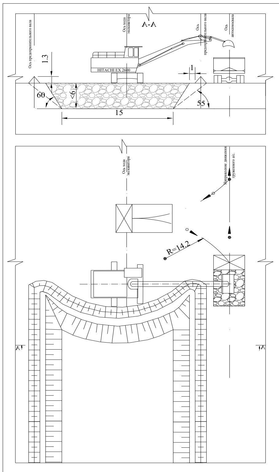
Рисунок 3.6 Схема проходки траншеи (съезда) гидравлическим экскаватором (обратная лопата) с нижним черпанием и погрузкой в автосамосвалы на уровне стояния экскаватора, с тупиковым разворотом
