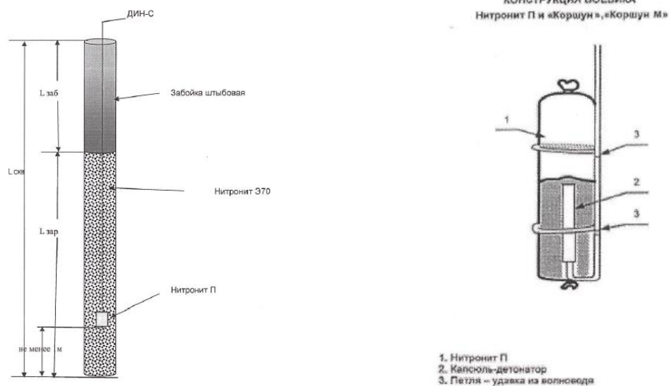
Рисунок 3.9- Параметры конструкции скважинного заряда
