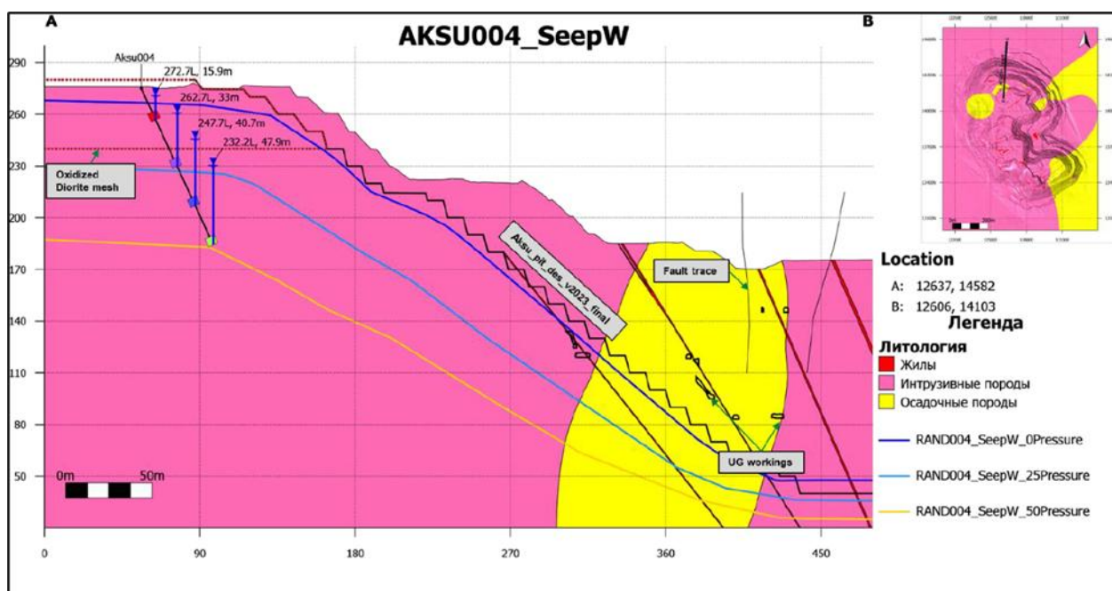
Рисунок 2.9 - Поперечный разрез AKSU004 с геологической моделью и результатами измерения порового давления
