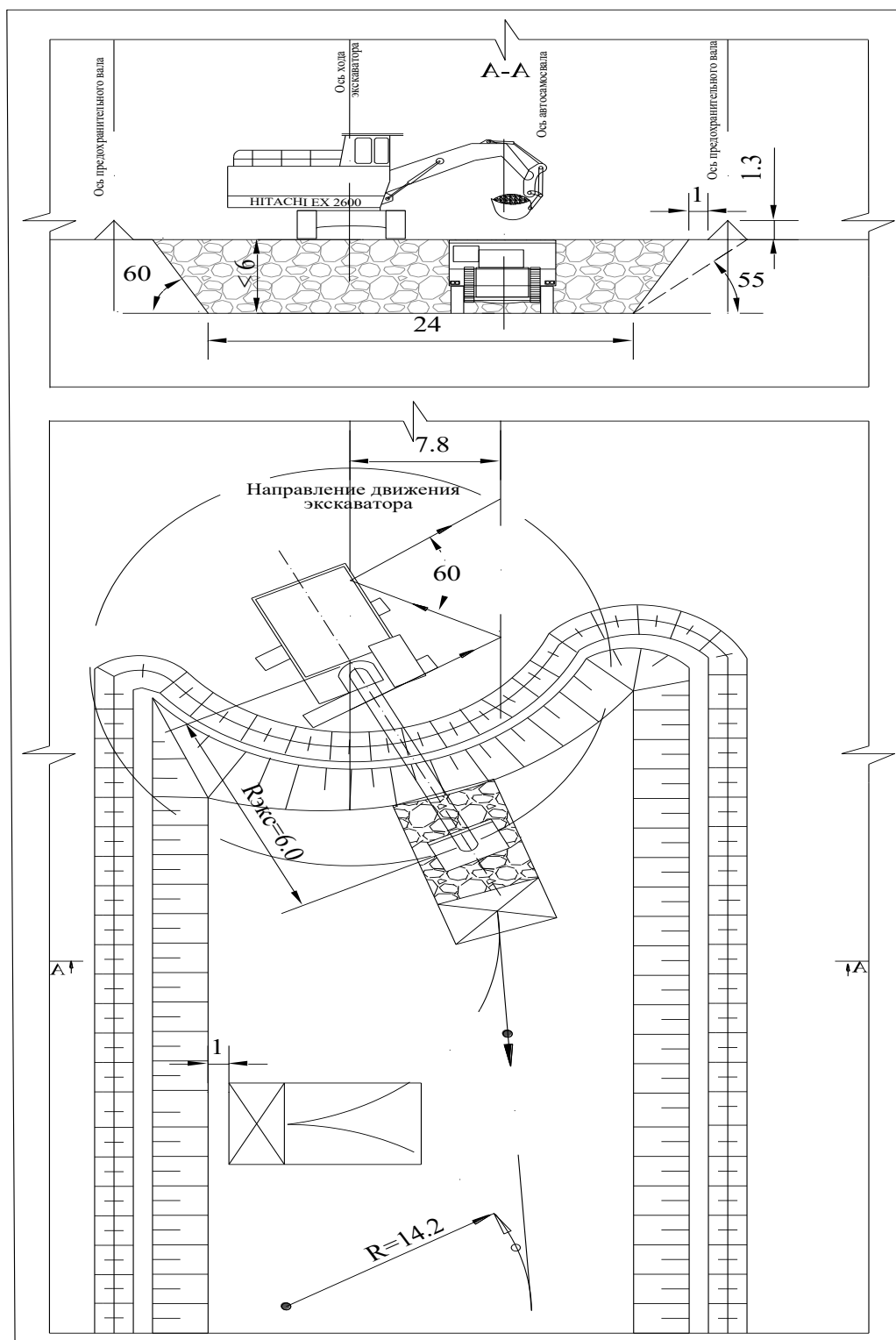
Рисунок 3.4 Схема проходки траншеи (съезда) гидравлическим экскаватором с нижним черпанием и погрузкой в автосамосвалы на уровне подошвы траншеи
