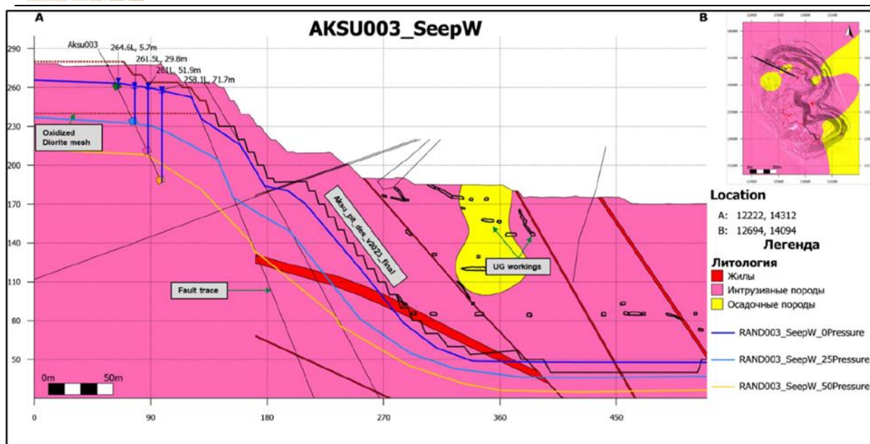
Рисунок 2.8 - Поперечный разрез AKSU003 с геологической моделью и результатами измерения порового давления
