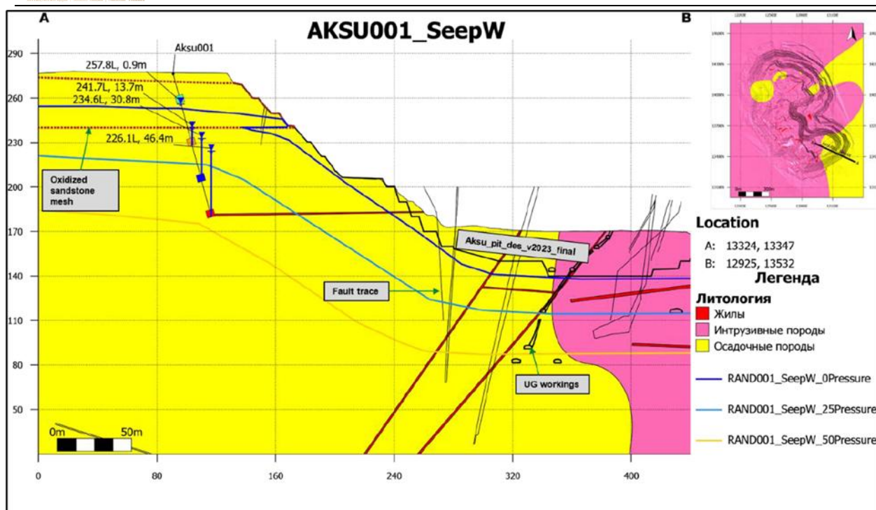
Рисунок 2.6 - Поперечный разрез AKSU0001 с геологической моделью и результатами измерения порового давления
