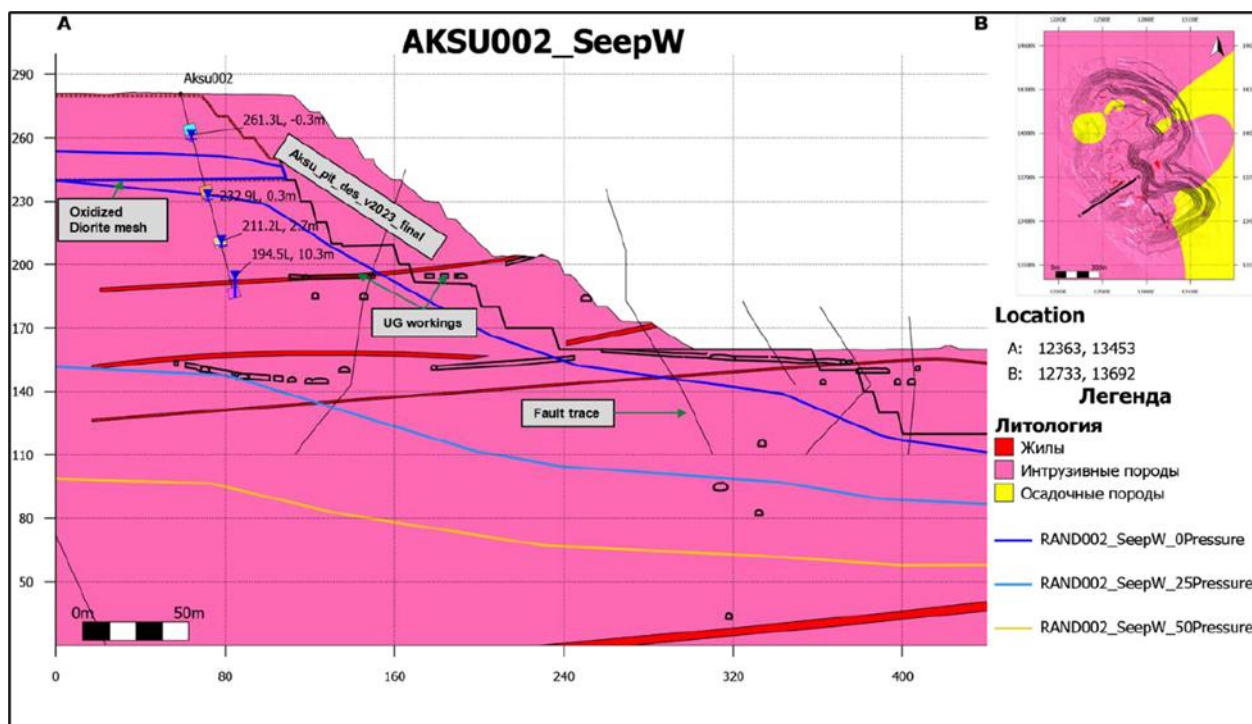
Рисунок 2.7 - Поперечный разрез AKSU002 с геологической моделью и результатами измерения порового давления
