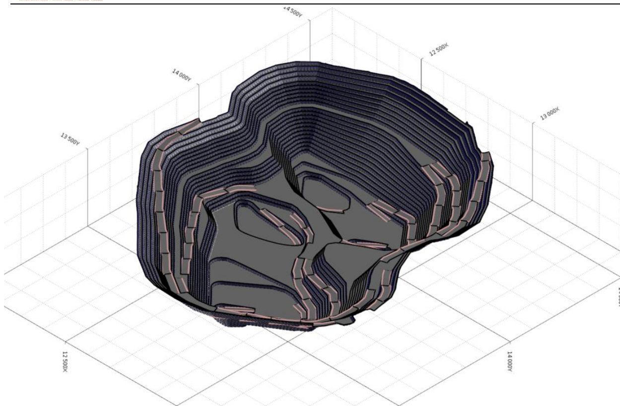
Рисунок 3.1 План карьера месторождения Аксу на конец отработки (изометрический вид на Северо-Запад)
