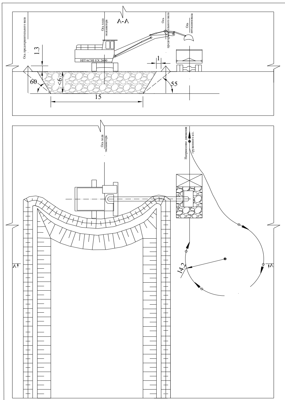
Рисунок 3.5 Схема проходки траншеи (съезда) гидравлическим экскаватором (обратная лопата) с нижним черпанием и погрузкой в автосамосвалы на уровне стояния экскаватора, с петлевым разворотом.
