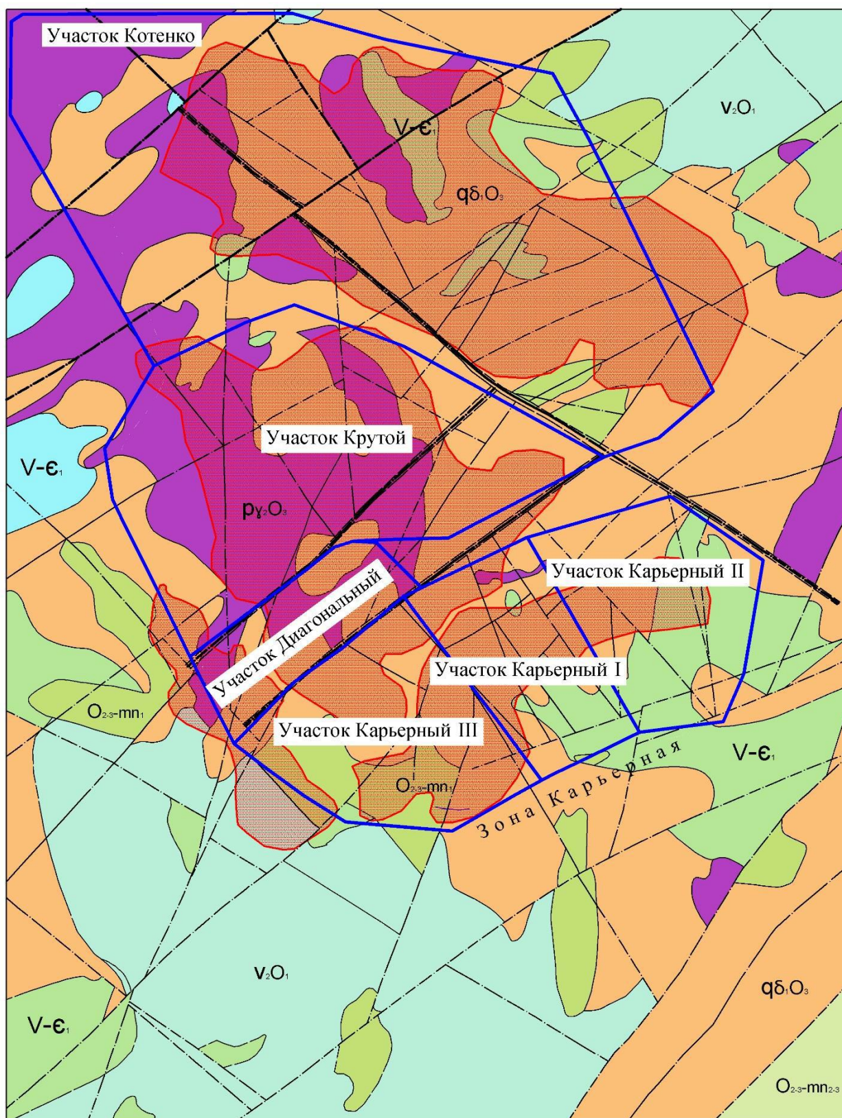
Рисунок 2.2- Геологическая схема месторождения Аксу (II Октябрьская площадь)
