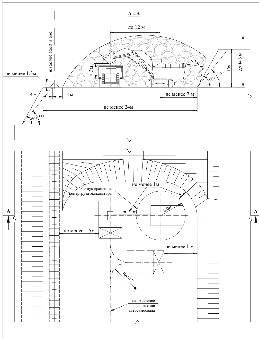
Рисунок 3.7 Схема отработки породного уступа тупиковым забоем экскаватором HITACHI EX 1900 (прямая лопата)
