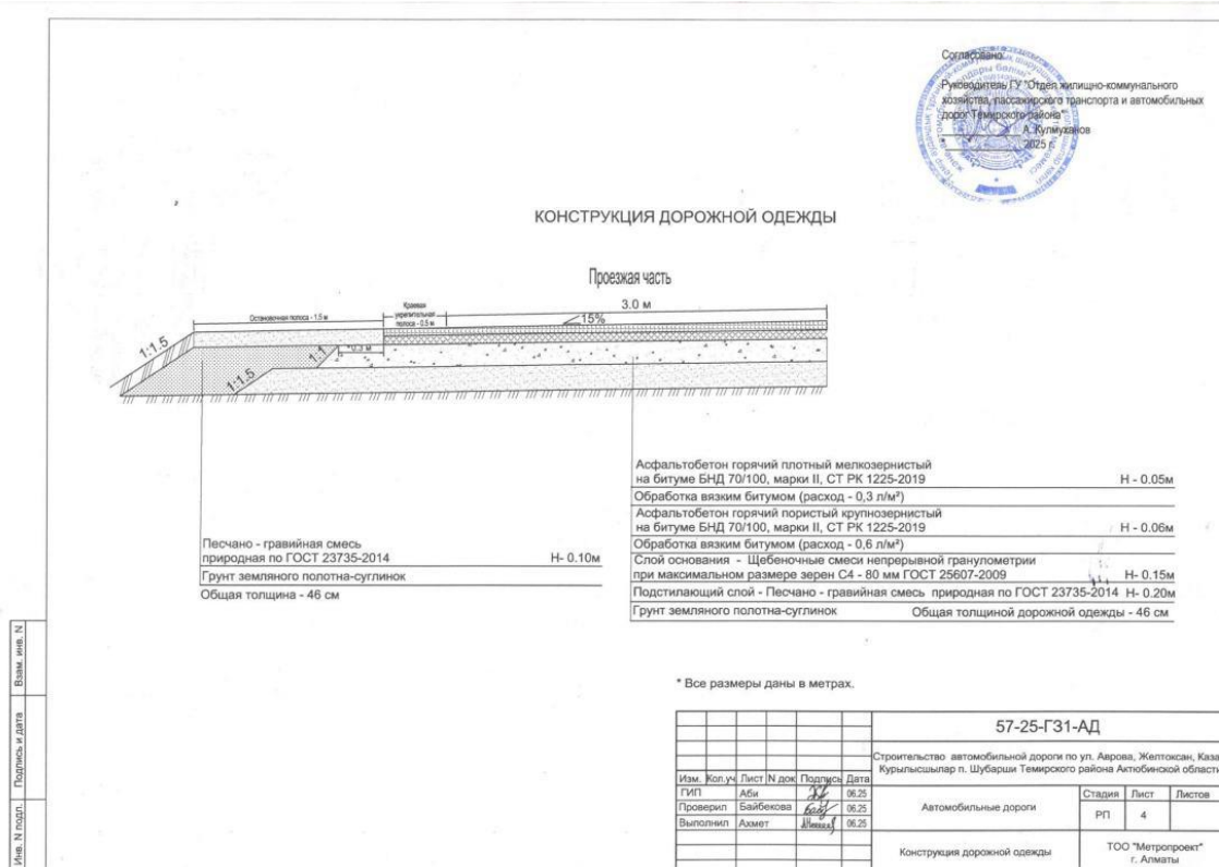
Рисунок-3. Конструкция дорожной одежды.
