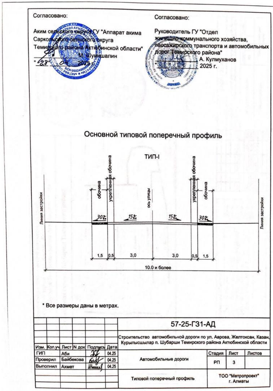
Рисунок-2. Основной типовой поперечный профиль. Земляное полотно
