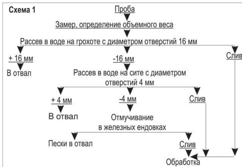
Рисунок 2. Схема отработки технологических проб
