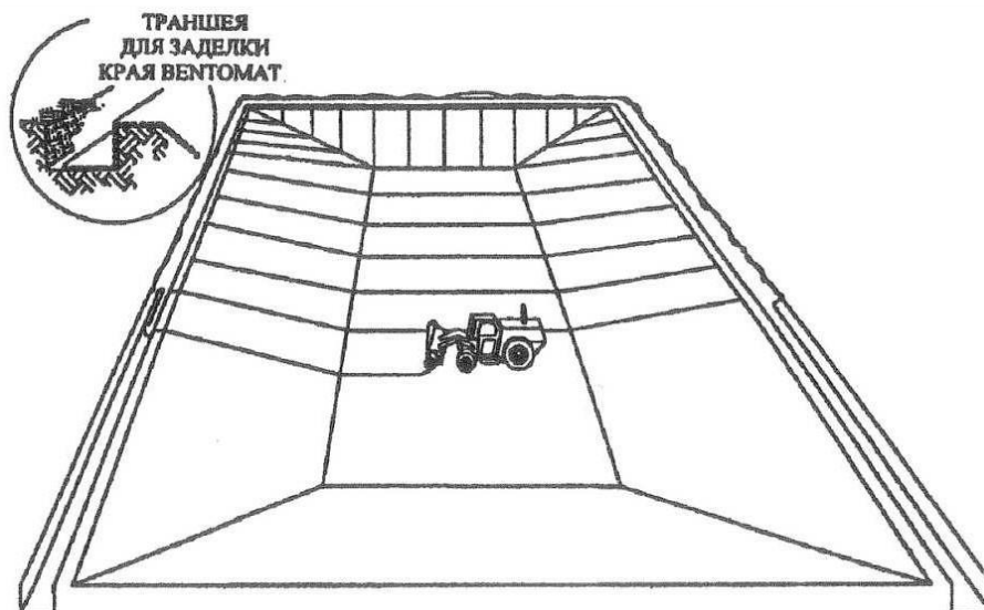
Рисунок 4.4.6.1 – Схема укладки бентонитовых матов
