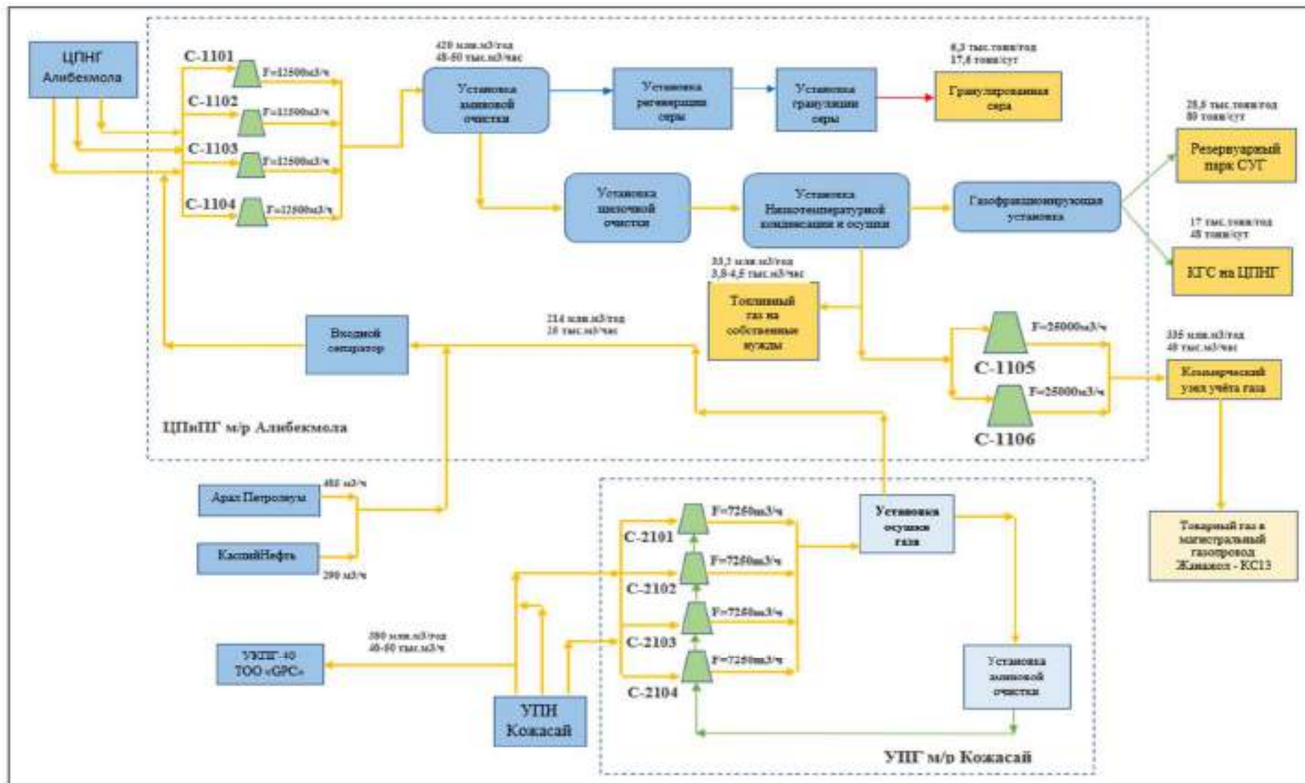
Рисунок 4 – Блок-схема ЦППГ м/р Алибекмола и УПГ м/р Кожасай
