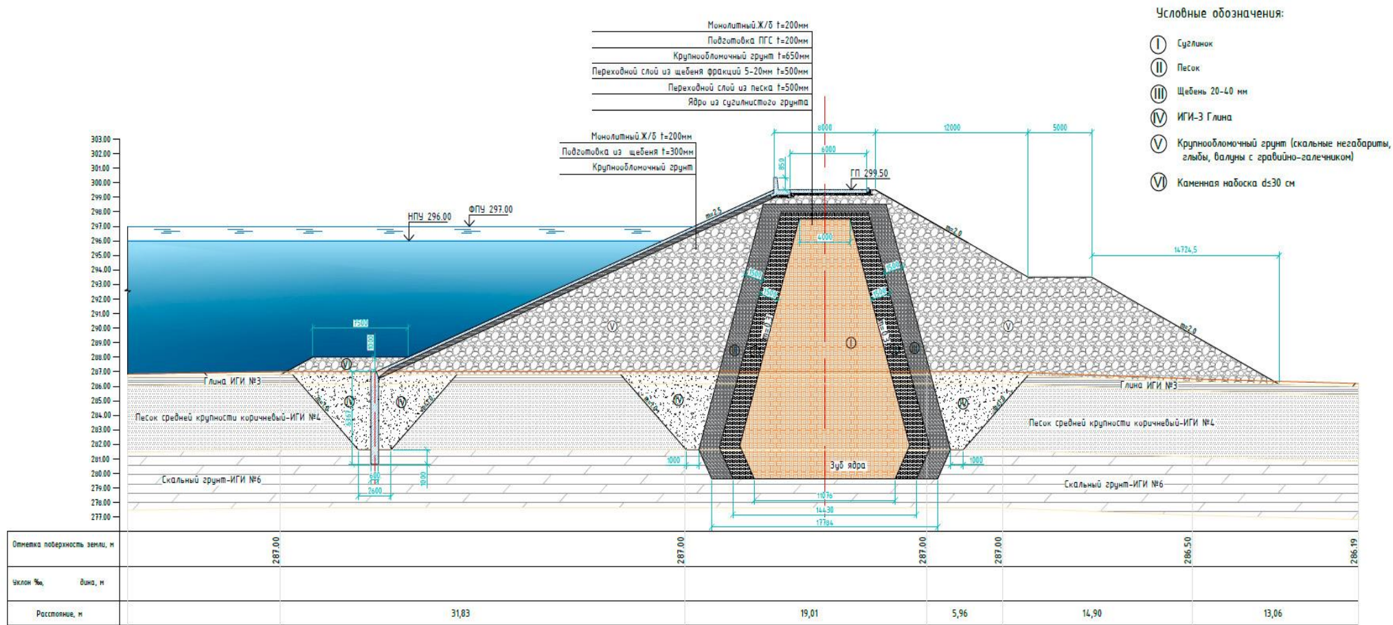
Поперечное сечение плотины на ПК 4+50,00
