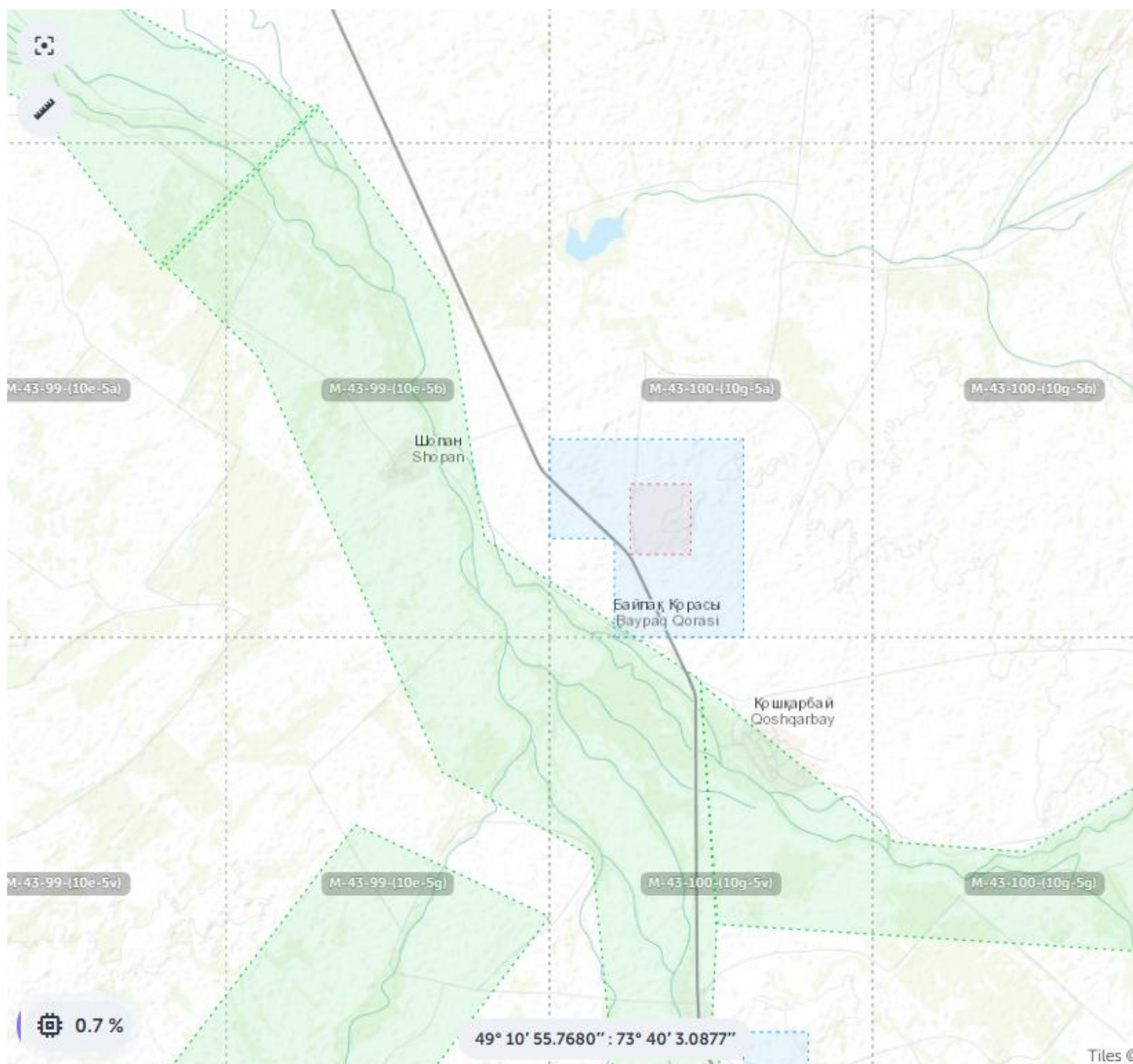
Рисунок 1.6. Гидрографическая сеть
