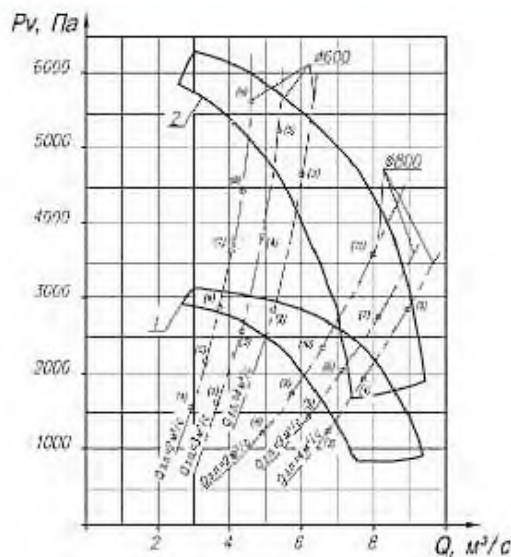
Рис. 4. Аэродинамическая характеристика вентилятора ВМЗ-6.
