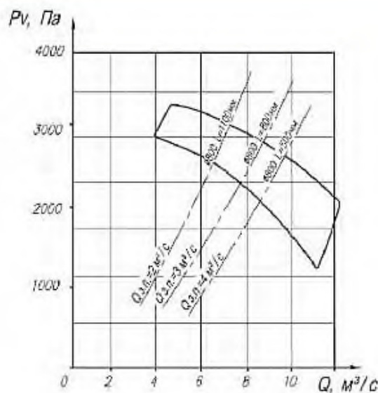
Рис. 5. Аэродинамическая характеристика вентилятора ВМЗ-8.
