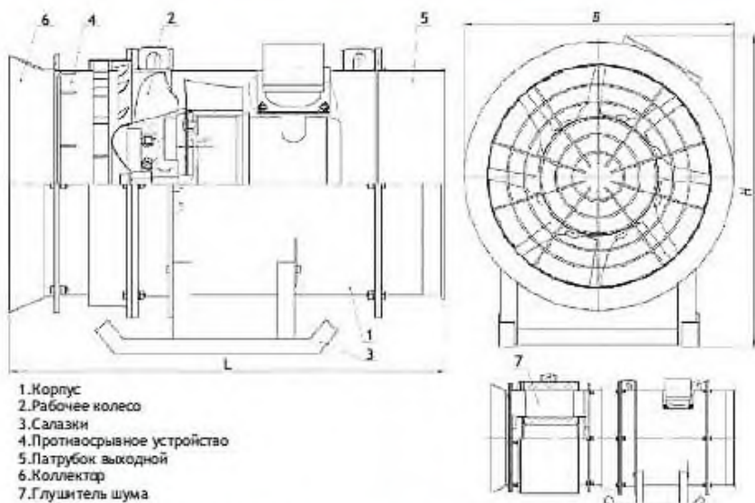
Рис. 1. Габаритные и присоединительные размеры вентиляторов шахтных местного проветривания ВМЗ.
