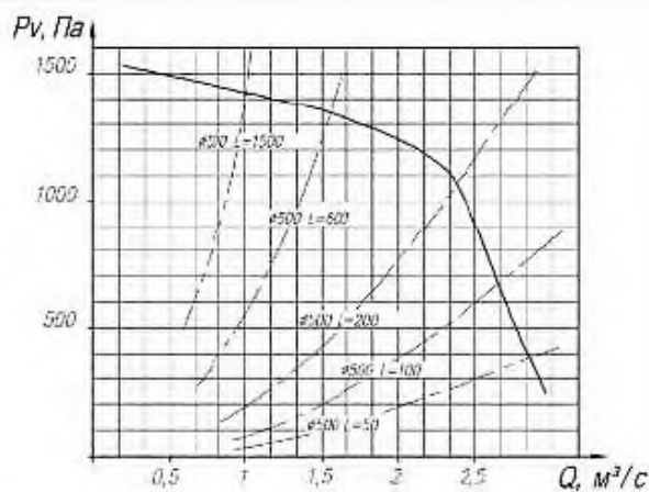
Рис. 2. Аэродинамическая характеристика вентилятора ВМЗ-4.
