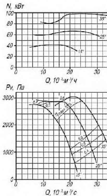
Рис. 6. Аэродинамическая характеристика вентилятора ВМЗ-12.
