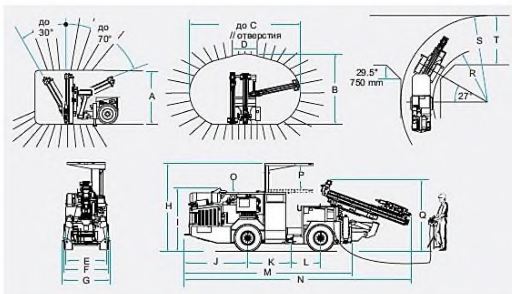
Габариты при бурении
