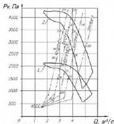
Рис. 3. Аэродинамическая характеристика вентилятора ВМЗ-5.
