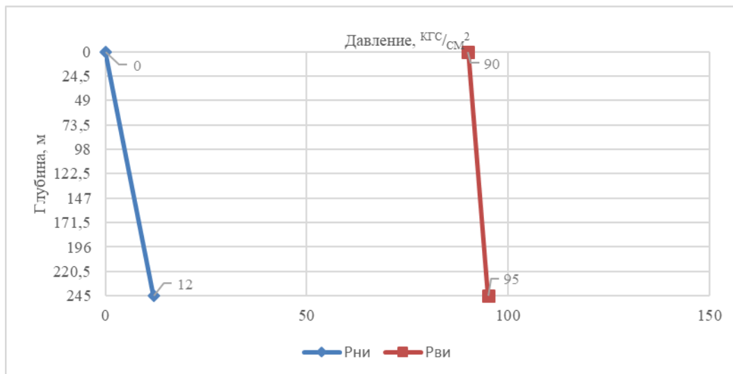
Рисунок 9.1– Эпюра избыточных наружных и внутренних давлений, действующих по длине на кондуктор Ø 244,5 мм (9 5/8")
