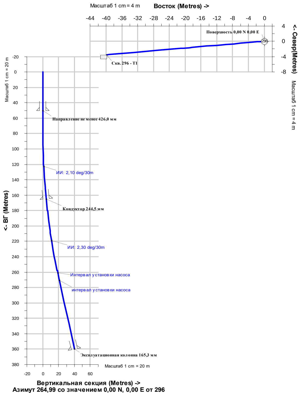
Рисунок 6.1 - Профиль вертикальной и горизонтальной проекции траектории наклонно - направленного ствола скважины
