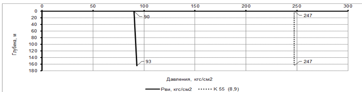
Рисунок 9.1– Эпюры избыточных наружных и внутренних давлений, действующих по длине на кондуктор Ø 244,5 мм
