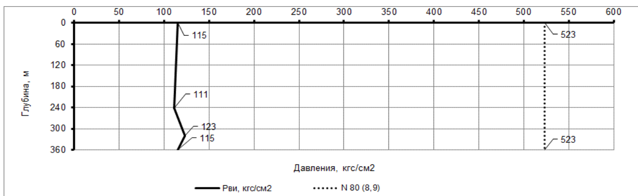
Рисунок 9.2– Эпюры избыточных наружных и внутренних давлений, действующих по длине на эксплуатационную колонну Ø 168,3 мм
