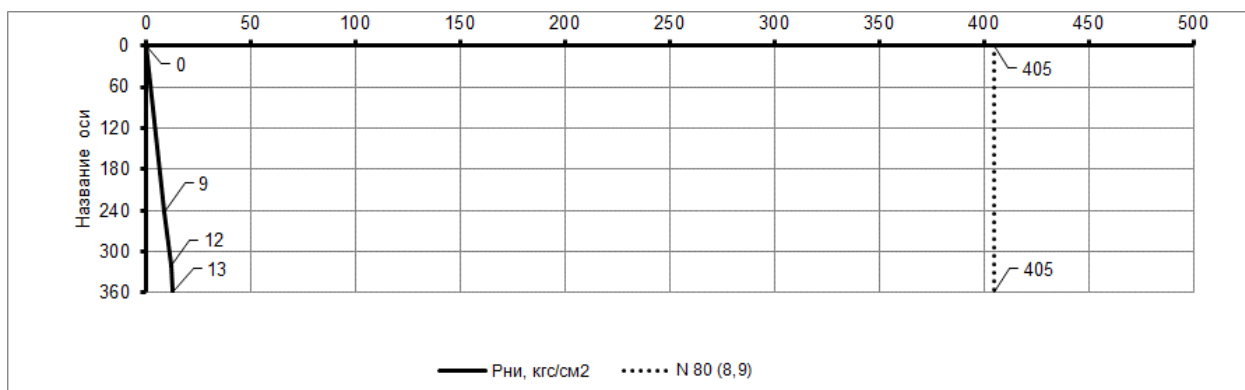
Рисунок 9.1– Эпюры избыточных наружных и внутренних давлений, действующих по длине на кондуктор Ø 244,5 мм
