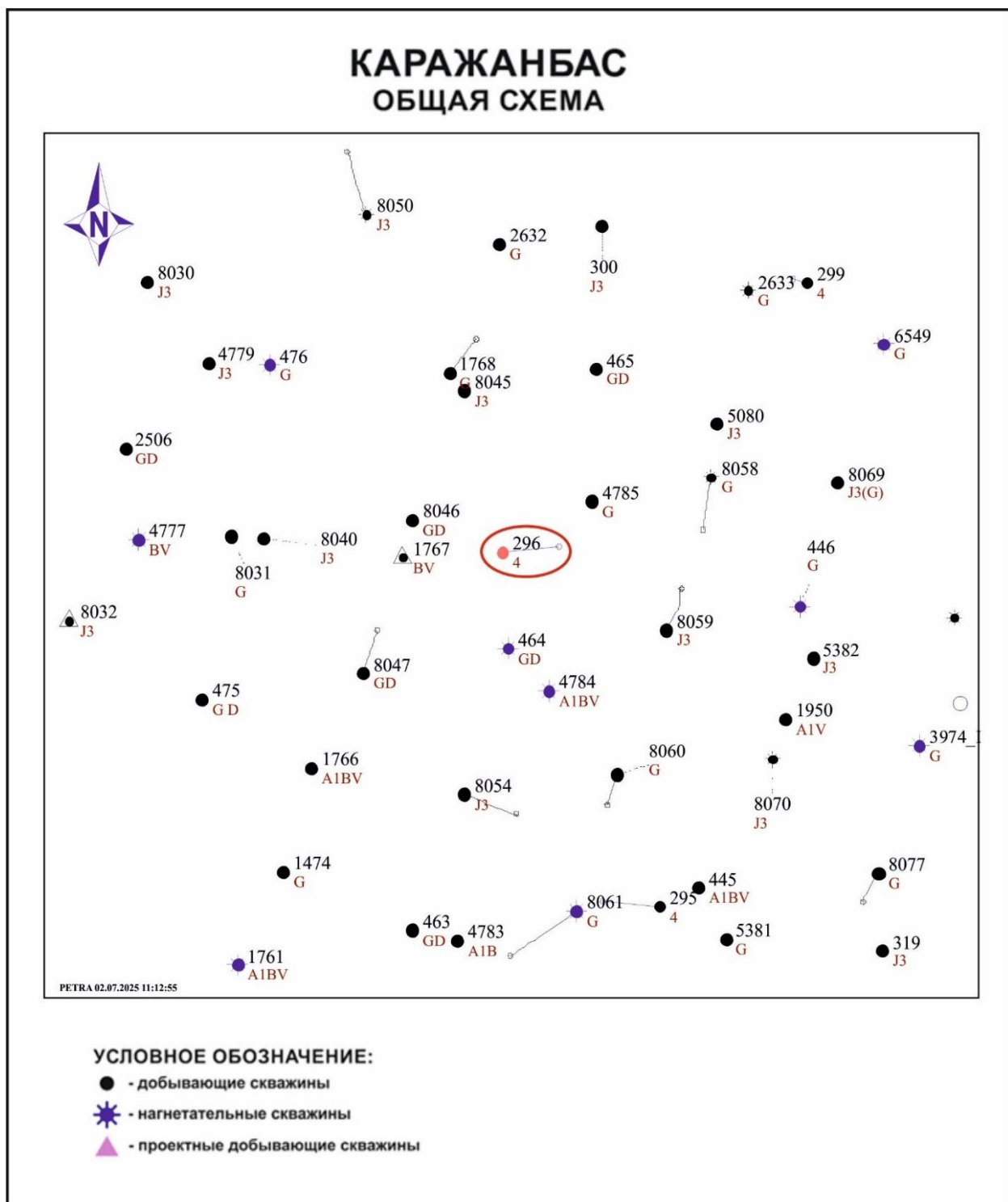
Рисунок 4.2 – Месторасположение проектной скважины №296
