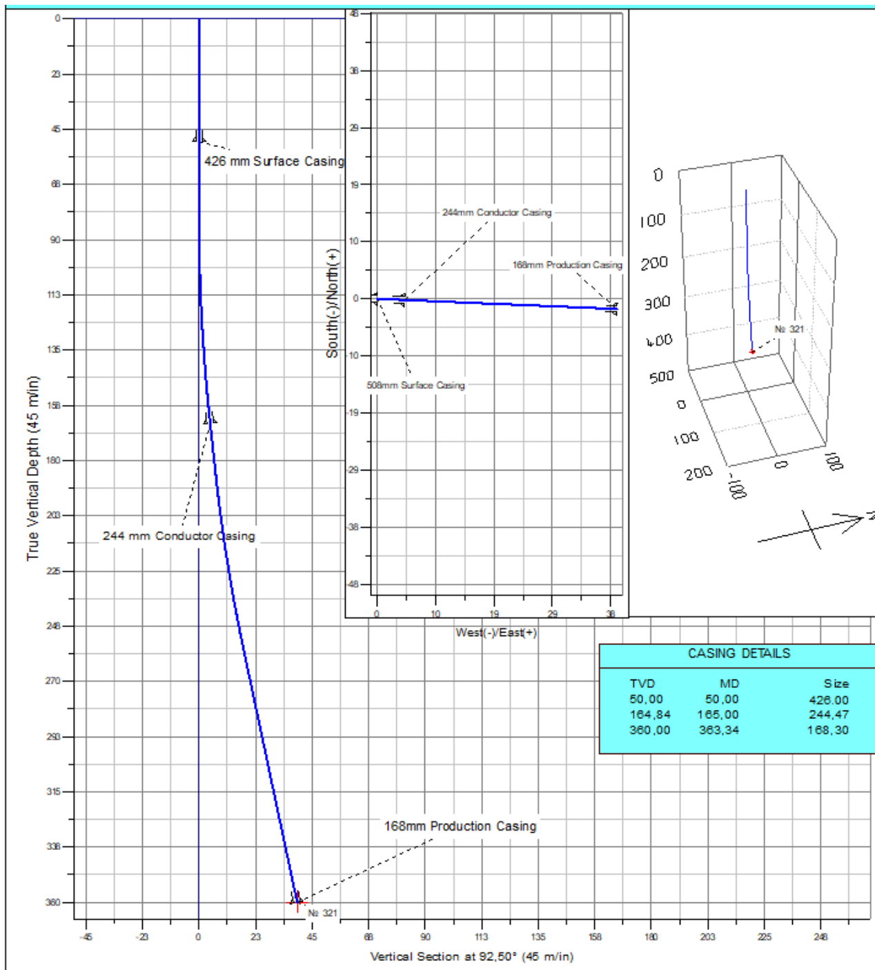
Рисунок 6.1 - Профиль вертикальной и горизонтальной проекции траектории наклонно - направленного ствола скважины
