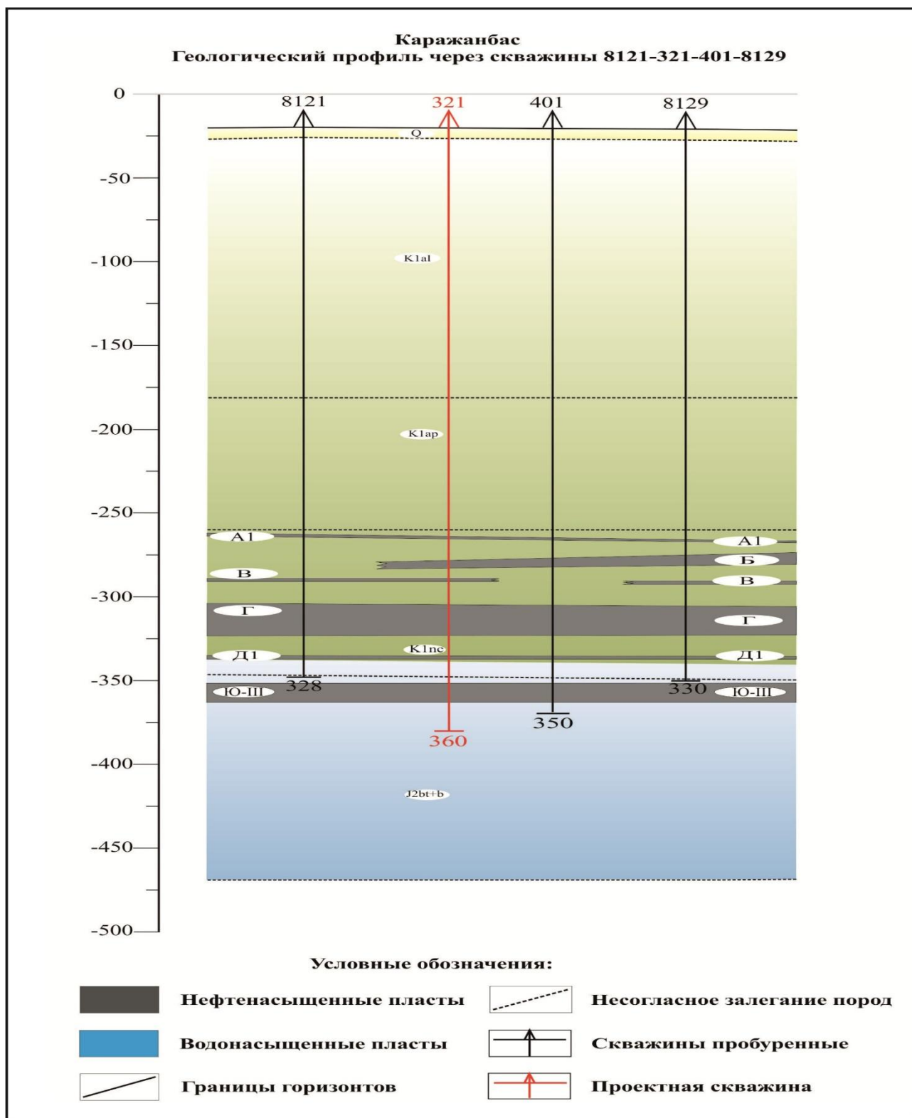
Рисунок 4.3 – Геологический профиль через скважины 8121-321-401-8129.
