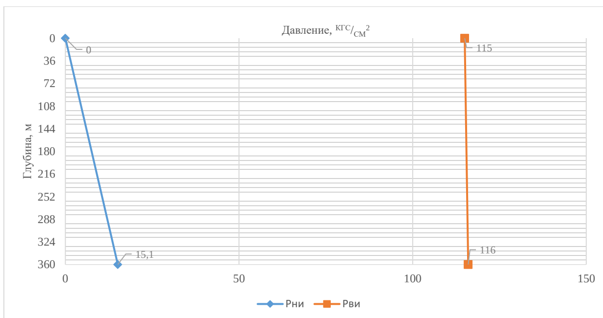
Рисунок 9.2– Эпюра избыточных наружных и внутренних давлений, действующих по длине на эксплуатационную колонну Ø 168,3 мм (6 5/8")
