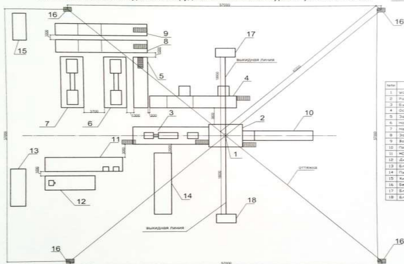
Схема расположения бурового оборудования мобильной буровой установки XJ 550
