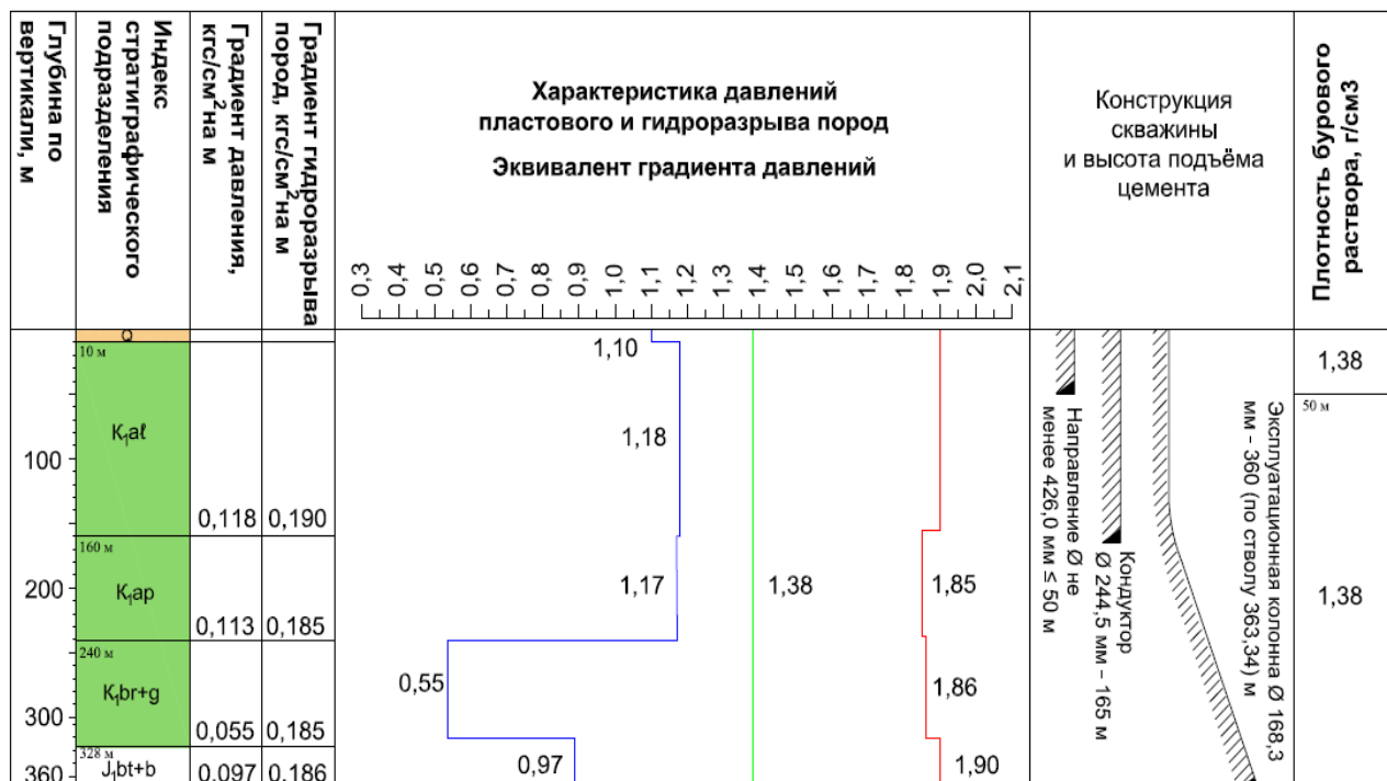
Рисунок 5.1 – График совмещенных давлений
