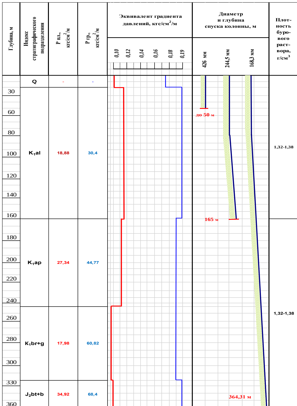
Рисунок 5.1 – График совмещенных давлений
