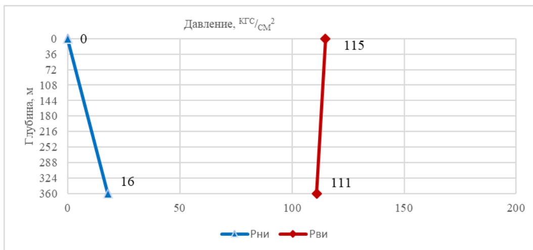
Рисунок 9.2– Эпюра избыточных наружных и внутренних давлений, действующих по длине на эксплуатационную колонну Ø 168,3 мм
