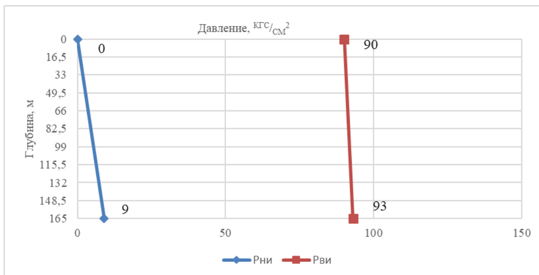
Рисунок 9.1– Эпюра избыточных наружных и внутренних давлений, действующих по длине на кондуктор Ø 244,5 мм
