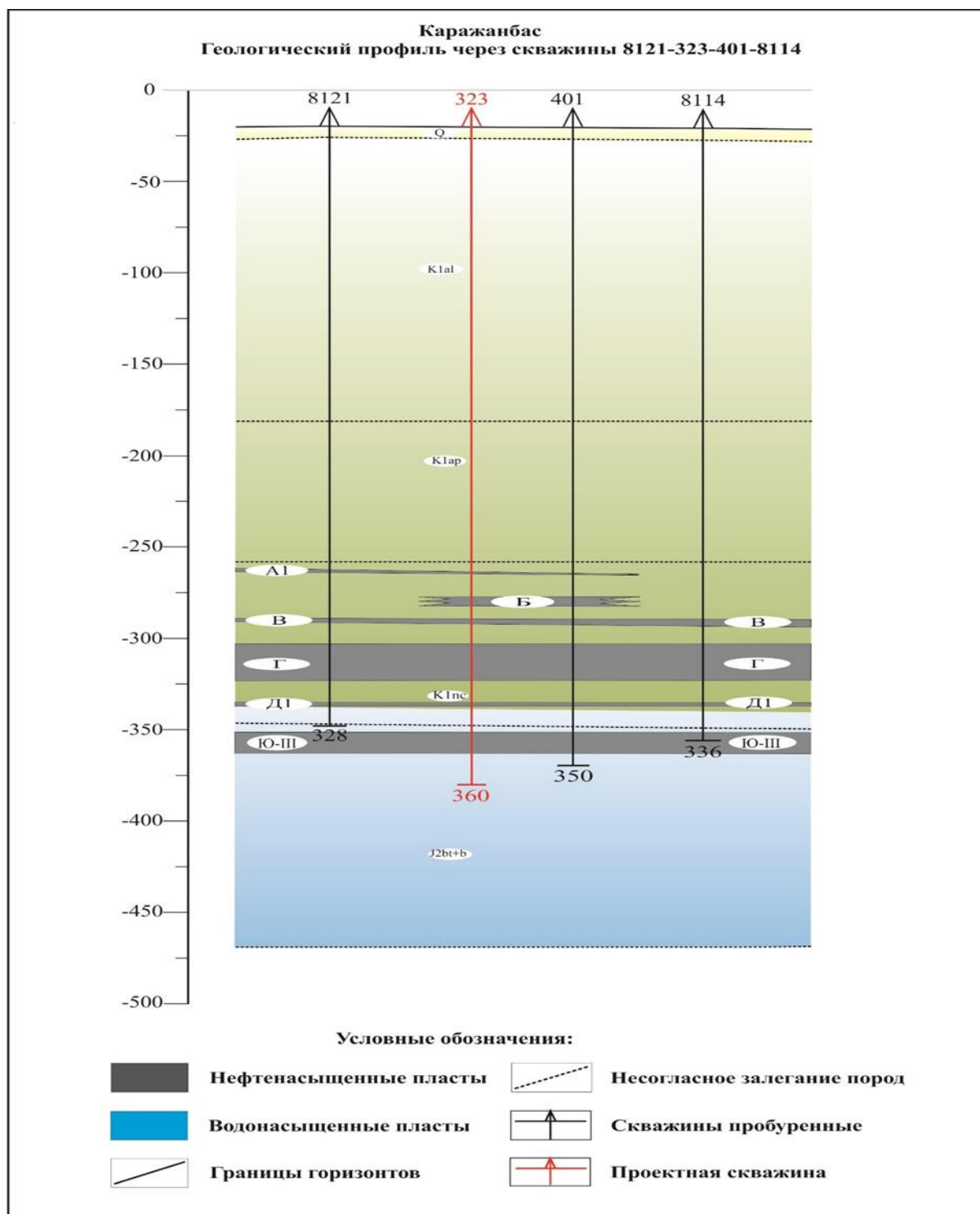
Рисунок 4.3 - Профильный геологический разрез через скважины 8121-323-401-8114
