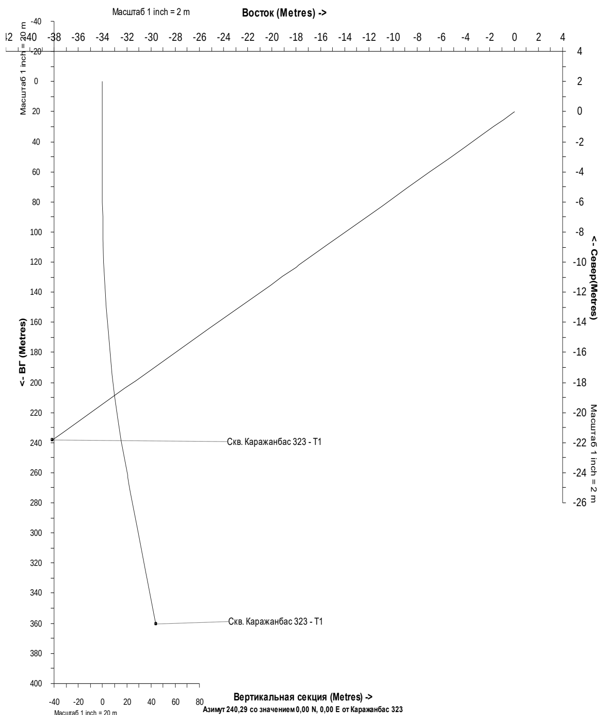
Рисунок 6.1 - Профиль вертикальной и горизонтальной проекции траектории наклонно - направленного ствола скважины
