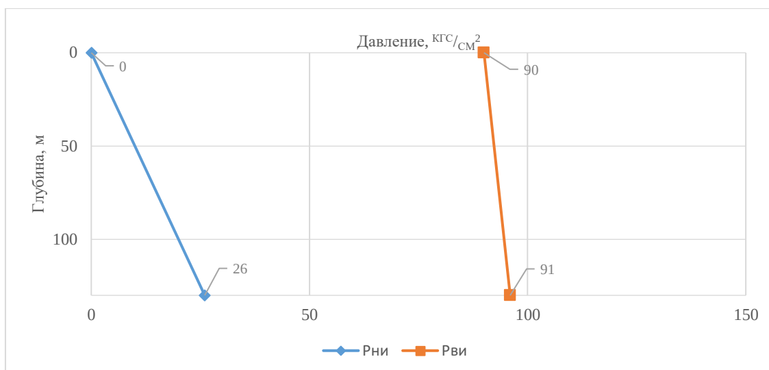
Рисунок 9.1 – Распределение избыточных внутренних и наружных давлений по длине колонны Ø 244,5 мм
