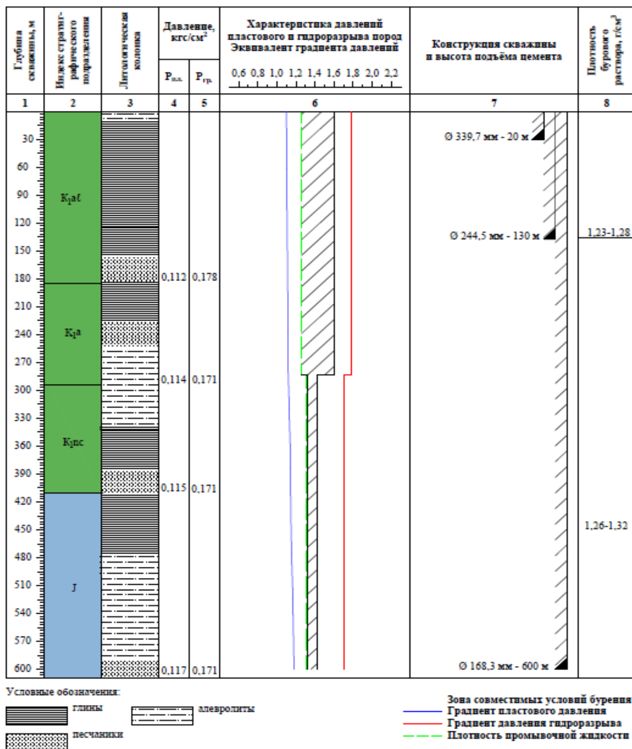
Рисунок 5.1 – График совмещенных давлений
