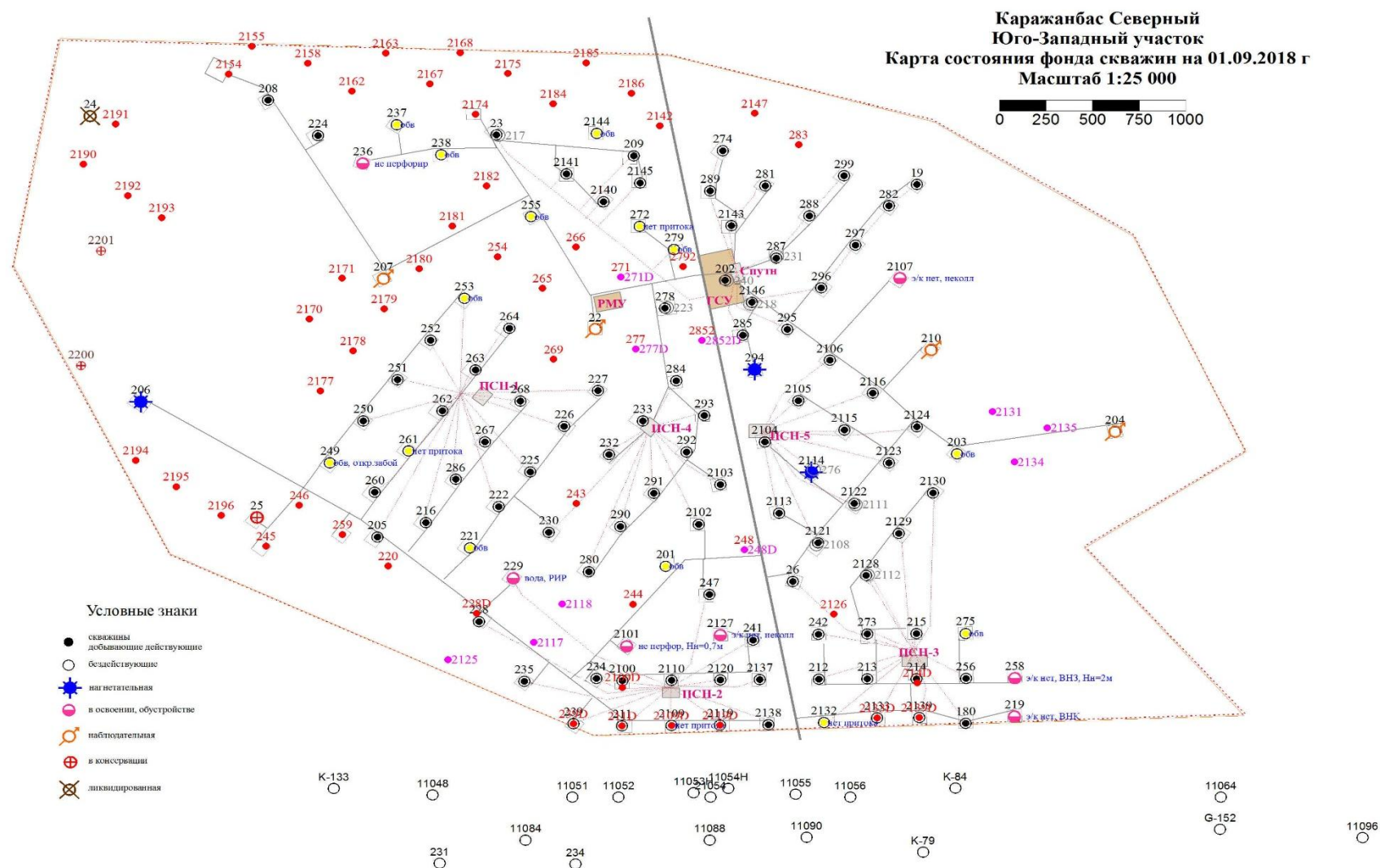
Рисунок 4.2 – Расположения пробуренных и проектная скважин
