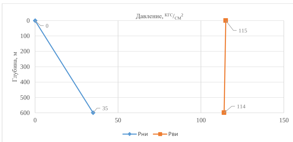
Рисунок 9.2 – Распределение избыточных внутренних и наружных давлений по длине колонны Ø 168,3 мм (эксплуатационная колонна)
