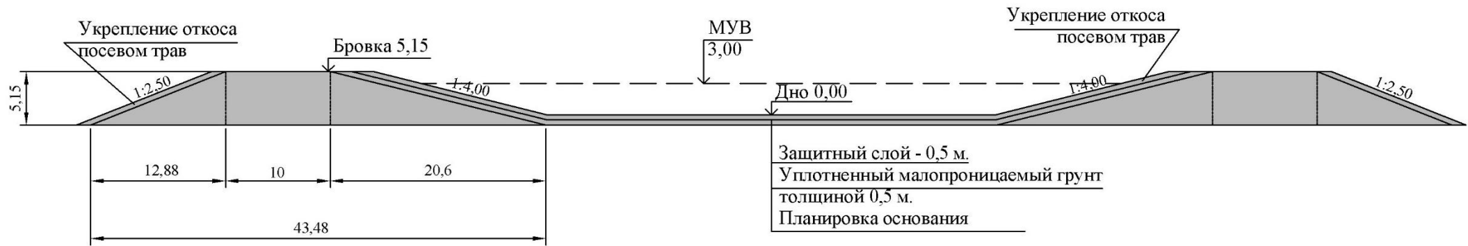
Рис. 6.1. Конструкция противофильтрационного экрана пруда-накопителя карьерных вод. Масштаб 1: 500
