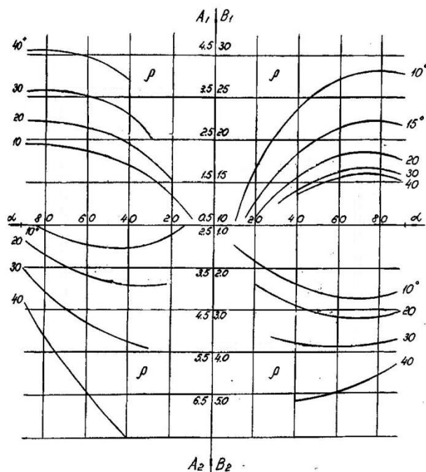
Рисунок 3.4— Номограмма для определения коэффициентов K_1 , H_1 , a , b
