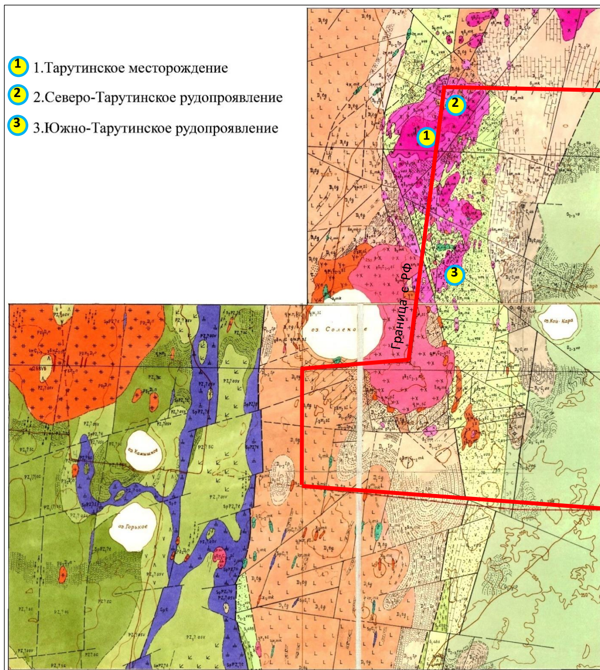
Рисунок 2.2 – Геологическая карта (фрагмент) палеозойского фундамента
