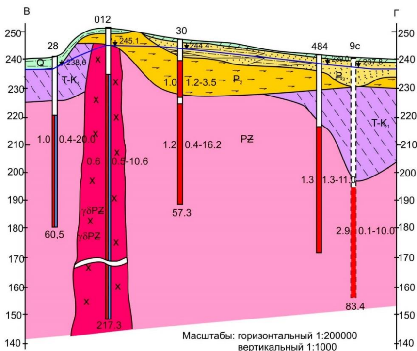
Рисунок 2.6–Гидрогеологический разрез по линии В-Г
