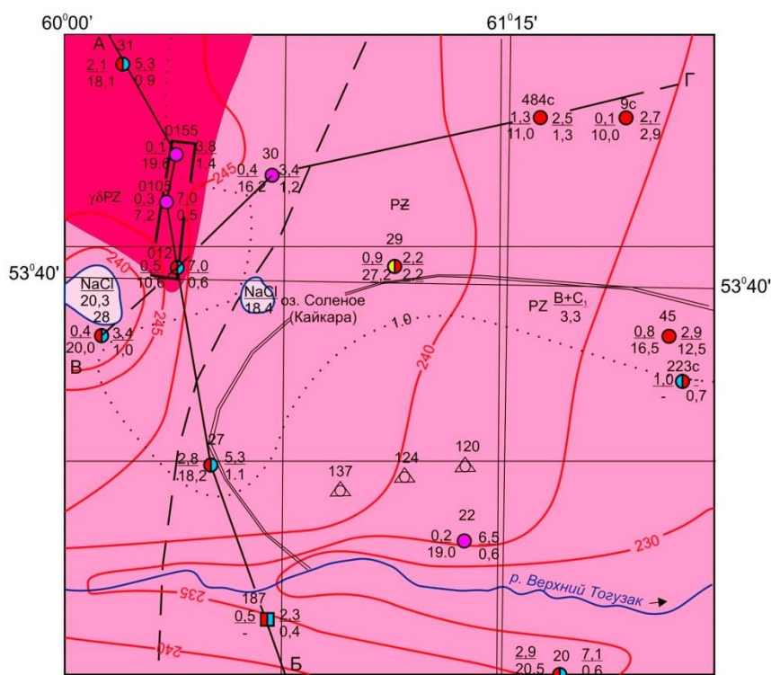
Рисунок 2.7 – Схематическая гидрогеологическая карта палеозойского водоносного комплекса пород Восточно-Тарутинское медно-золотого рудопроявления
