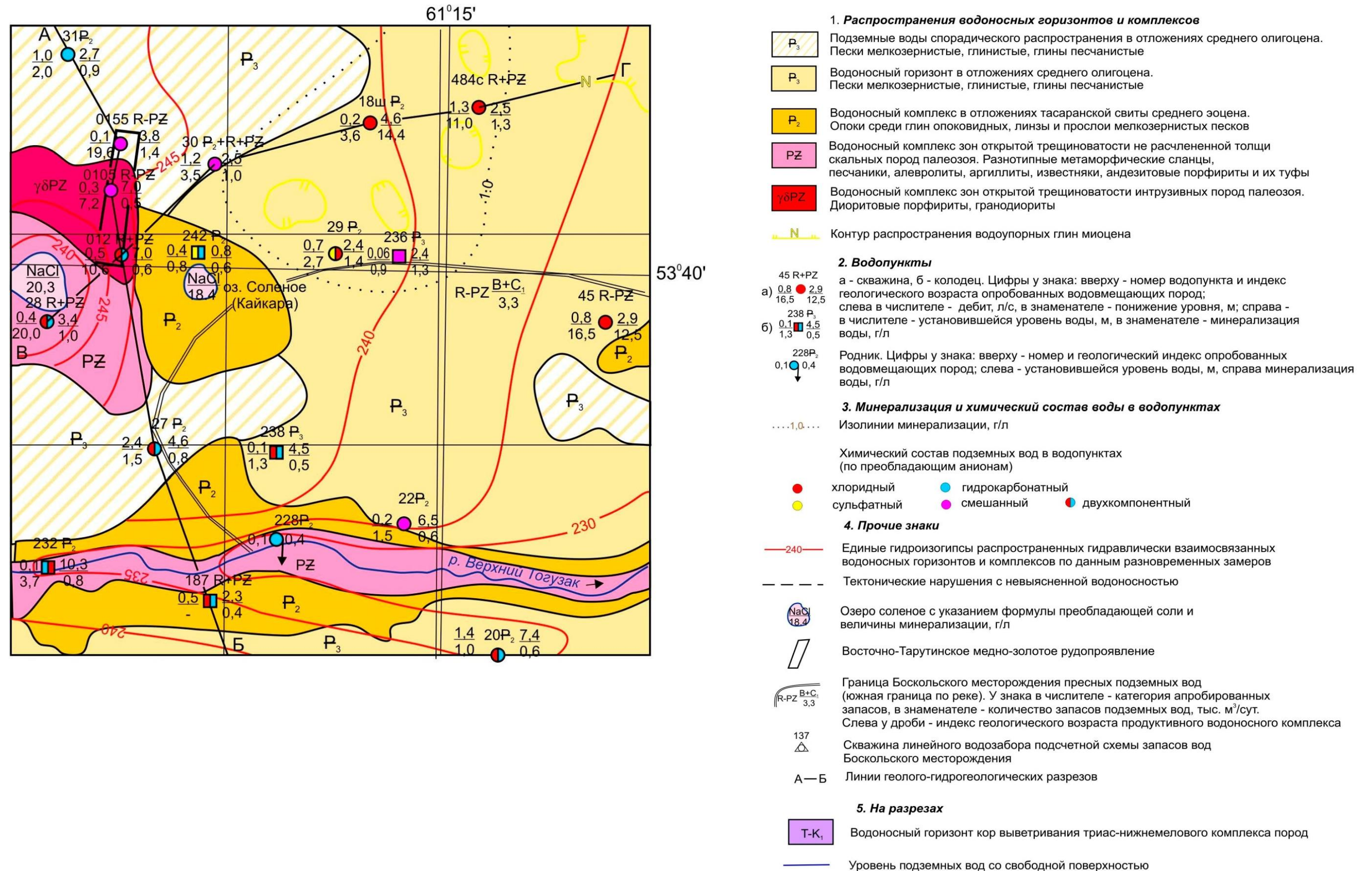
Рисунок 2.4 – Гидрогеологическая карта района Восточно-Тарутинскоемедно-золотого рудопроявления
