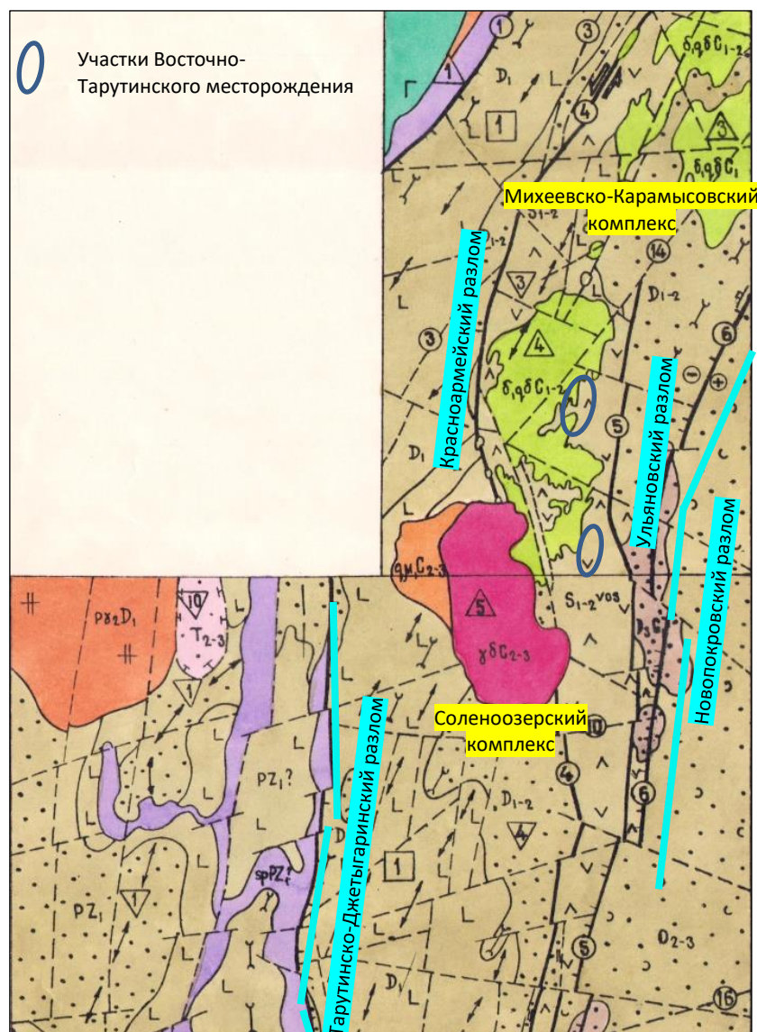
Рисунок 2.1 – Структурно-формационная схема района месторождения
