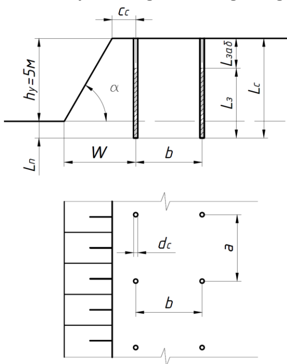
Рисунок 3.6 – Схема расположения технологических скважин в массиве горных пород
