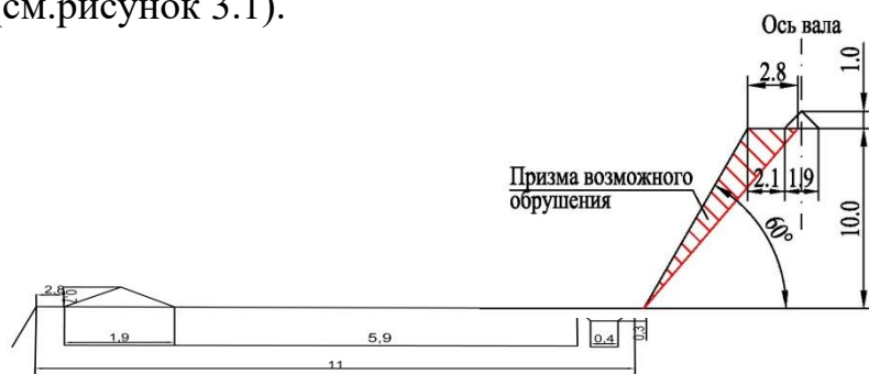
Рисунок 3.1 – Призма возможного обрушения и Схема к определению ширины транспортной бермы
