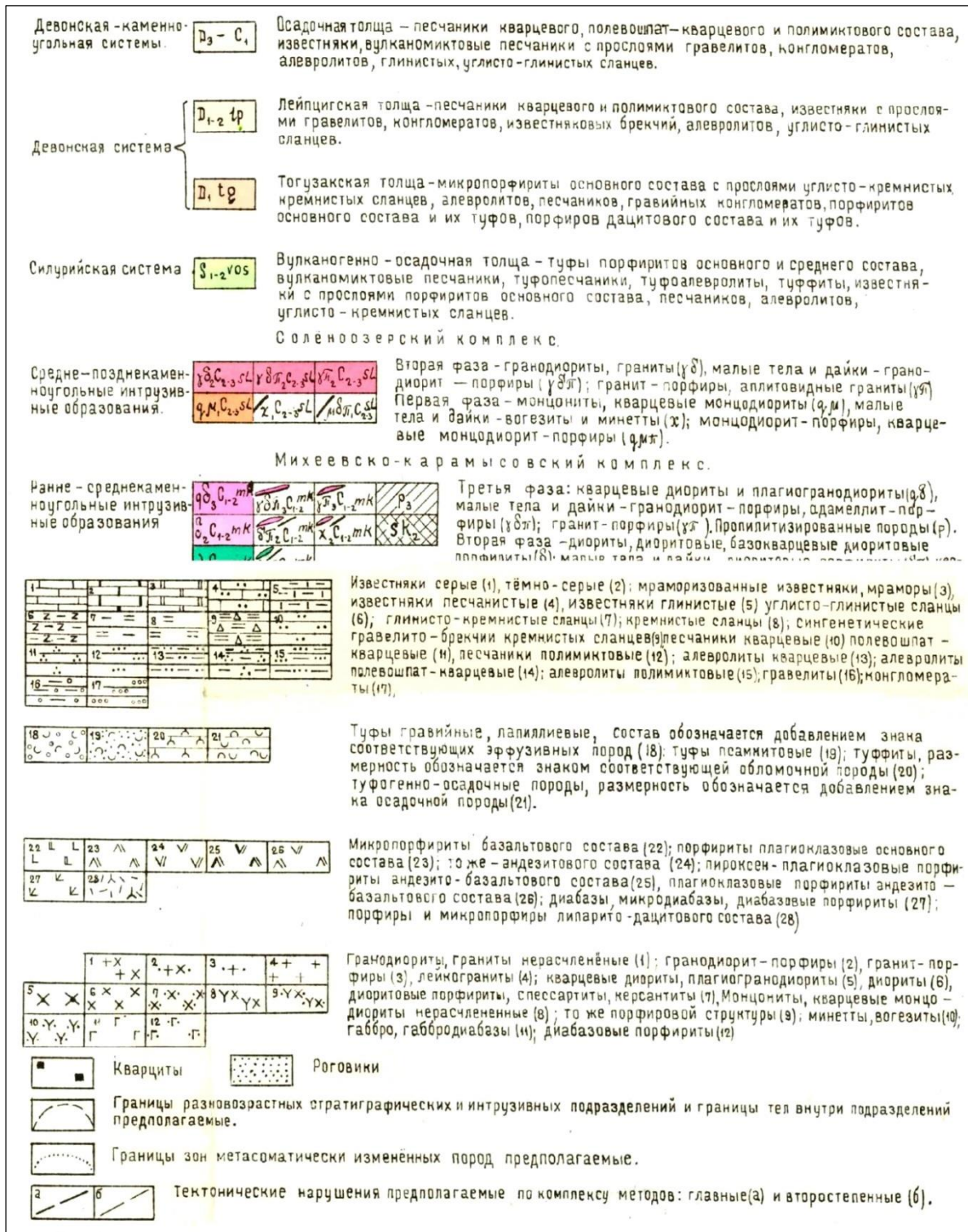
Рисунок 2.3 – Условные обозначения к геологической карте
