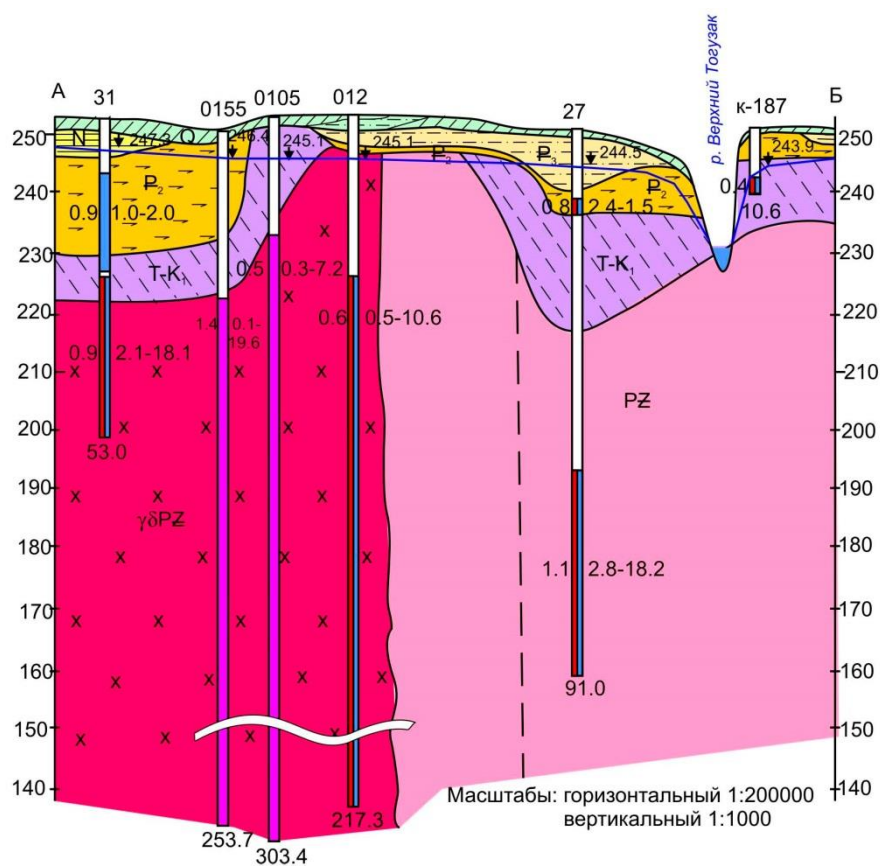
Рисунок 2.5—Гидрогеологический разрез по линии А-Б
