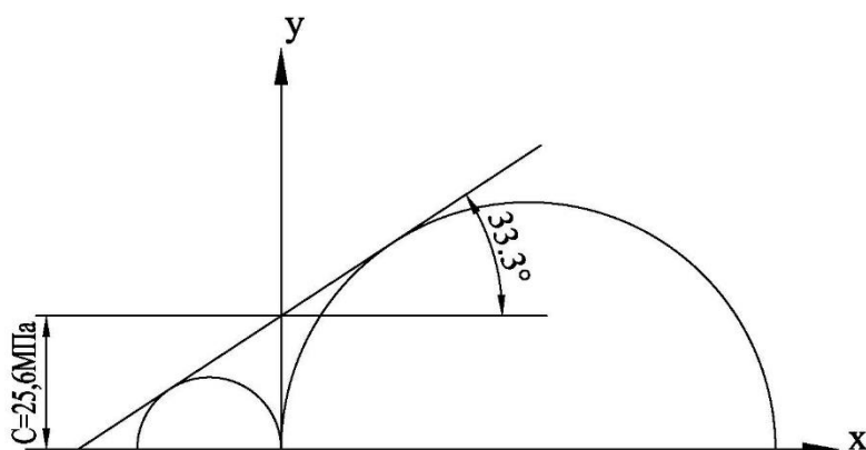
Рисунок 3.2 – Паспорт прочности для средневзвешанных значений физико-механических свойств скальных пород
