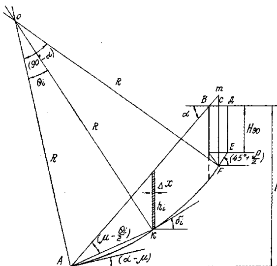
Рисунок 3.5– Схема к расчету устойчивости откоса аналитическим способом с использованием круглоцилиндрической поверхности скольжения
