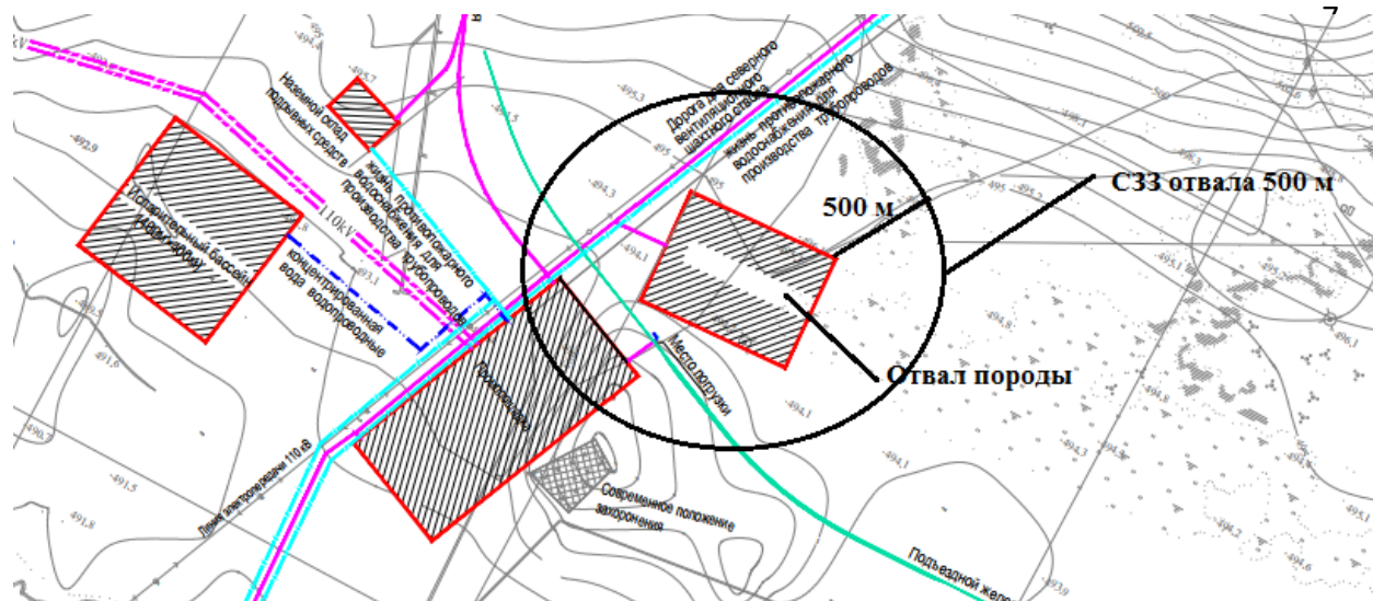
Рисунок 2. Расположение объектов поверхностной инфраструктуры с указанием границы СЗЗ
