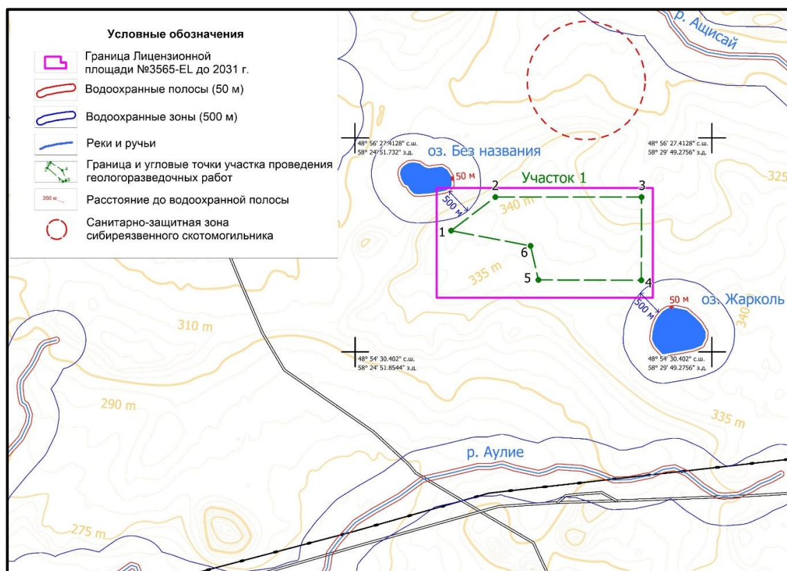
Рисунок 7.1 Схема расположения участка проведения ГРП относительно поверхностных водных источников
