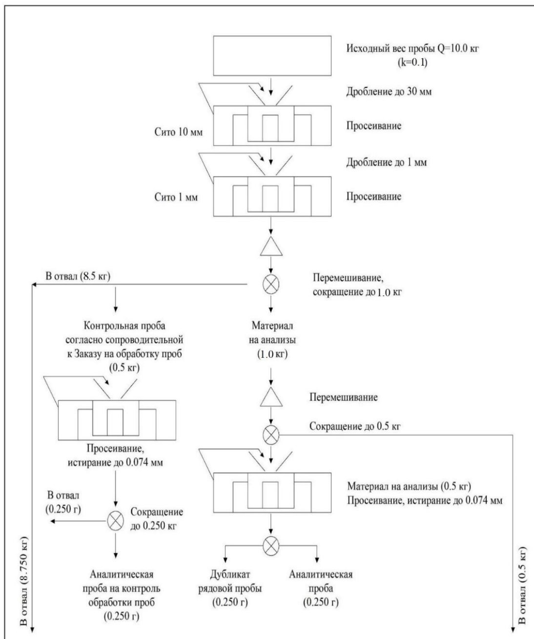
Рисунок 5.4 Схема обработки бороздовых проб
