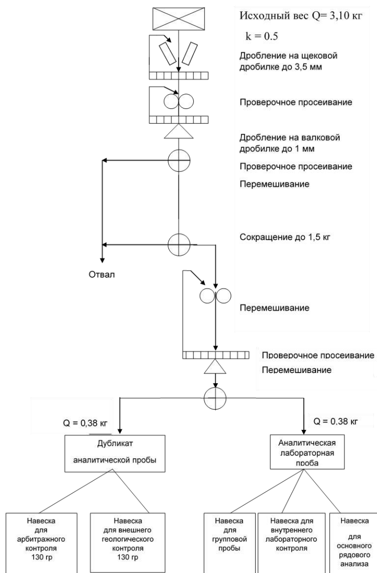
Рис. 4.5 - Схема обработки керновых проб
