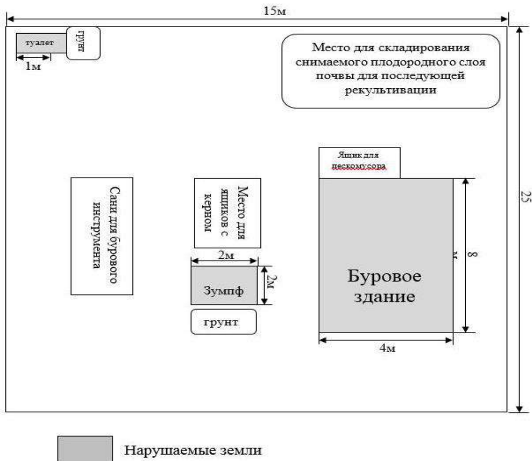
Рис.4.2 - Схема размещения бурового оборудования на площадке
