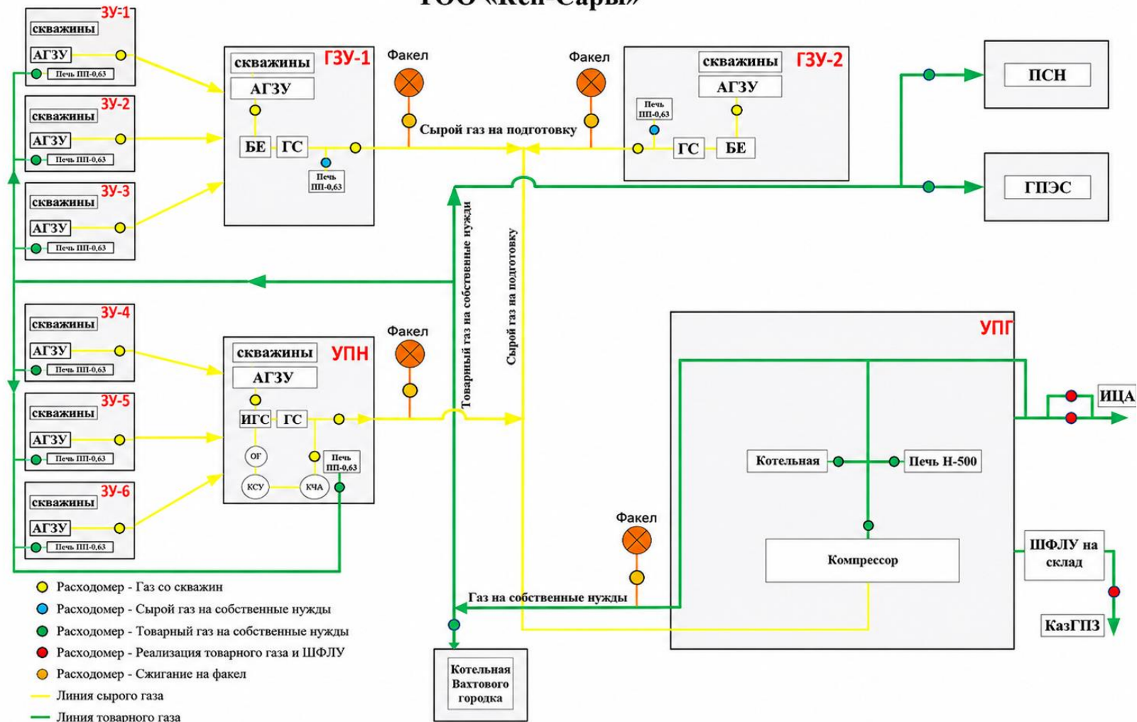
Рисунок – Принципиальная схема системы промышленного сбора продукции скважин месторождения Арыстановское
