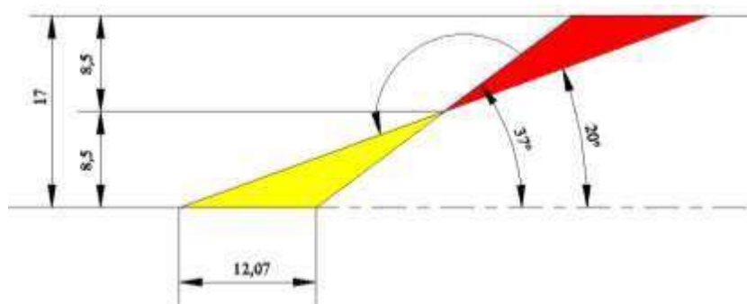
Рис. 21. Схема выполаживания отвала вскрышных пород
