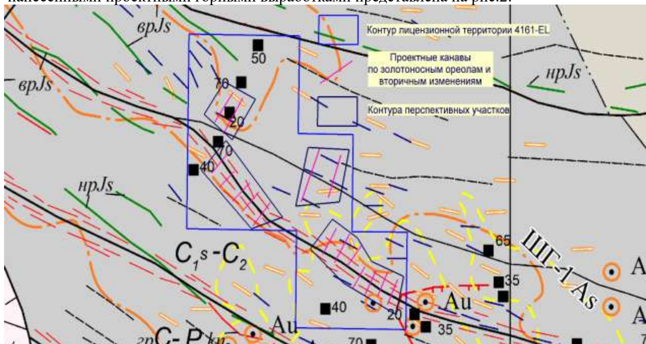
Рис.2 Схематическая карта расположения вторичных ореолов и полезных ископаемых с нанесёнными проектными горными выработками
