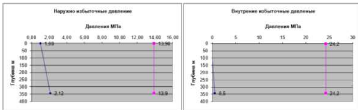
Рисунок 9.1-Распределение избыточных давлений (кондуктор)
