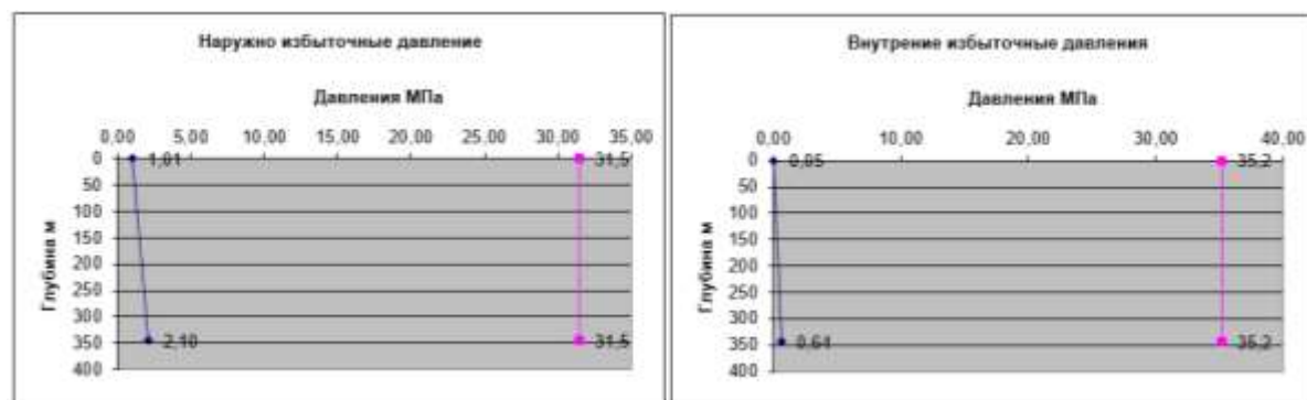
Рисунок 9.2-Распределение избыточных давлений (эксплуатационная колонна)
