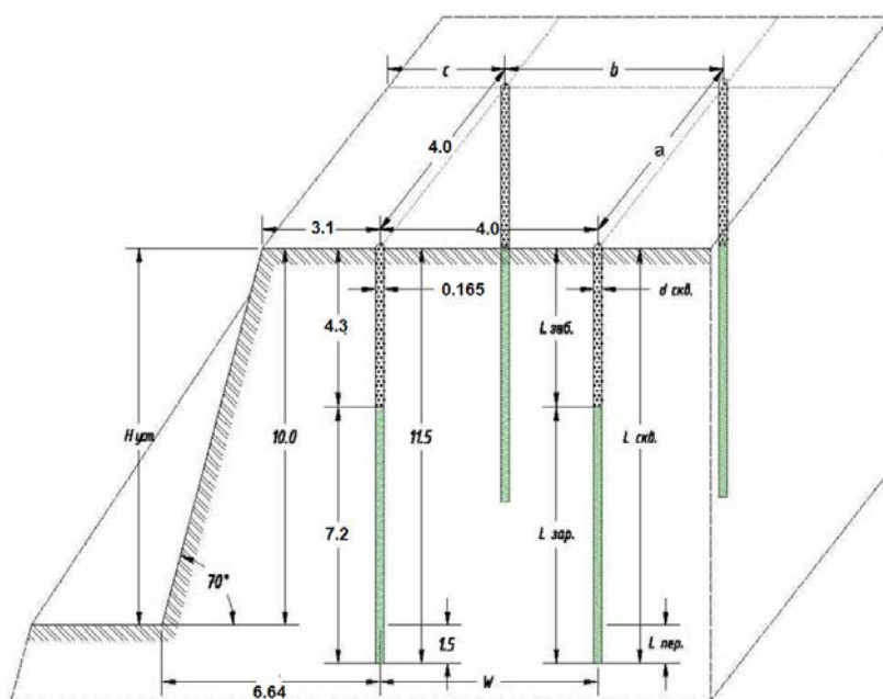
Рисунок 3.16.3.1 - Параметры конструкции скважинного заряда на вскрыше
