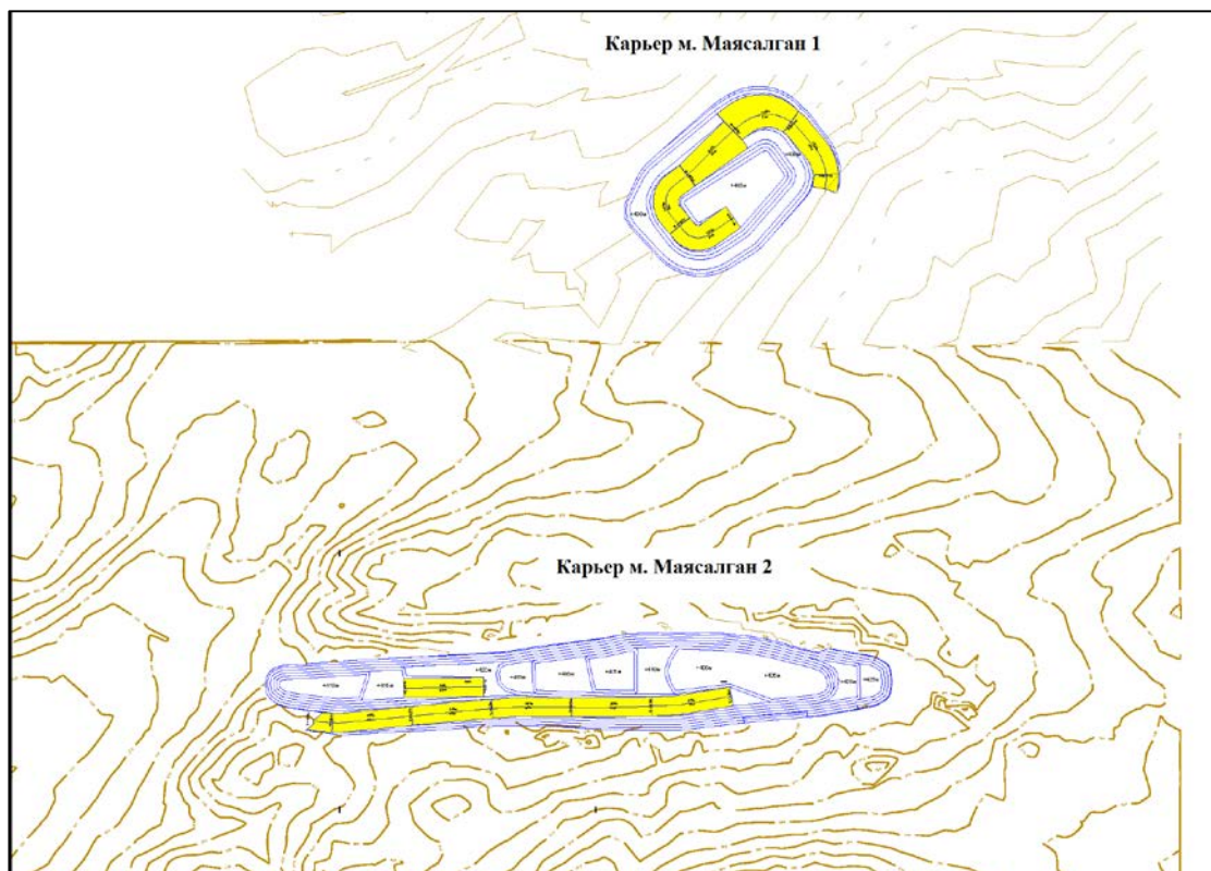
Рисунок 3.8.1 – Карьеры месторождений Маясалган 1 и Маясалган 2 на конец отработки 2031 г. (вид в плане)
