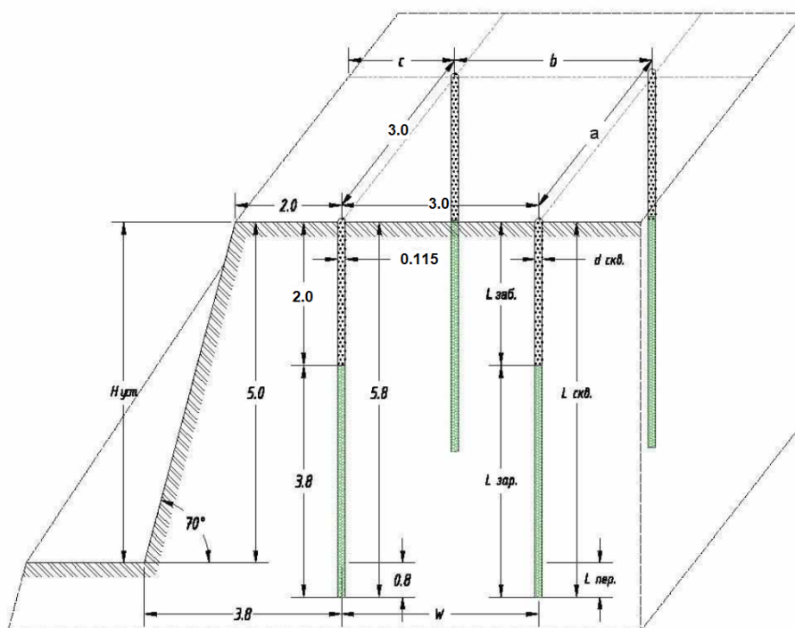
Рисунок 3.16.3.1 - Параметры конструкции скважинного заряда на вскрыше
