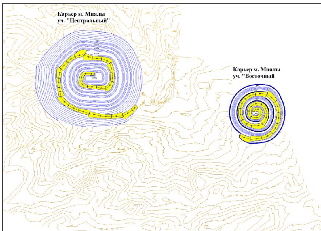
Рисунок 3.8.2 – Карьеры участков «Центральный» и «Восточный» месторождения Миялы на конец отработки 2031 г. (вид в плане)
