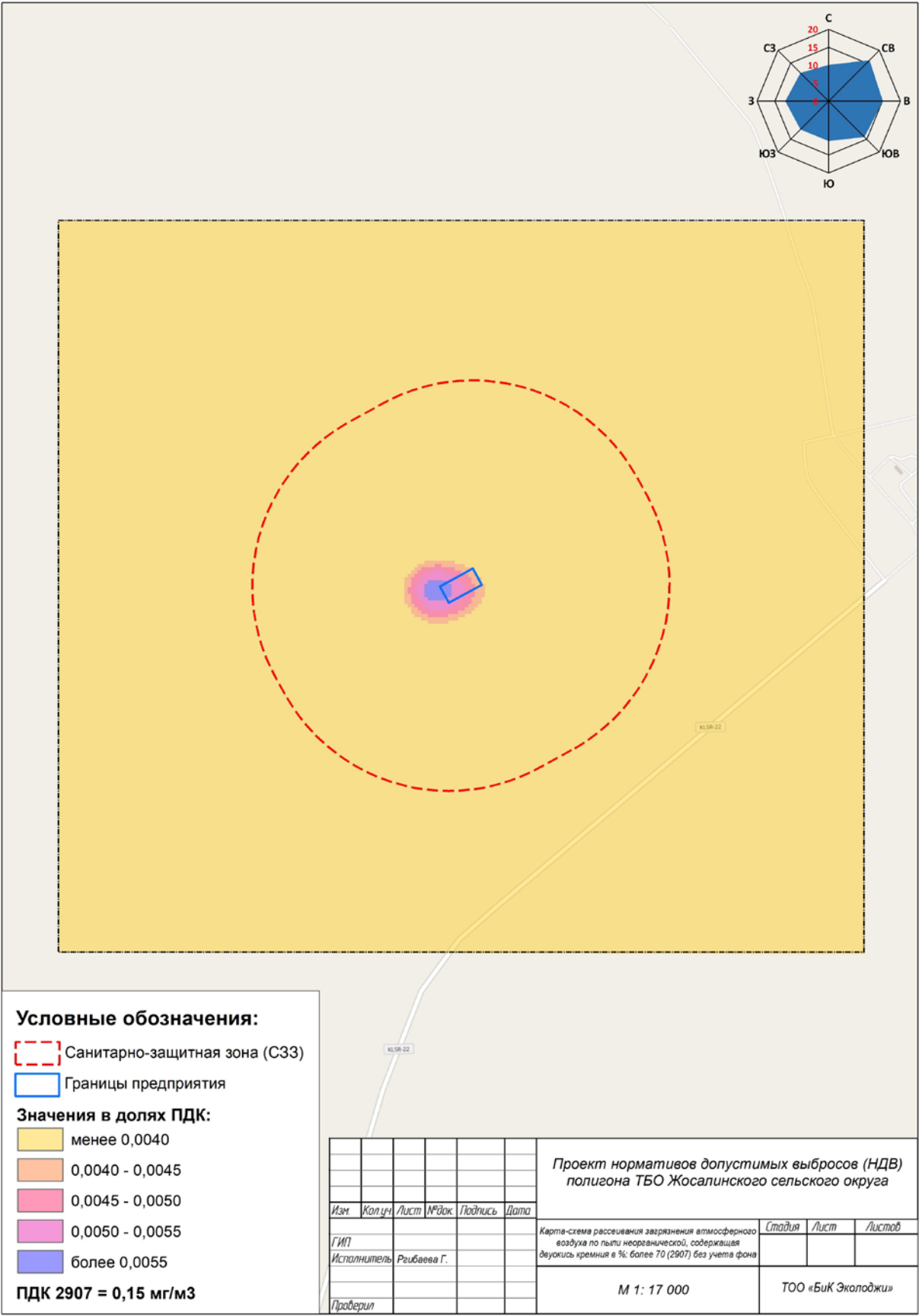
Рисунок 3 Карта-схема рассеивания загрязнения атмосферного воздуха по пыли неорганической, содержащая диоксид кремния в %: более 70 (2907) без учета фона
