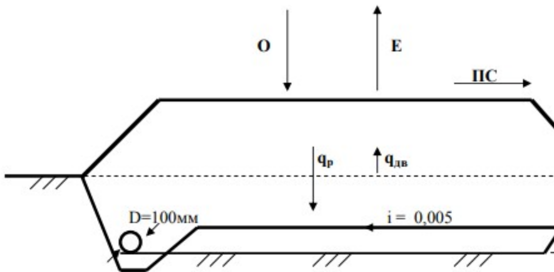
Рис. 4.17. Расчет притока фильтрата к дренаю: О - атмосферные
