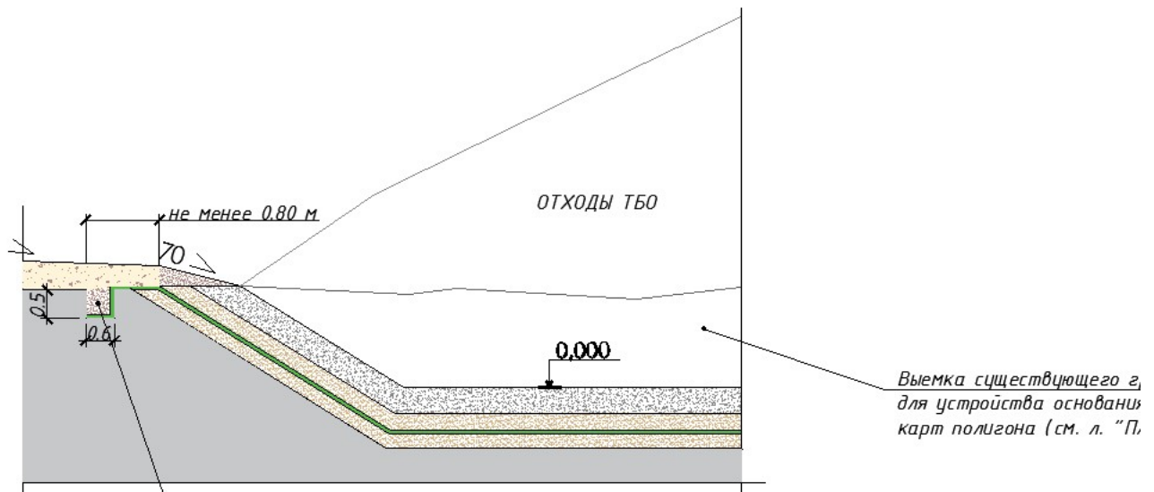
Рисунок 3 – Рекомендуемые размеры траншеи для закрепления материала Укладка материала
