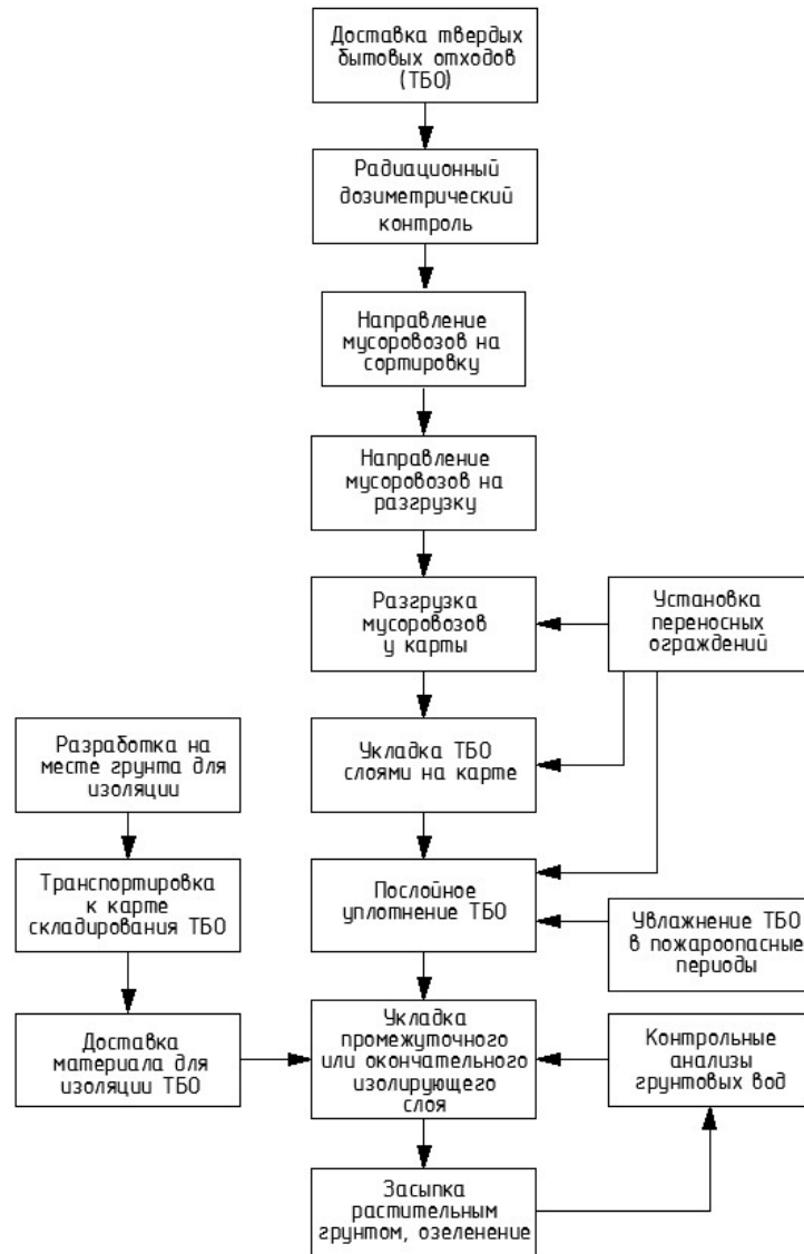
Рисунок 2 - Схема технологии работы полигона ТБО
