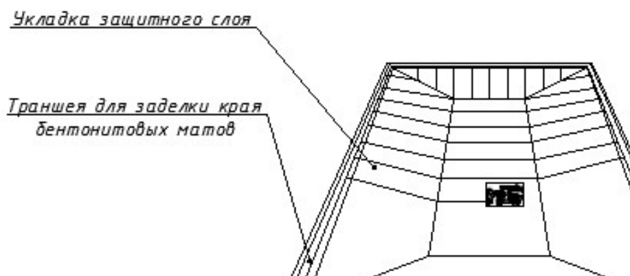
Рисунок 4.1 – Схема укладки бентонитовых матов
