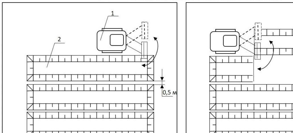
Рисунок 7 – Схема перебуртовки
