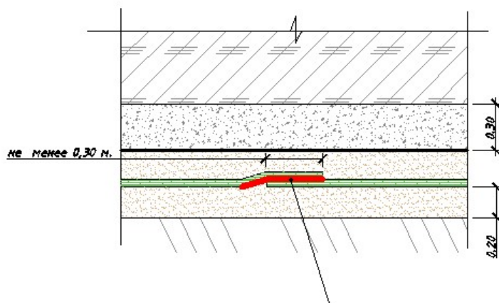
Рисунок 4.2 – Схема нахлеста материала
